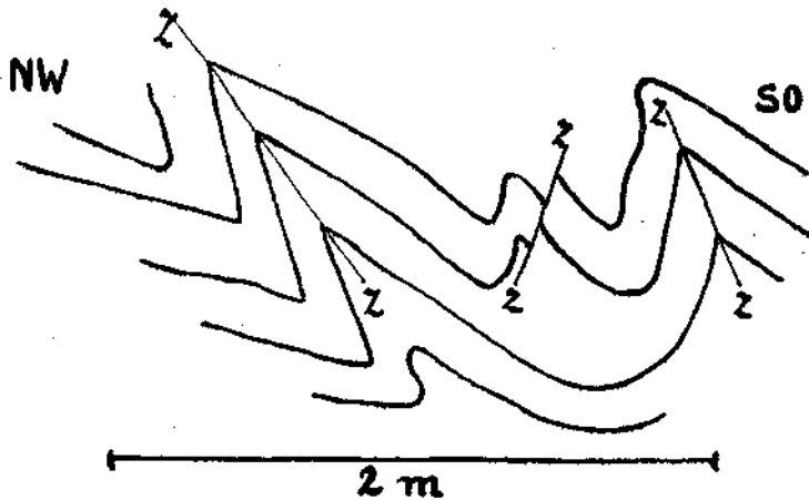
Fig. 6. Faltung von Tonschiefer zwischen Skalar und P. 1011. Z = Zerreiungsflachen.
