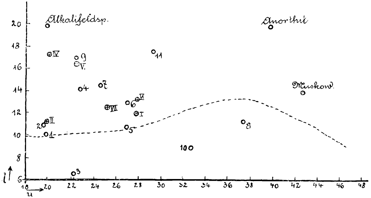
Diagramm nach Becke. (Zum Abschnitt Si-U-L.)
