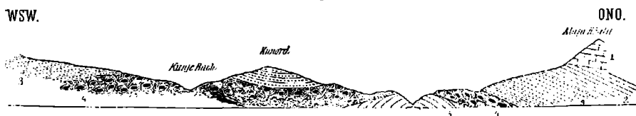
Profil durch die Stammesgebiete von Šala und Kiri.
