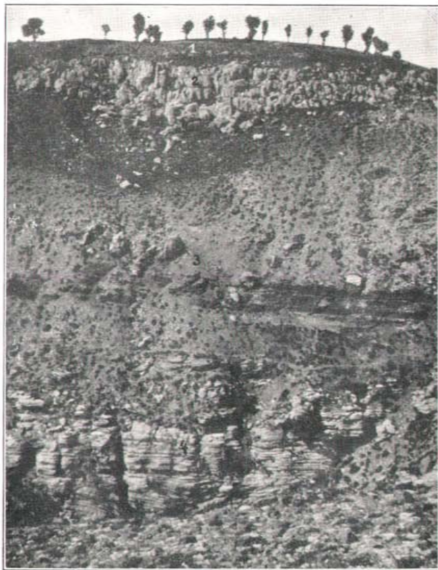
Fig. 1. Juraschichten bei Kroni Madh.
