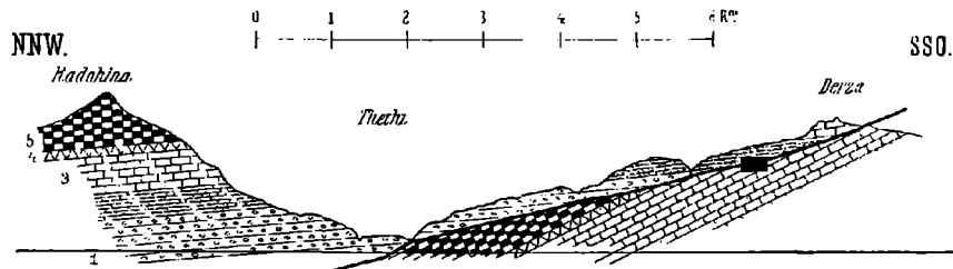
Profil durch das Thethital.
