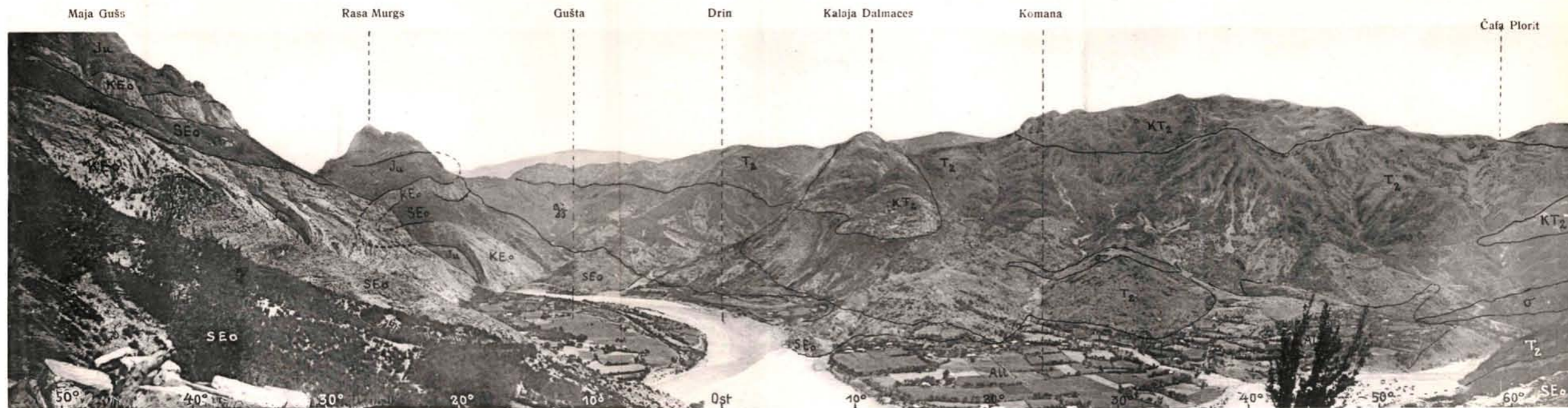
2. Gesamtansicht von Komani, das Versinken der Kukali-Falten unter das Eruptivmassiv von Merdita zeigend.
