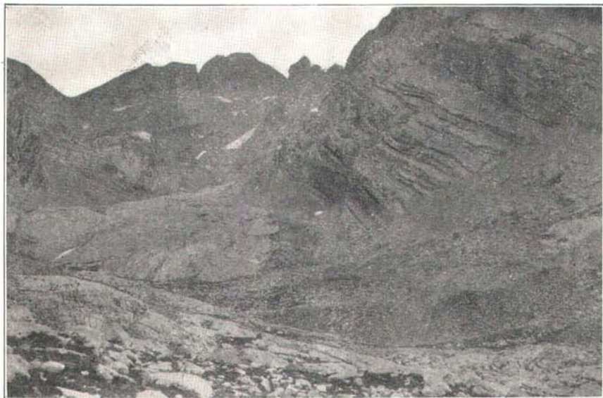
Fig. 1. Unterkretazischer Kalk bei Buni Koprištit.
