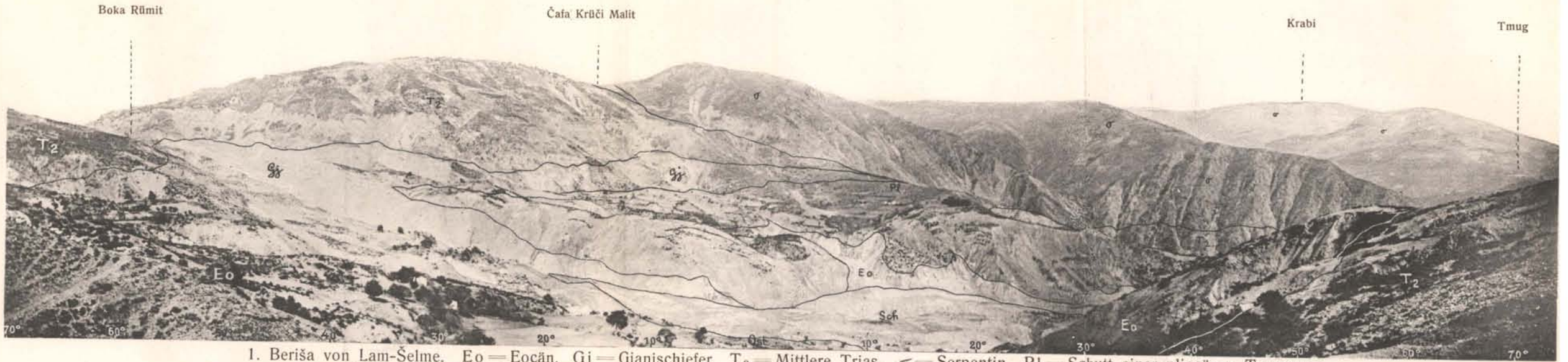
1. Beriša von Lam-Šelme. E o = Eocän. G j = Gjanischiefer. T 2 = Mittlere Trias. σ = Serpentin. Pl = Schutt einer pliocänen Terrasse. Sch = Schutt eines recenten Berggrutsches.
