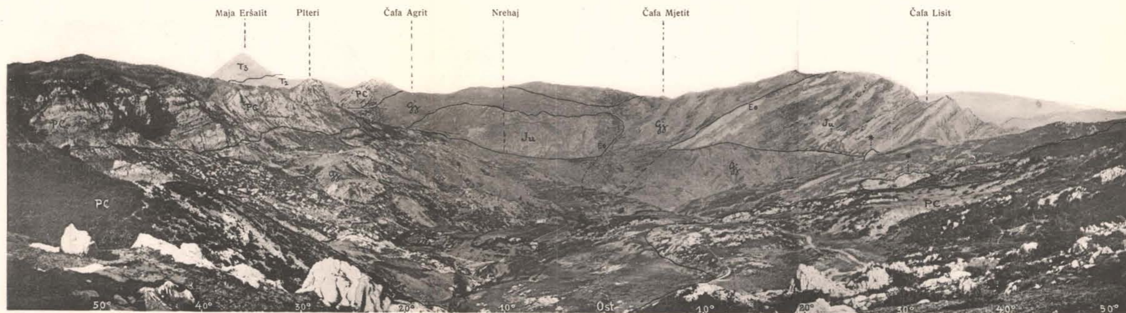
2. Panorama von Mlet i Keč gegen Osten. J_u = Mittlerer Jura. E_o = Eocäner Plattenkalk. G_j = Gjanischiefer. P_c = Permocarbon. T_2 = Mittlere Trias. T_3 = Obere Trias. * = Kalkeinschlüsse im Gjanischiefer.
