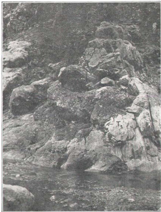
Fig. 2. Werfener Kalk ( T_1 ) und Porphyr ( \pi ) bei Met dü Rasave unweit Duši Eper.
