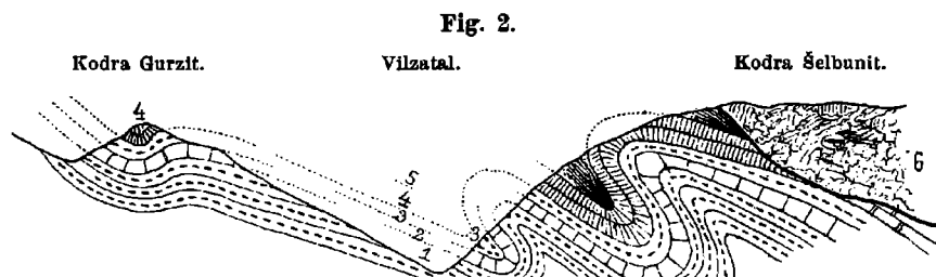
Profil im Vilzatal bei Kodra Gurzit.
