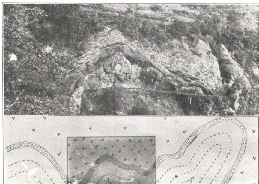
Fig. 2. Triasantiklinale im Gömsičebache unweit Kortpula und Diagramm des photographierten Teiles.
