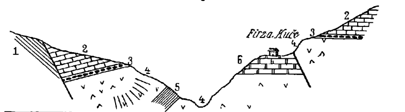
Profil durch die mittlere Trias bei Firza Kuče.
