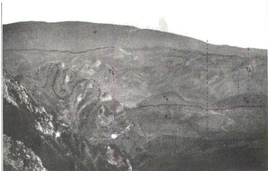
Fig. 1. Posteoecäne Falten der Maja Guß.
