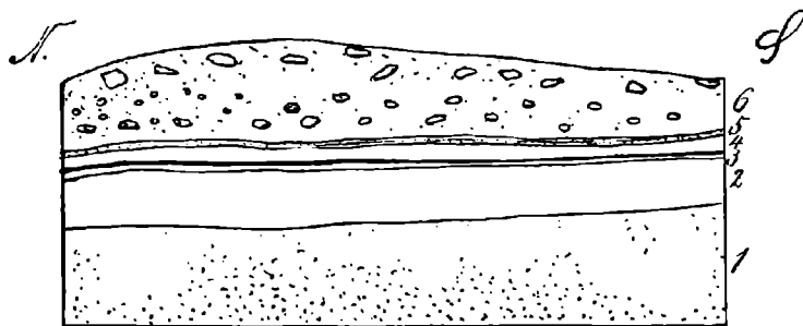
Profil einer Tongrube westlich von Kaplitz.
