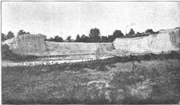
Sandschichten östlich von Dirnfellern.
