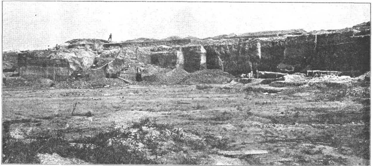
Die obersten Tonschichten des Tertiärs mit den darüber lagernden groben Sanden und Schottermassen beim Ziegelschlag östlich von Budweis.
