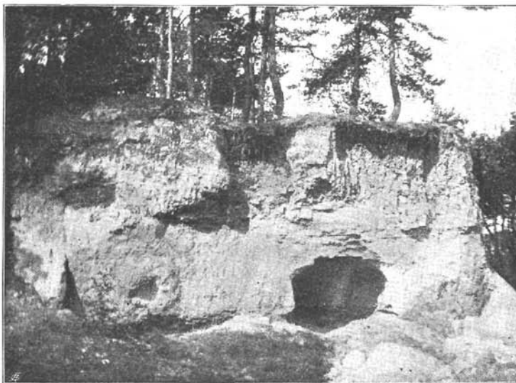
Strandbildungen bei Bida.
