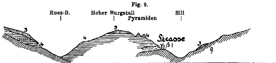
W. West-östl. Schnitt durch das Wipphthal wenig südl. von der Stefansbrücke. O. 3. Moräne α. 4. (mit Punktirung) Terrassen-Schotter; (ohne Punktirung) Terrassen Sand. γ? β? Moräne. 9. Grundgebirge.
