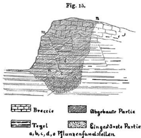
Nord-Süd-Schnitt durch die Tegelgrube.
