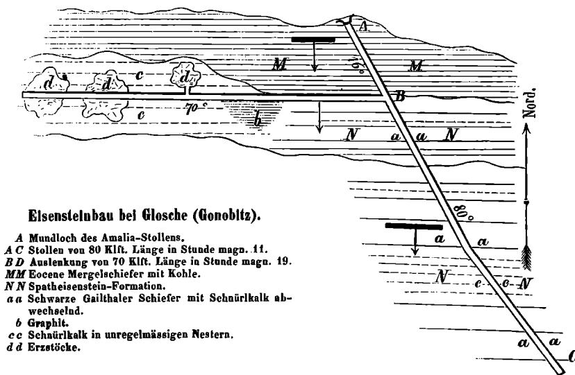
Figur 4 (Grundriss).
