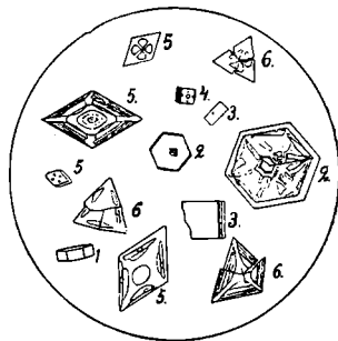
Fig. 14. Krystalle von Tantalsäure. AGNES CLEVE gez.
