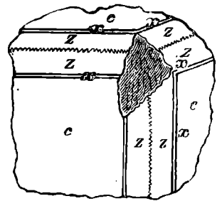
Fig. 4. Zwillingsartige Verwachsung beim Perowskit nach KOKSCHAROW.
