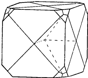
Fig. 15. Perowskitkrystall, zwillingsartig von 12 Individuen aufgebaut.
