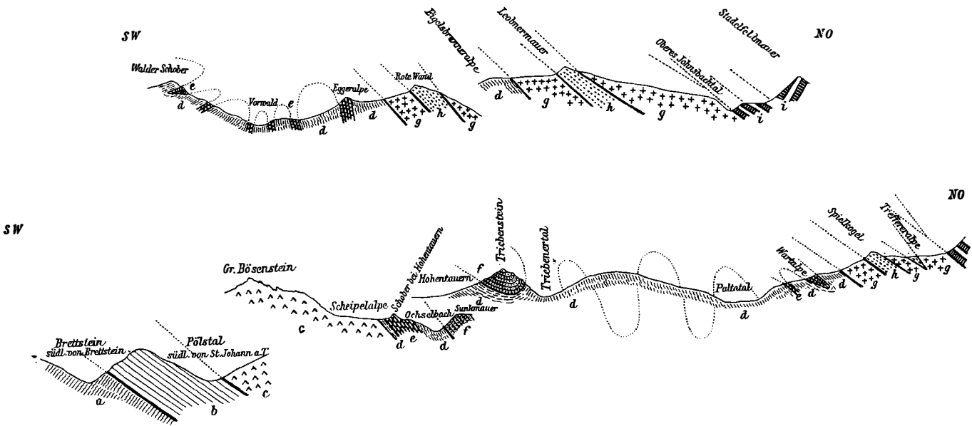
Generalprofil durch die Grauwackenzone des Paltentales (etwas schematisiert). Maßstab 1 : 75000.
