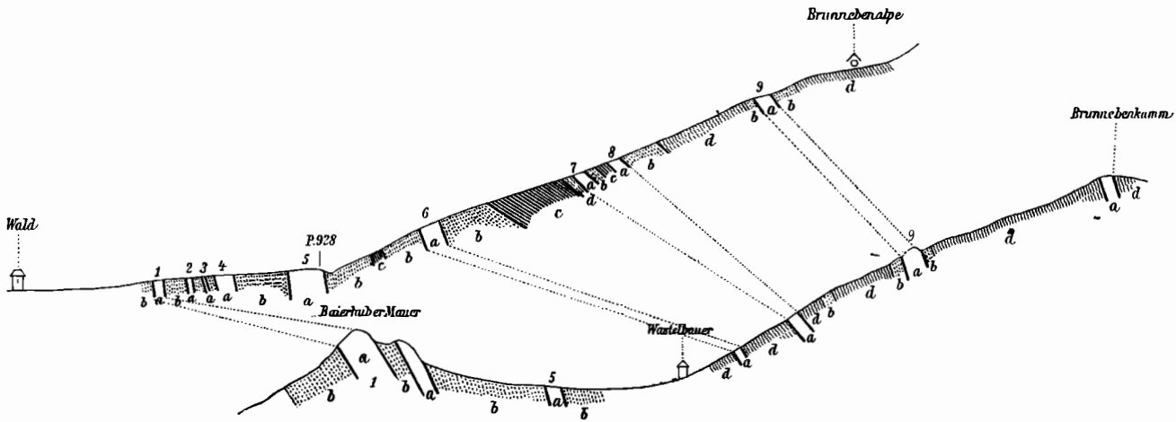
Profile von Wald-Brunneben und Baierhubermauer-Brunneben.
