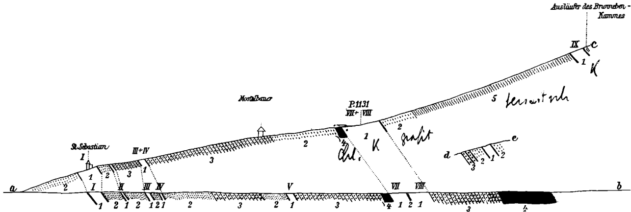
Profil durch die Hölle bei Kallwang ( a-b ) und über das Gehänge des Brunnebenausläufers bis Kallwang ( c-a ), d-e Profil im Langen Teichgraben.
