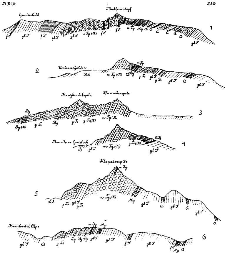
Fig. 1 bis 6. Übersichtsprofile durch die Klopaierspitzenkette (1:40.400). Tg = Tonalitgneis, Ts = Tonalitschiefer, a. Tg = amphibolitähnlicher Tonalitgneis, Dg = Dioritgneis, A Tg = Albitonalitgneis, qfTg = quarzfreier Tonalitgneis; A = Amphibolit, Gg = Biotitgranitgneis, Mg = Muskowitgranitgneis; gbS und fS = grobkrySTALLINER und feinschuppiger Schiefergneis, qS = quarzreiche Lagen in ersterem, a. Zg = aplitähnlicher Zweiglimmergneis, Q = Quarzgänge; B = Blockmoränen, S = Schutthalden. Ein vorgesetztes n oder g bezieht sich auf die helle (»weiße«) oder graue Färbung des Gesteins, ein nachgesetztes ( K ) oder ( k ) gibt merkliche bis spurenweise Mengen von Kalifeldspat an.
