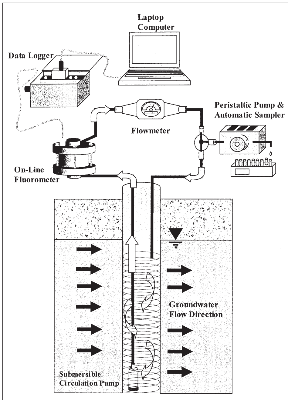
Fig. 3: Continuous circulation apparatus used to monitor tracer concentrations in injection well, K1-2 and observation well, K3-2. Note: automatic sampler not used in injection well setup. Apparatur mit kontinuierlichem Durchfluss zur Analyse der Tracerkonzentrationen im Eingabebrunnen (K1-2) und in der Messstelle (K3-2). Anmerkung: automatischer Probenehmer nur für die Messstelle.
