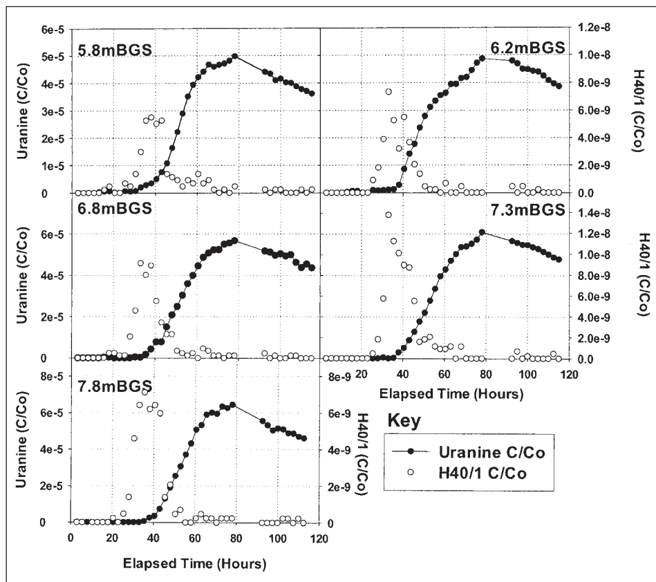
Fig. 4: Breakthrough curves for five different depths sampled using a multi-channel low-flow sampling system at K3-2, Kappelen Test Site, Switzerland. C/C_0 – injectate concentration, m BGS – metres below ground surface. Durchgangskurven in fünf verschiedenen Tiefen ermittelt mit Hilfe eines Multi-Level-Probenahme-systems an K3-2, Testgebiet Kappelen, Schweiz. C/C_0 -Injektatkonzentration, m BGS – Meter unter Geländeoberkante.
