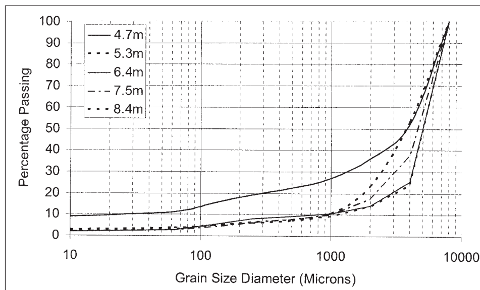
Fig. 2: Representative grain size distribution analyses for samples of aquifer material collected from depth corresponding to the screened interval of K3-2, Kappelen Test Site, Switzerland. Hydraulic conductivity estimated from HAZEN rule (R. A. FREEZE & J. A. CHERRY, 1979). Repräsentative Korngrößenverteilungskurven für Aquifermaterial aus verschiedenen Tiefen entsprechend der Filterstrecke von K3-2, Testgebiet Kappelen, Schweiz. Hydraulische Leitfähigkeit abgeschätzt nach der HAZEN-Regel (R. A. FREEZE & J. A. CHERRY, 1979).
