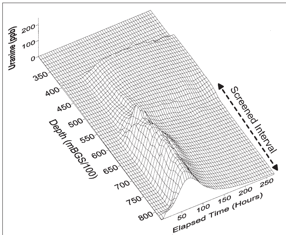
Fig. 5: Composite depth-specific breakthrough curve generated using mobile downhole fluorometer, K3-2, Kappelen Test Site, Switzerland. Note: tracer storage above screened interval due to tracer displacement by fluorometer during successive measurement cycles. Mittels eines mobilen in-situ-Fluorometers generierte tiefenspezifische Durchgangskurve, K3-2, Testgebiet Kappelen, Schweiz. Anmerkung: Tracerkonzentrationen oberhalb des verfilterten Bereichs aufgrund von Verschleppung durch das Fluorometer während der Messungen.
