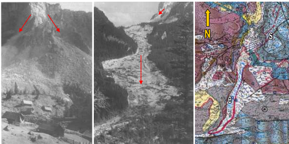
Abb. 17a, b, c: Sandling kurz nach der Felssturzkatastrophe von 1920 (links); der dadurch ausgelöste Erdstrom entlang des Michlhallbachs (Mitte, beides aus Marchetti 1991); Geologische Karte der Westseite des Sandlings (s) mit dem Michlhallbach Erdstrom (e), aus Geol. B.-A. 1982.
