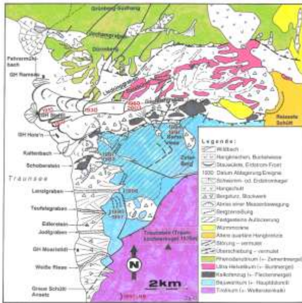
Abb. 3a (oben): Die Massenbewegungen des Gschlifgraben und der Traunstein-NW-Flanke (links, nach Daurer, Schäffer 1983, Prey 1983, Baumgartner 1981 und Weidinger 2003).
