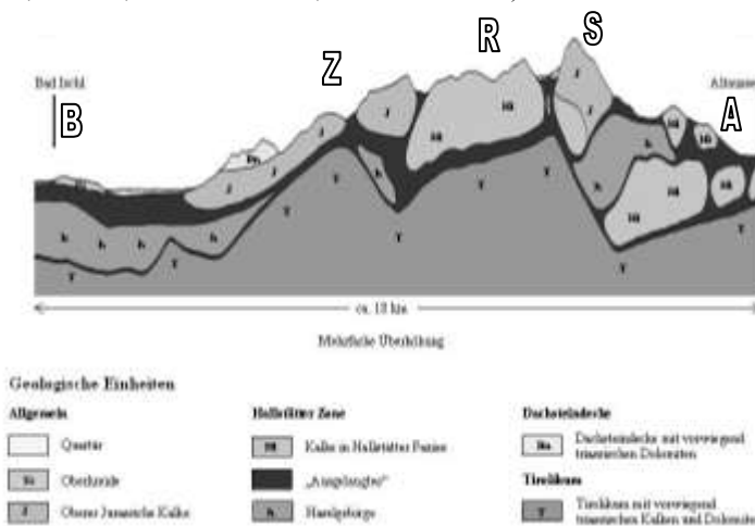
Abb. 15: Geologisches Profil Bad Ischl (B) – Altaussee (A) durch Zwerchwand (Z), Raschberg (R) und Sandling (S), nach Arndt, Mayr 2003.
