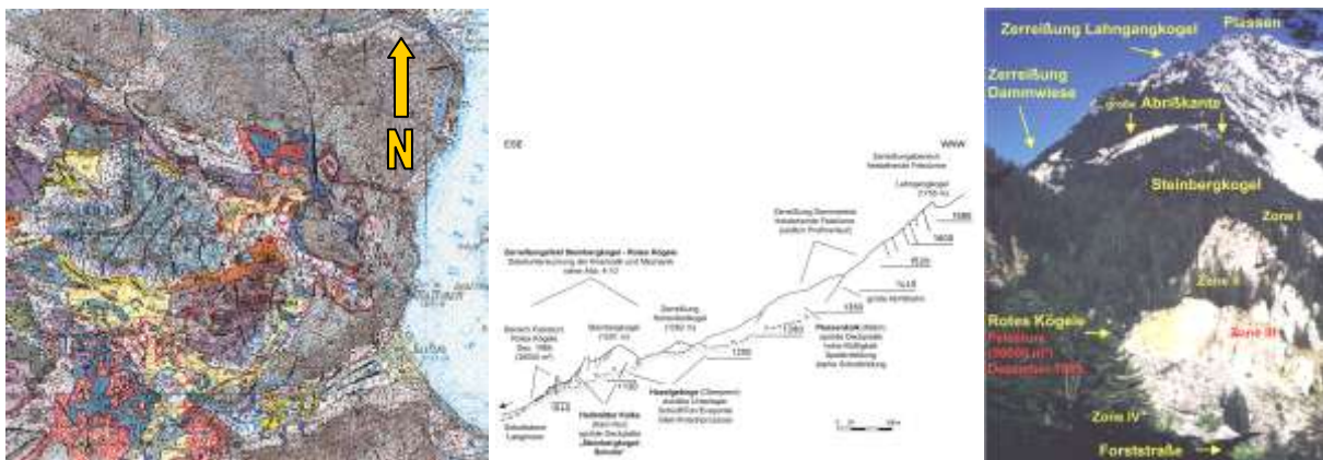
Abb. 18a, b, c: Geologische Karte der Ostseite des Plassen (aus Geol. B.-A. 1982); geotechnischer Längsschnitt durch die Großmassenbewegung der Plassen Ostflanke mit ihren vielfältigen Teilproblemen (aus Moser et al. 2003); E-W Blick auf die Bergzerreibungen der Plassen Ostflanke und das Felssturzgebiet der Roten Wand/Rotes Kögele (aus Moser et al. 2003).
