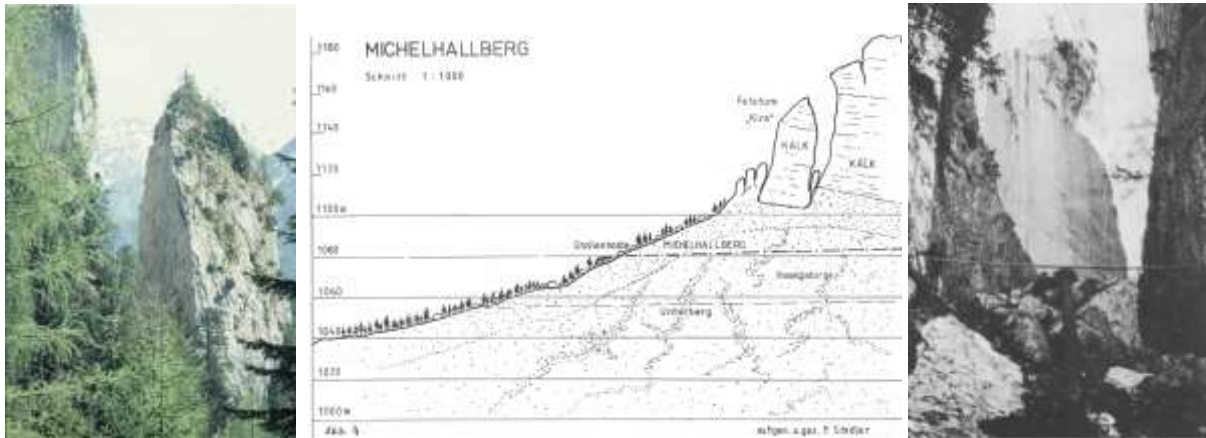
Abb. 16a, b, c: Der Felsturm der „Uh-sinnig Kira“ (links; Foto: J.T. Weidinger 1997), Profilschnitt durch diesen Bereich (Mitte) und die Rekonstruktion eines der ältesten geotechnischen Messvorgänge im Salzkammergut – die eingelegten Messstangen in den Felskerben der weit geöffneten Kluft zwischen dem Felsturm und dem Anstehendem (rechts), b und c aus Stadler 1986, 1991.
