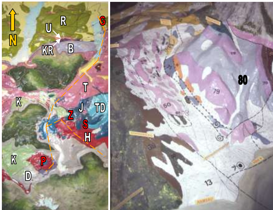
Abb. 1b: Relief-Modell des Salzkammerguts mit der geologisch-tektonischen Gliederung vom Traunstein (1.691m) am Nordrand der Kalkalpen zum Massiv des Hohen Dachsteins (2.995m) nach den Geol. Karten der Rep. Österr. Blatt 66 Gmunden (Geol. B.-A. 1996) und Blatt 96 Bad Ischl (Geol. B.-A. 1982); U – Ultra-Helvetikum, R – Rhenodanubikum od. Flyschzone, KR – Kalkalpine Randschuppe od. Randcenoman, B – Bajuvarikum (Langbathzone, Zirler Scholle), T – Tirolikum (Höllengebirgsdecke, Haslergupf-Deckscholle), H – Hallstätter Zone, TD – Totengebirgsdecke, D – Dachsteindecke, J – Jura, K – Kreide (Gosau); Lage der Untersuchungsgebiete: G – Gschlifgraben, Z – Zwerchwand, S – Sandling, P – Plassen, (---) Exkursionsroute (links); 1c: Geologisch-tektonische Situation im Gschlifgraben und am Nordfuß des Traunsteins (Modell 1:2000 im Stadtmuseum Gmunden nach Geol. B.-A. 1996; rechts).
