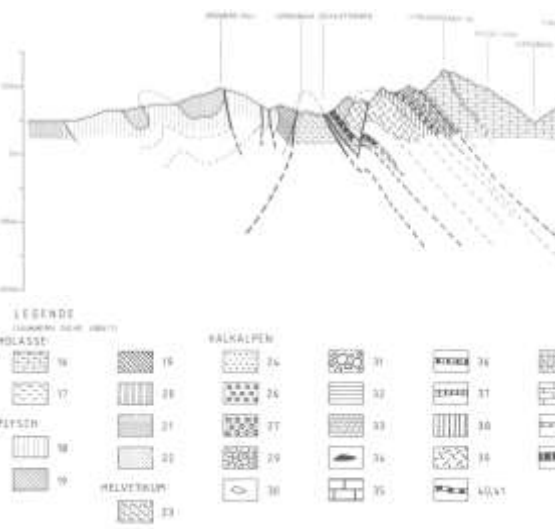
Abb. 3b (unten): N-S Profilschnitt durch Grünberg (Rhodanubikum), Gschlifgraben (Ultra-Helvetikum) und Traunstein (Kalkalpin), aus Daurer, Schäffer 1983; Legende: 18 – Mürlsandsteinführende Oberkreide, 19 – Obere Bunte Schiefer, 20 – Zementmergelerde, 21 – Reiselberger Sandstein, 22 – Gaultflysch, 23 – Helvetikum, 26 – Rossfeldschichten, 27 – Neokom, 32 – Fleckenmergel, 33 – Kieselkalk, 36 – Kössener Kalk, 37 – Kössener Mergel, 38 – Plattenkalk, 39 – Hauptdolomit, 43 – Wettersteinkalk, 44 – Gutensteiner Kalk, 45 – Haselgebirge.
