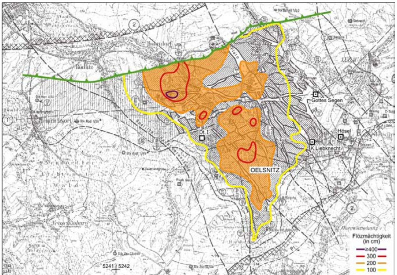
Abb. 1b: Mächtigkeitsdarstellung des Glückaufflöz im Lugau/Oelsnitzer Revier (LOBST 1983, Anl. 21). 100-200-300- \geq 400-cm-Isopachen hervorgehoben. Schräg schraffiert: ausgekohlte Flächen. Grüne Zackenlinie: Grenze der permischen Flözerosion. Hervorgehobene Quadrate: Schächte der beprobten Bereiche, davon Quadrate mit Punkt: Schächte mit charakteristischer Verbreitung der Neuoelsnitz-Subformation
