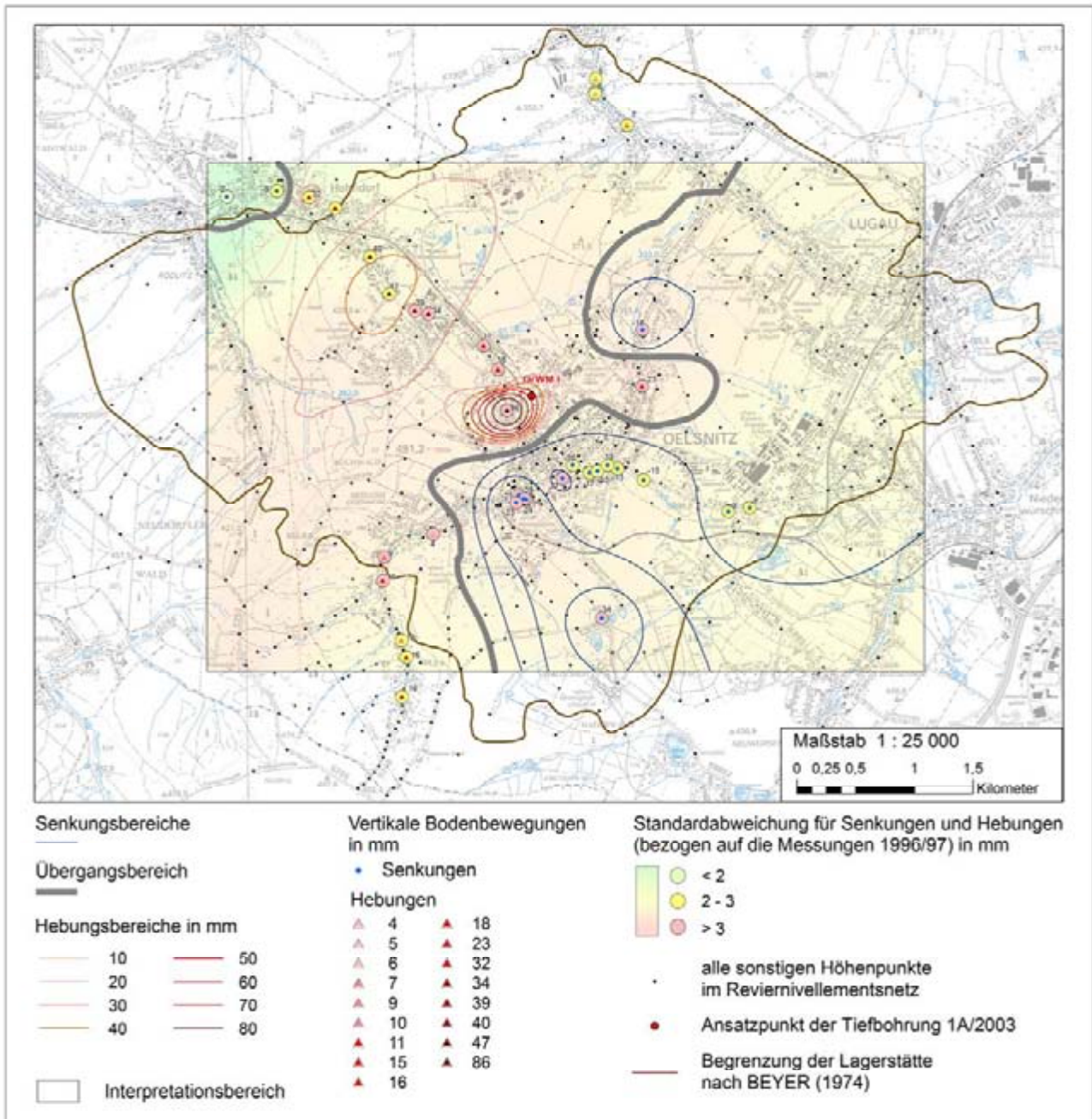
Abb. 17: Vertikale Bodenbewegungen von 1972 bis 1996/97 (Löbel, Döhner), Ausschnitt aus Felix u. a. (2007)
