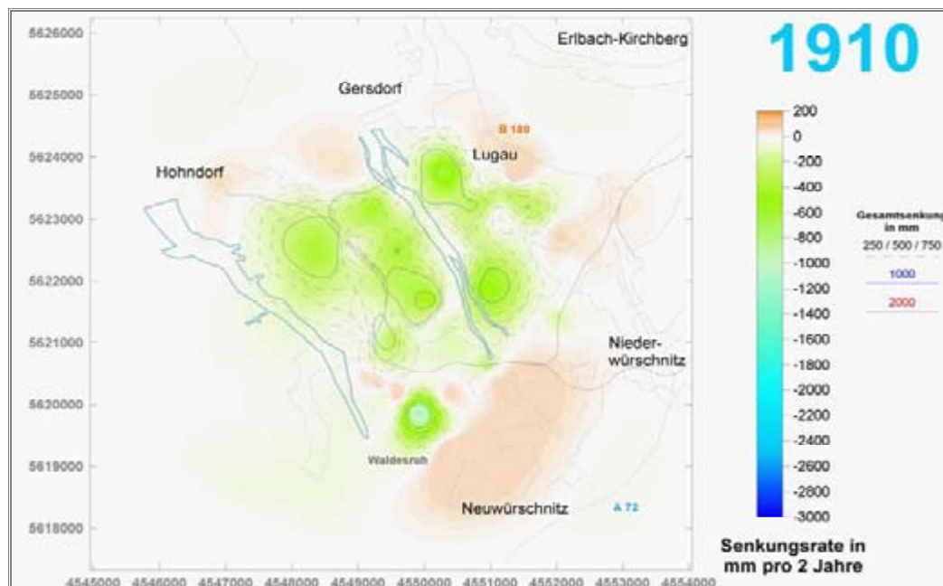
Abb. 11: Visualisierung der Senkungsraten mit Störungen und Isokatabasen
