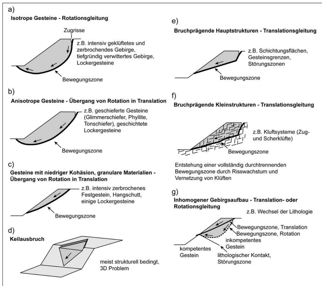
Abb. 9. Unterschiedliche Arten des Gleitens: a) Rotationsgleitung in isotropen, homogenen Gesteinen, b) Übergang zwischen Rotations- und Translationsgleitung in anisotropen Gesteinen, c) Translationsgleitung in granularen Materialien mit niedriger Kohäsion, d) strukturell bedingter Keilausbruch (3-D Problem), e) strukturell, d.h. durch prä-existierende spröde Störungszonen oder Schichtungsflächen bedingte Translationsgleitung, f) strukturell beeinflusste, d.h. prä-existierende Klüfte vernetzten sich zu einer zusammenhängenden Bewegungszone und führen zu einer Translationsgleitung und g) ein lithologisch inhomogener Gebirgsaufbau wie z.B. kompetentes Gestein im Hangfuß kann die Ausdehnung der Bewegungszone für eine Translations- oder Rotationsgleitung limitieren (modifiziert und ergänzt nach Hudson & Harrison 1997).
