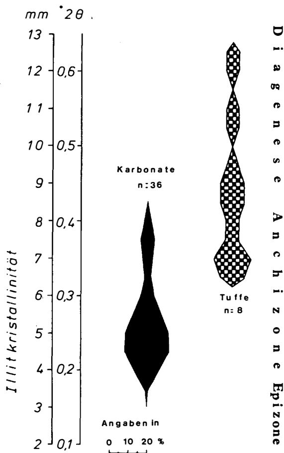
Abb. 6: Häufigkeitsverteilung der Illit-Halbhöhenbreiten, getrennt nach Karbonaten und Tuffen.
