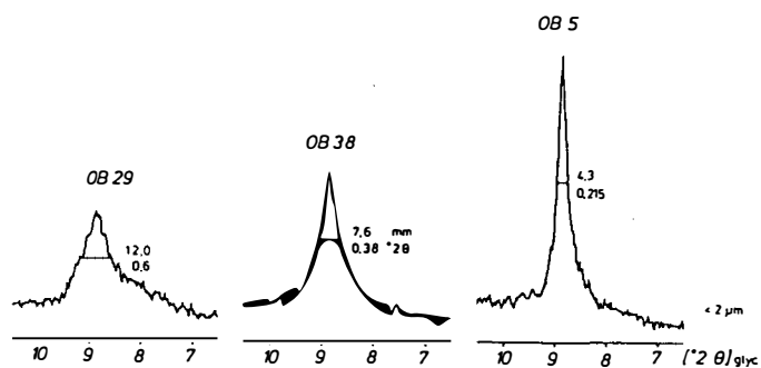
Abb. 4: Illit-Basisreflex und Halbhöhenbreite von drei Proben aus dem Profil Öfenbach. Fraktion kleiner 2 \mu\text{m} . Von links nach rechts nimmt die Halbhöhenbreite der Illit-Basisreflexe ab, d.h. die Illitkristallinität nimmt zu! Die Probe OB 29 stammt aus einer Tufflage; OB 38 aus dem Reiflinger Knollenkalk und OB 5 aus dem Steinalmkalk.
