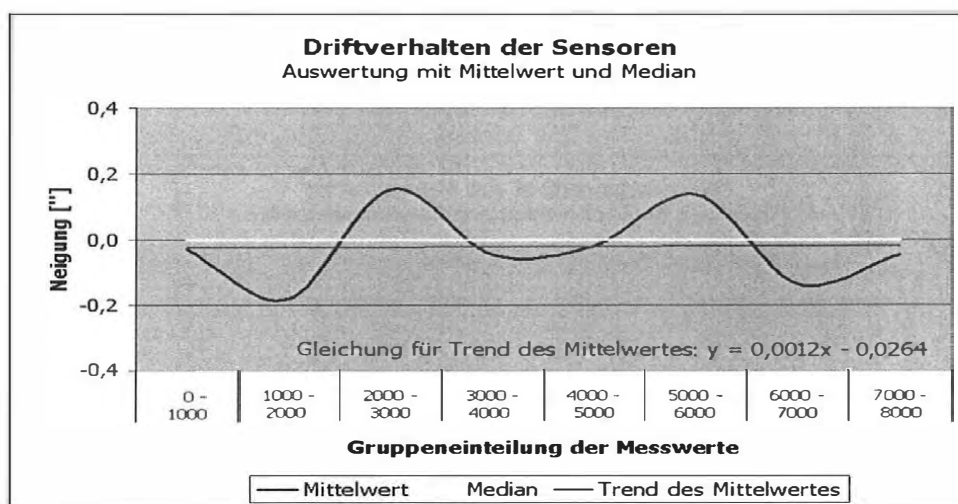
Driftverhalten der Sensoren (Auswertung mit Mittelwert und Median)
