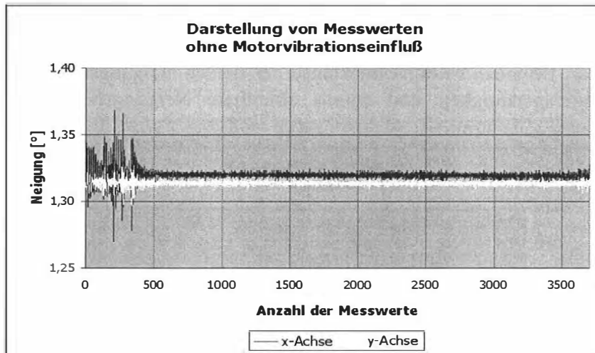
Messwertreihe ohne Einfluss von Motorvibrationen
