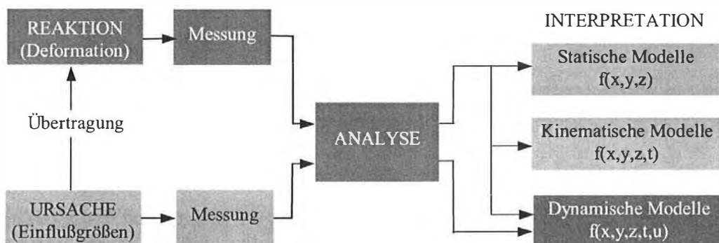
Abb.1. Interpretationsmodelle der Deformation
