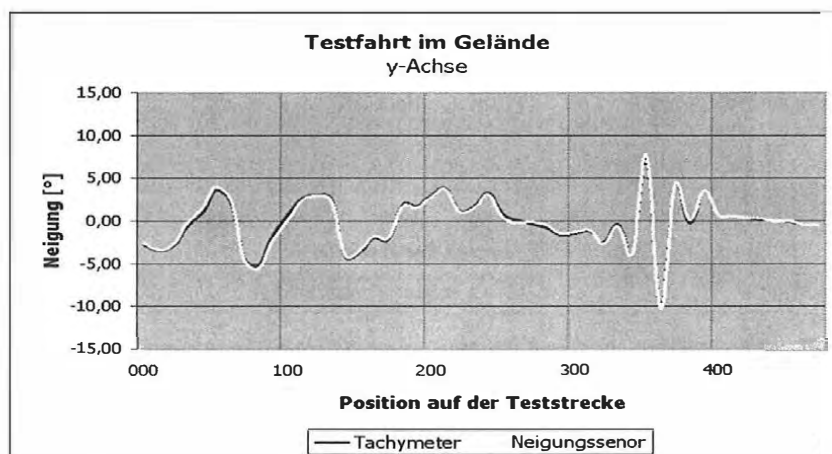
Neigungskurve als Ergebnis der Testfahrt im Gelände für die y-Achse
