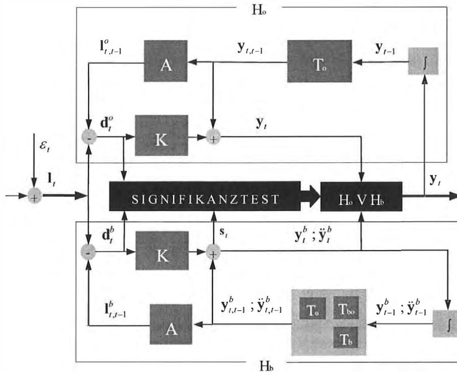
Abb.5. Adaptives Filtermodell mit zwei Parallelfiltern
