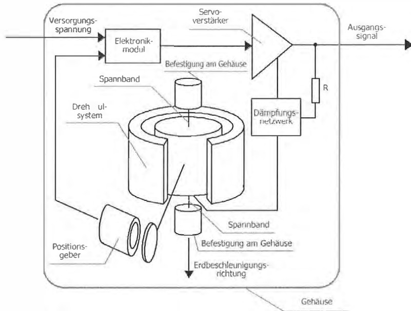
Prinzipische Skizze eines Inclinometers [Reißner, 1999]
