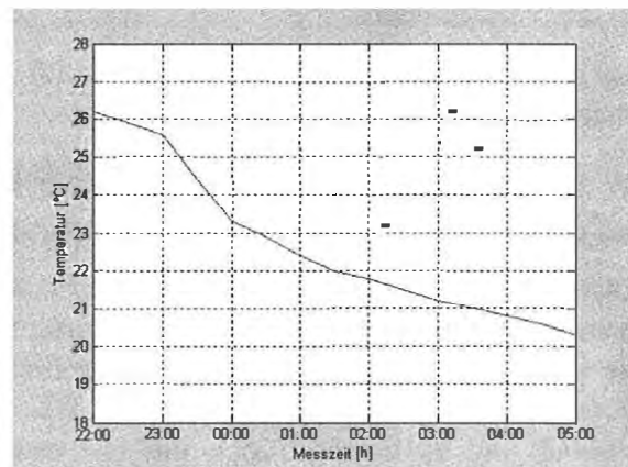
Abb. 5: Gemessene Lufttemperaturen
