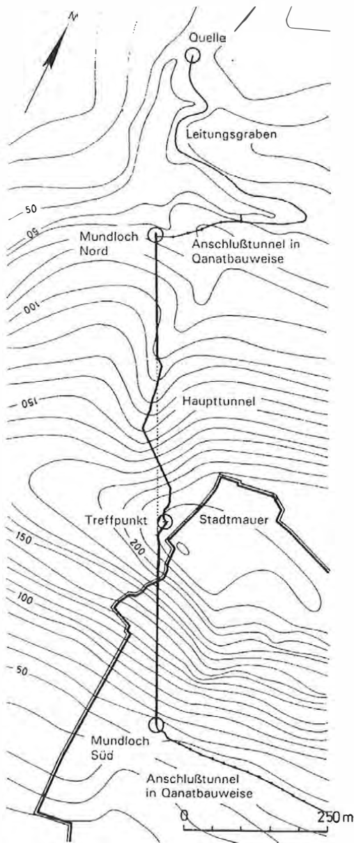
Abb. 1: Eupalinos-Tunnel nach Grewe [1998] und Kienast [1977]
