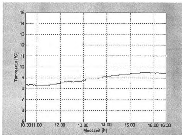
Abb. 9: Gemessene Lufttemperaturen
