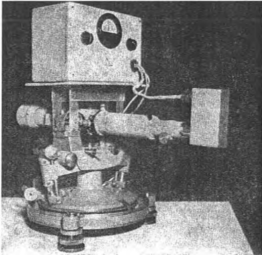
Bild 1: Elektrisches Auge des IFAG
