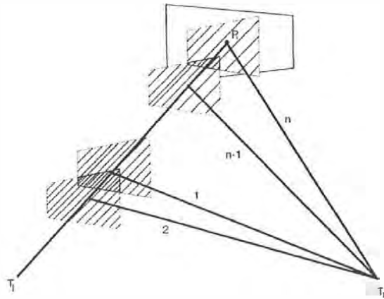
Abb. 7: Tracking-Verfahren des Slave-Theodolits
