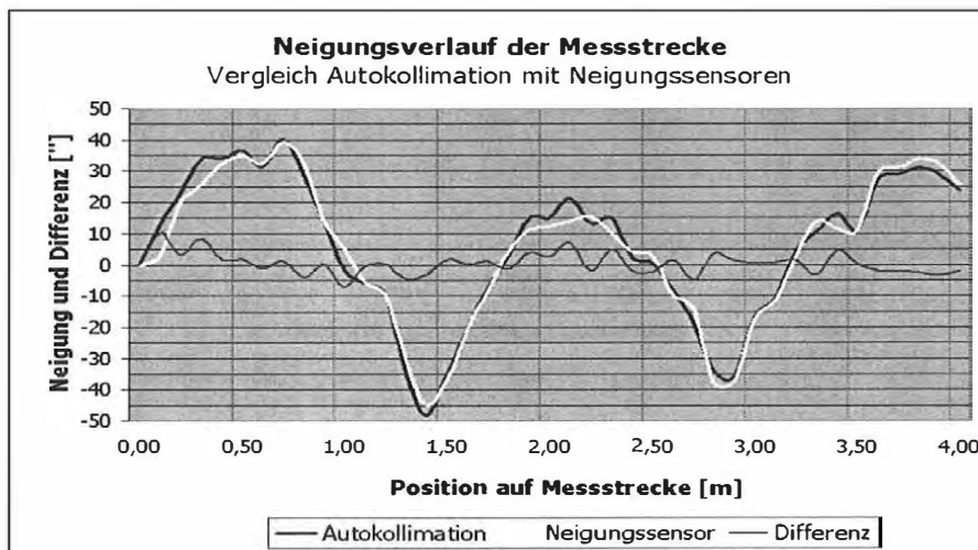
Vergleich der gemessenen Neigungen
