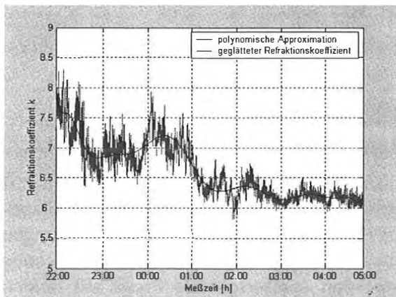
Abb. 4: Gang der Refraktionskoeffizienten
