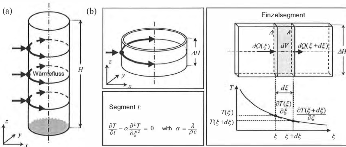
Abbildung 3: Modellierung des Wärmeflusses in finiten Mantelsegmenten
