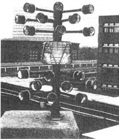
Bild 3: Hg-Lichtquelle/Raumreflektor
