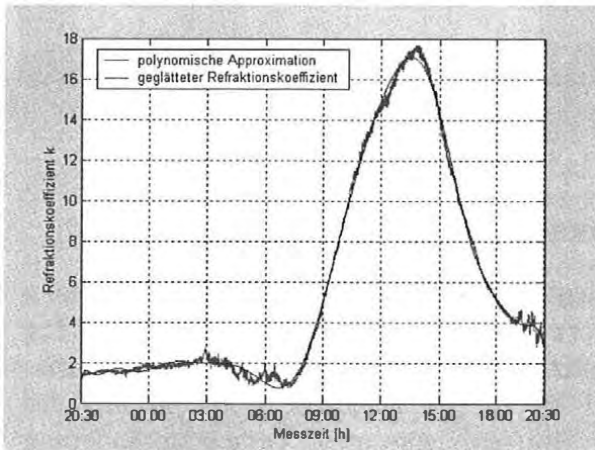
Abb. 6: Gang der Refraktionskoeffizienten
