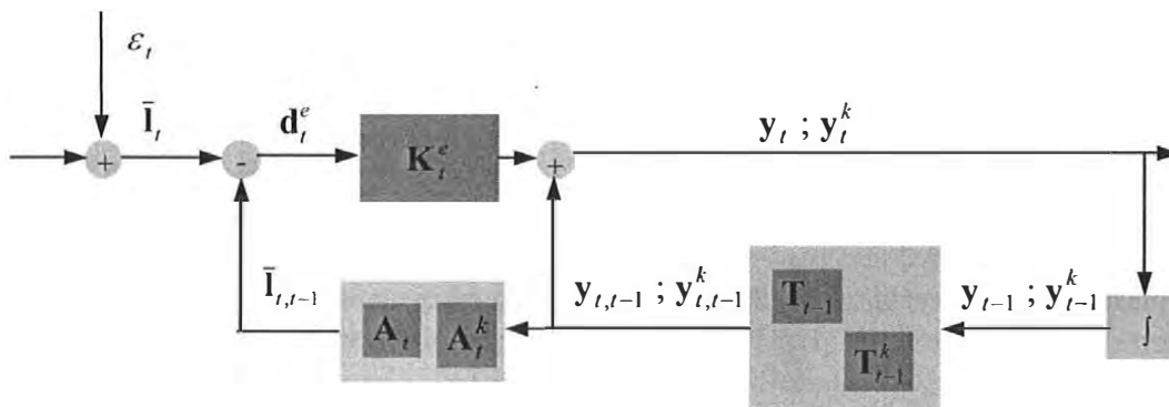
Abb.4. Erweitertes Kalman-Filter (Formfilter)
