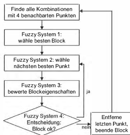
Abbildung 2: Gesamtschema des Algorithmus.
