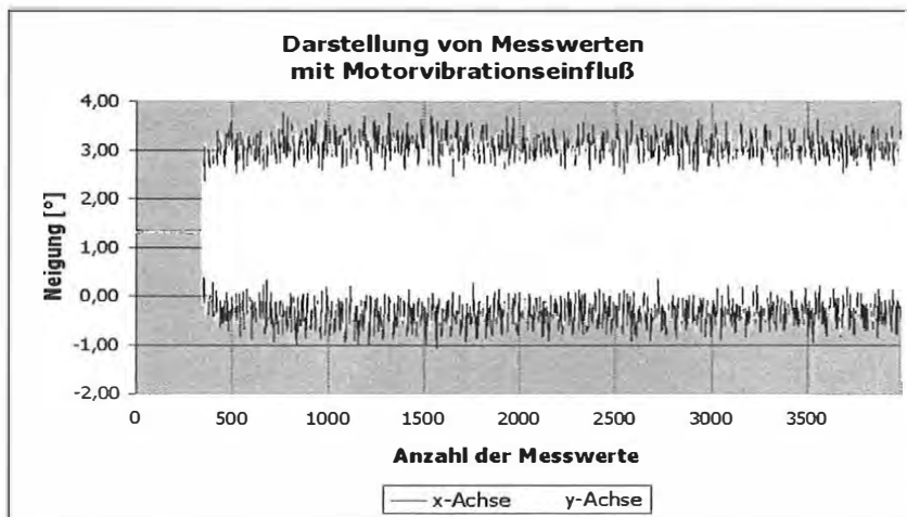
Messwertreihe mit Einfluss von Motorvibrationen
