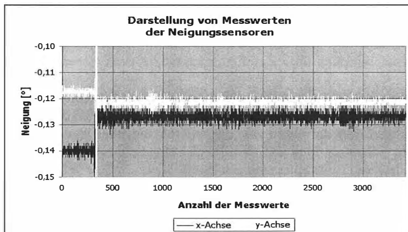
Darstellung von Messdaten der Neigungssensoren
