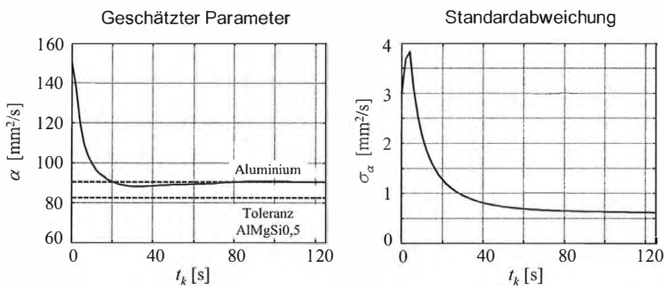
Abbildung 4: Ergebnisse der Identifikation von \alpha
