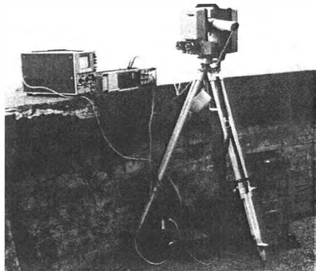
Bild 4: Prototyp des GEOROBOT
