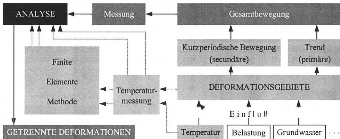
Abb.2. Zustandsschätzung im dynamischen Modell
