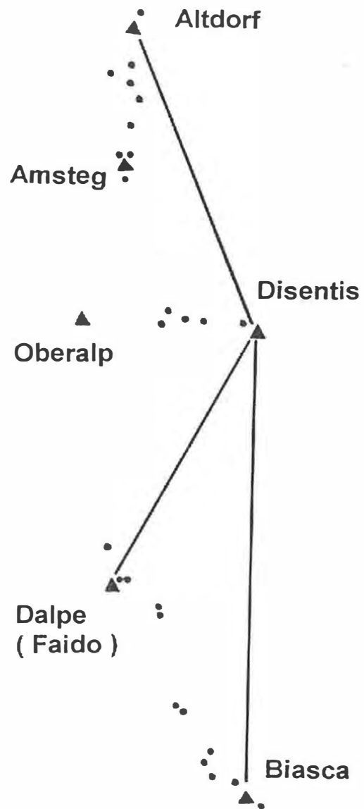
Abb. 3: GPS-Netz des Gotthard-Basistunnels nach Haag u.a. [1996]; die Punkte Biasca, Dalpe, Disentis u. Aldorf waren permanent besetzt
