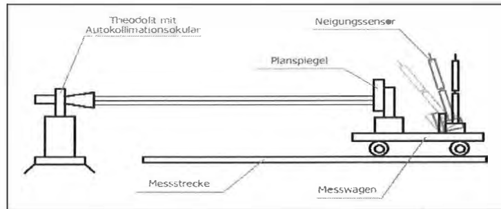
Prinzipische Skizze der Messanordnung für die Autokollimation
