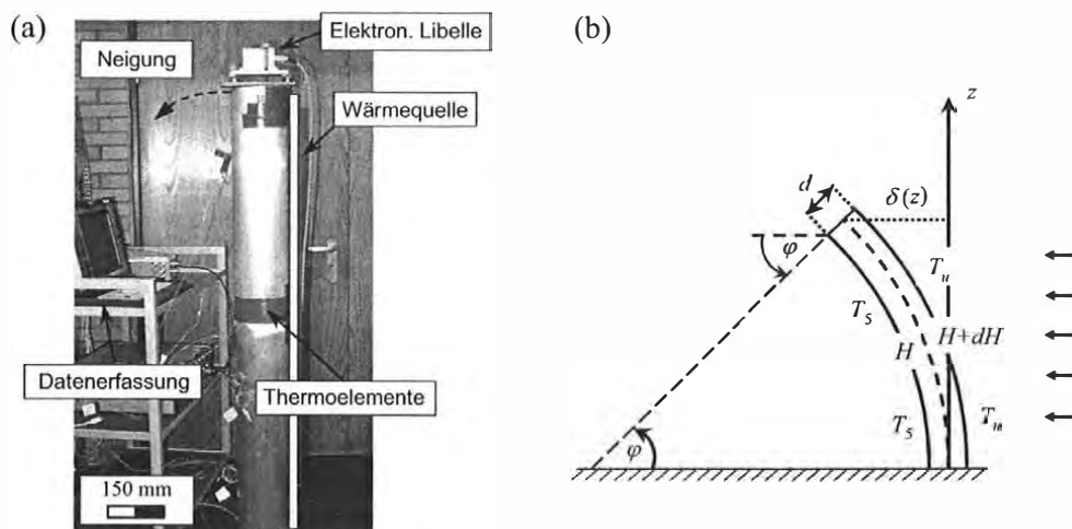
Abbildung 5: Thermische Biegung der Säule
