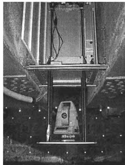
Abb. 2 : Die Fallersleber-Tor-Brücke und der ausfahrbare Support für das automatische Tachymeter
