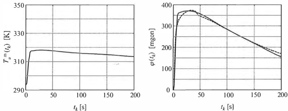
Abbildung 6: Vergleich von gemessener und gerechneter Säulenneigung \varphi
