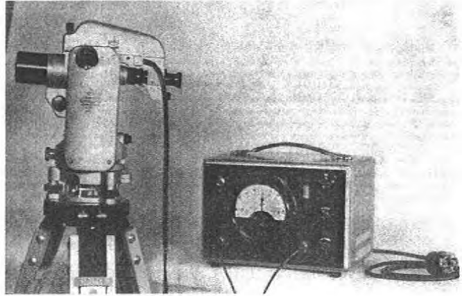
Bild 2: ASKANIA Theodolit für elektrische Zielung
