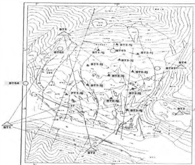
Abb. 4 : Baota Landslide im Hinterland des Drei-Schluchten Staudamms in China
