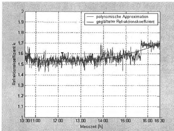
Abb. 8: Gang der Refraktionskoeffizienten
