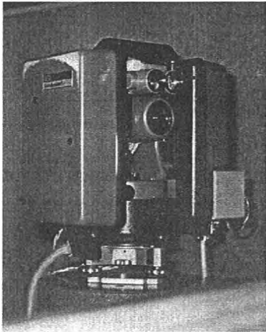
Abb. 5: GEOROBOT
