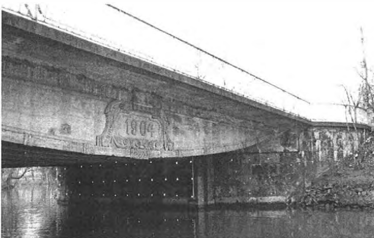
Abb. 2 : Die Fallersleber-Tor-Brücke und der ausfahrbare Support für das automatische Tachymeter
