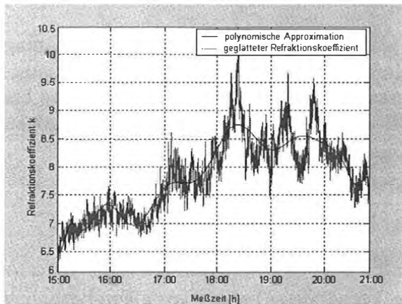
Abb. 2: Gang der Refraktionskoeffizienten
