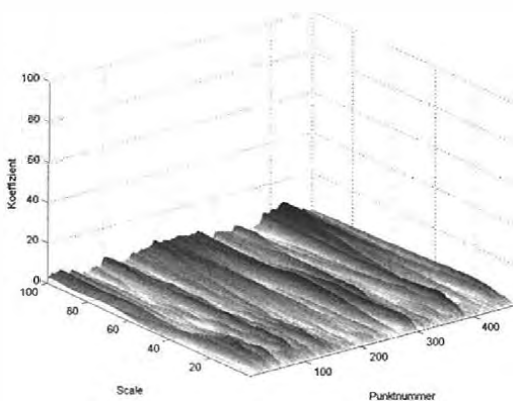
Abb. 13: Differenz-Wavelet-Transformation des Kreises bei kleinen Deformationen (0,3%)
