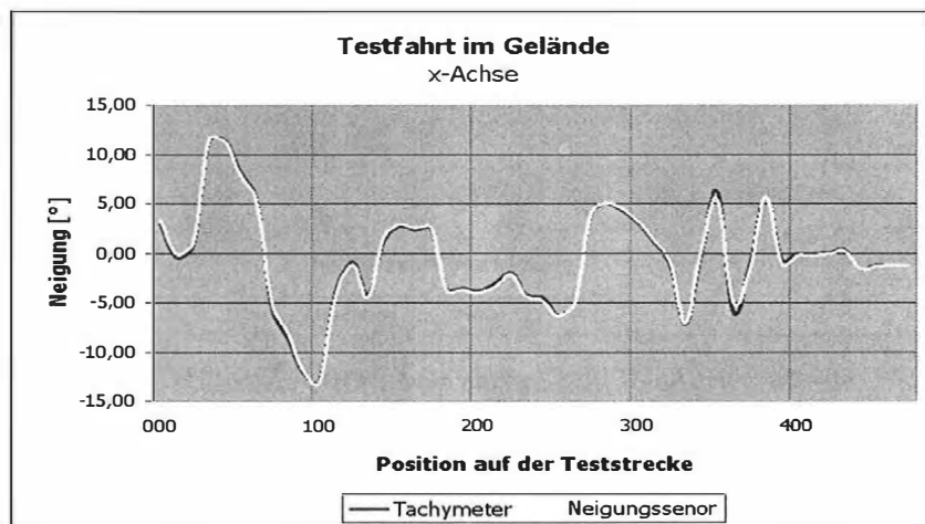
Neigungskurve als Ergebnis der Testfahrt im Gelände für die x-Achse
