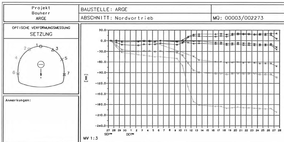
Abb.: Setzungsentwicklung von sieben Messpunkten in Messquerschnitt 3
