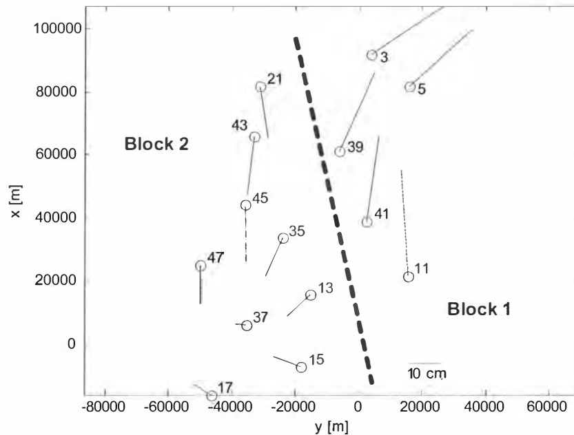
Abbildung 3: Übersicht über die Verschiebungsvektoren zwischen den beiden Messepochen. Die beiden detektierten Blöcke werden durch eine strichlierte Linie getrennt, die der Verwerfungszone entspricht.
