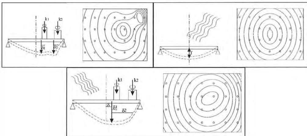
Abb.3. Periodischer Temperatureinfluss und durch Belastung verursachte Deformation
