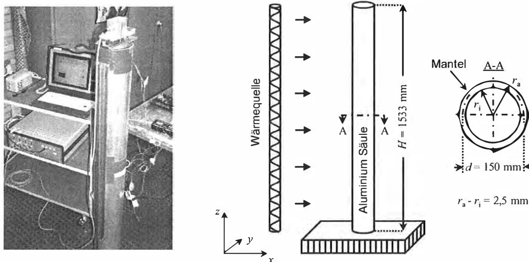
Abbildung 2: Einseitige thermische Belastung einer Aluminiumsäule
