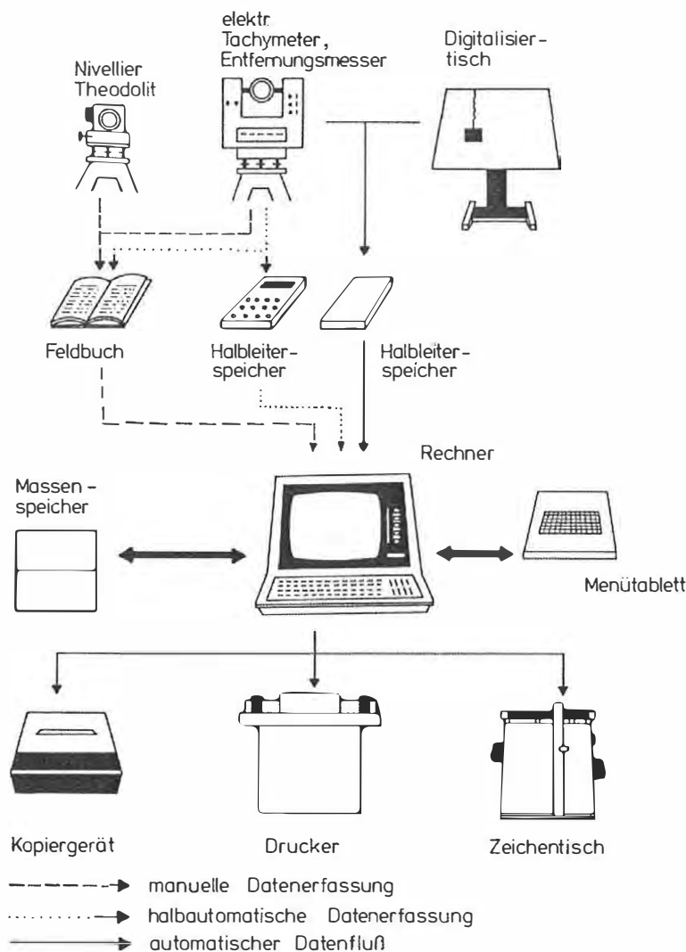
Abb. 4: Komponenten eines interaktiven Vermessungssystems (1981)
