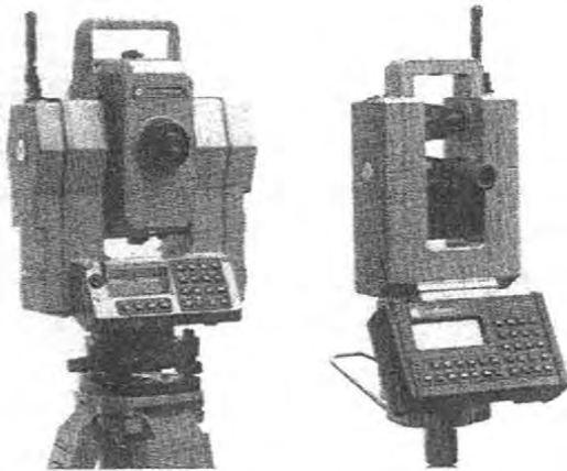
Bild 8: GEODIMETER 4000 mit Remote Positioning Unit
