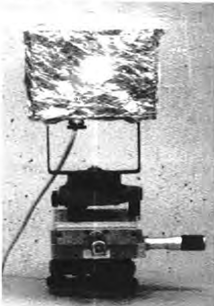
Abbildung 6.1 Aktive Zielmarke
