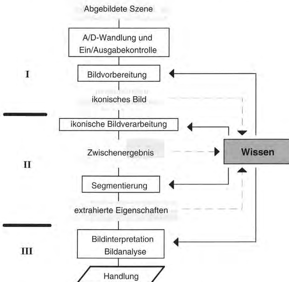
Abbildung 3.3 Prinzipielle Struktur einer Meßbildverarbeitungsanlage.
