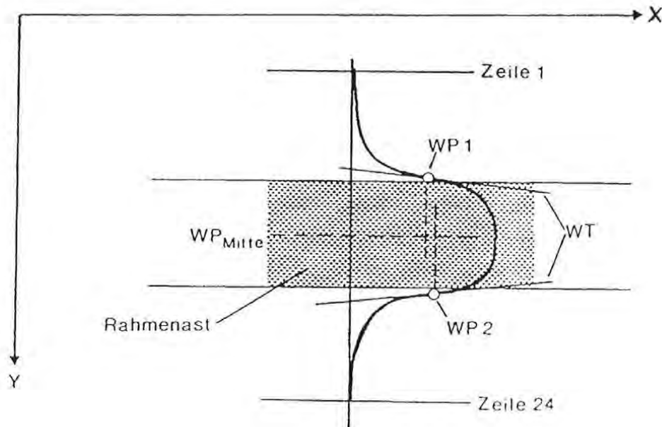
Abbildung 2.8 Bestimmung der Wendepunkte (WP ... Wendepunkte, WT ... Wendetangenten)
