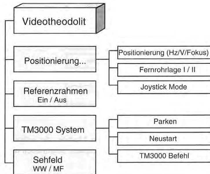
Abbildung 3.2 Untermenü Videotheodolit
