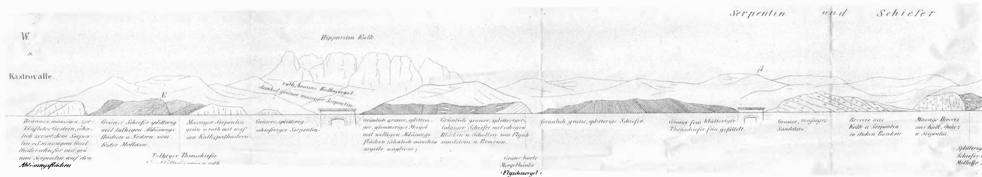
Profil an der Strasse von Kastrovalle nach Kumi auf Euboea.
