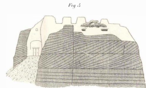
Höchster Punkt des Festungsberges von Gerace Bryozoenkalk mit falscher Schichtung
