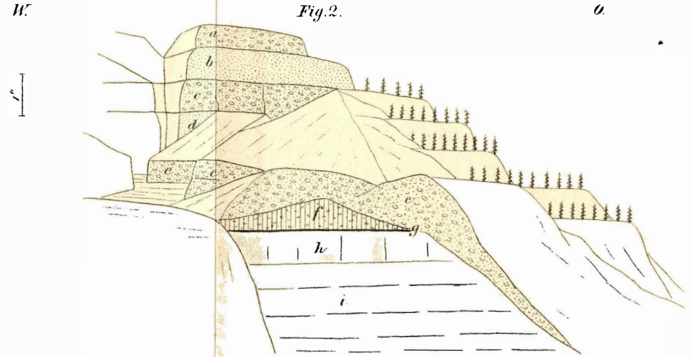
Aus dem Thale von San Nicola.
