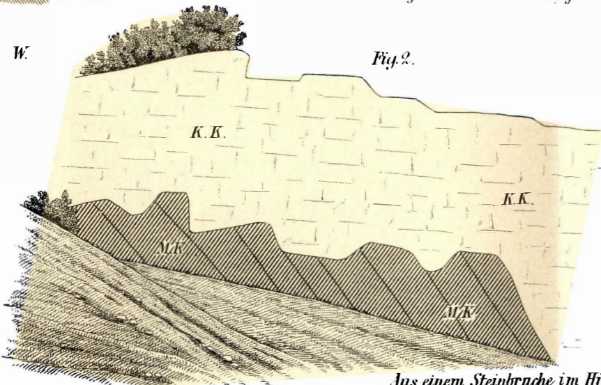
Aus einem Steinbrüche im Hintergrunde des Thales von Scoppo. M.K. Miocener Kalkstein. K.K. Korallen Kalk (Zandéen) W.M. Weisse Mergel (Zandéen)
