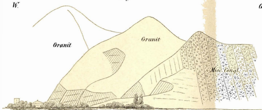
Anhöhen hinter Cattarratti.
