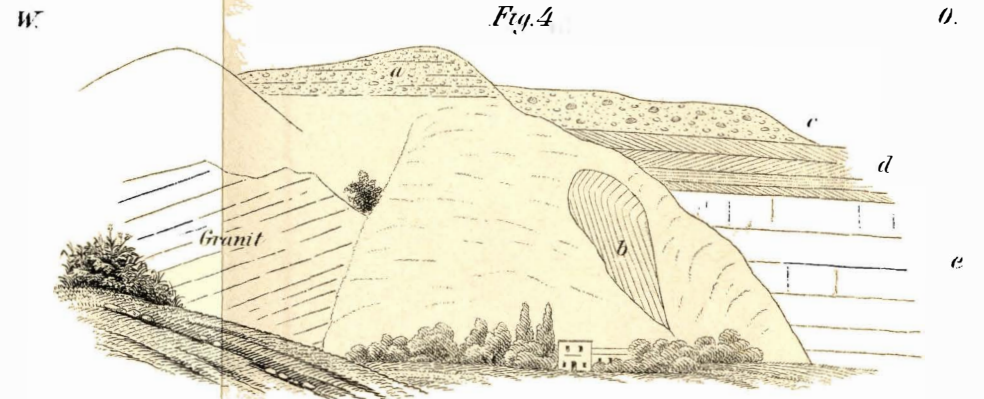
Anhöhen nördlich von Cattarratti.
