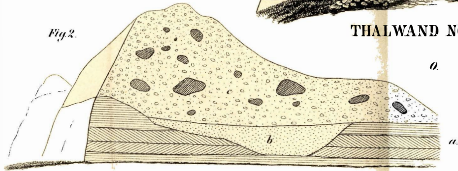
Hinter dem Forte Gonzaga.
