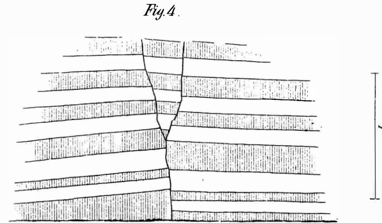
Nördlicher Abhang des Stadtberges von Gerace an der neuen Strasse nach dem Monte Jejunio. Weisse gebänderte Mergel (Zandéen) von Verwerfungen durchsetzt.
