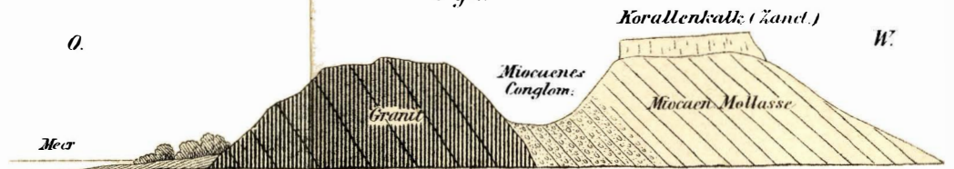
Durchschnitt durch das Küstengebirge südlich von Messina.
