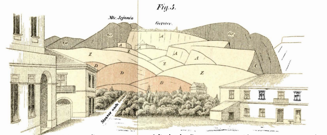
Ansicht von Gerace paesi v. d. Bahnhofstation am Meere (Gerace marina). D. Diluvialschotter. Z. Weisse Mergel (Zandéen). A. Bryozoenkalk (Astien). Gr. Granit (Grundgebirge).
