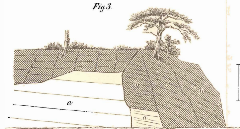
An der Strasse nach Gerace. a. Weisse Mergel. b. Bryozoenkalk.
