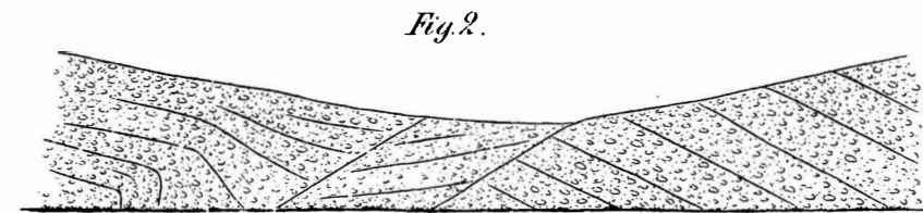
An der Strasse nach Gerace. Diluvial Schotter mit gestörter Lagerung.
