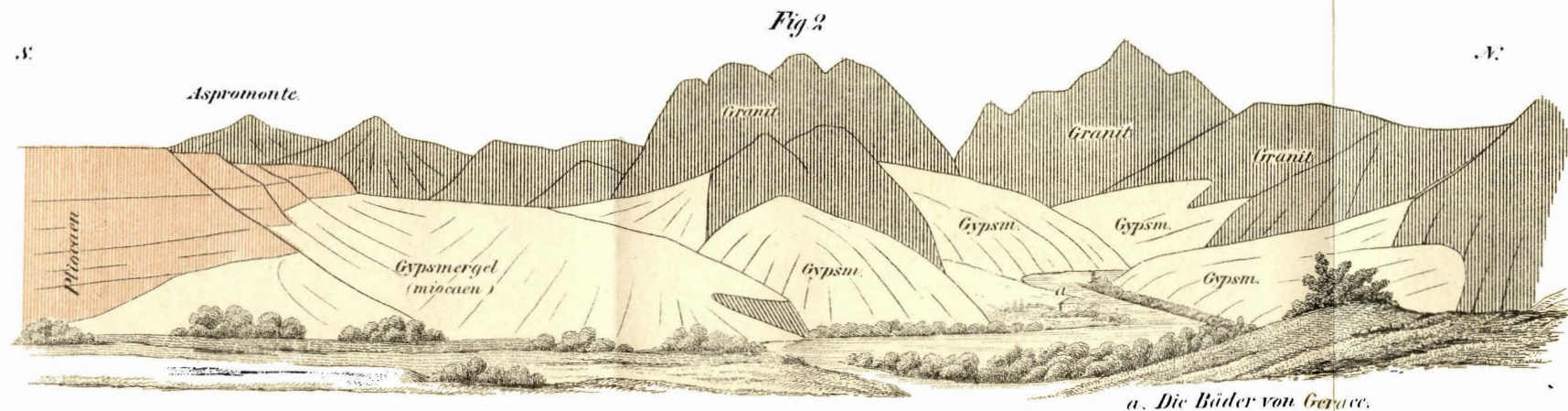
Das Thal des Merico süd. von Gerace.
