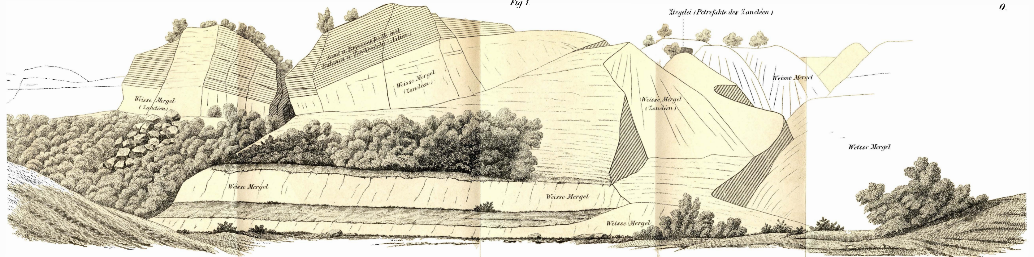
AUS DEM THALE VON GERACE. (Linke Thalseite.)
