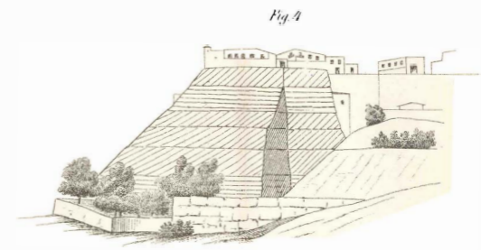
Aus der Stadt Gerace Bryozoenkalk mit falscher Schichtung
