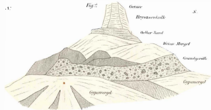
Ansicht von Gerace aus dem Westen vom Monte Iguzzo aus
