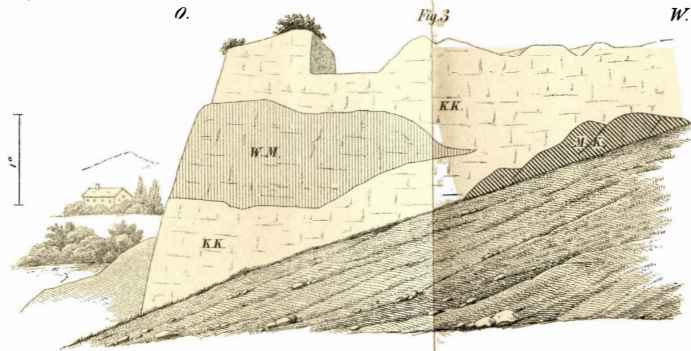
Aus einem Steinbrüche im Hintergrunde des Thales von Scoppo. M.K. Miocener Kalkstein. K.K. Korallen Kalk (Zandéen) W.M. Weisse Mergel (Zandéen)
