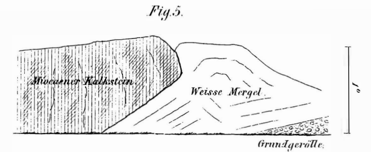
An der Strasse nach Gerace.
