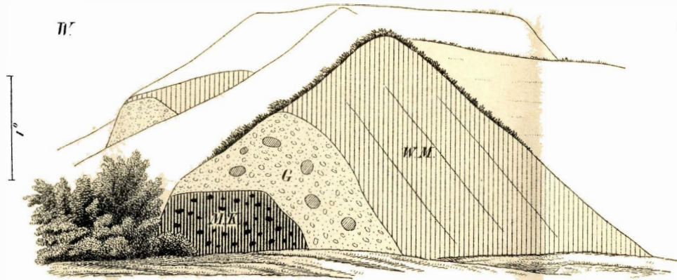
Im Hintergrunde des Thales von San Nicola
