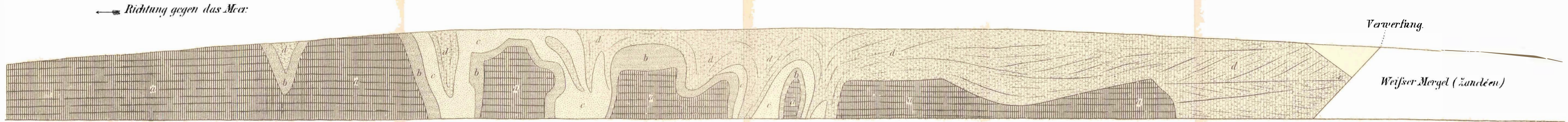
An der Strasse von Gerace
