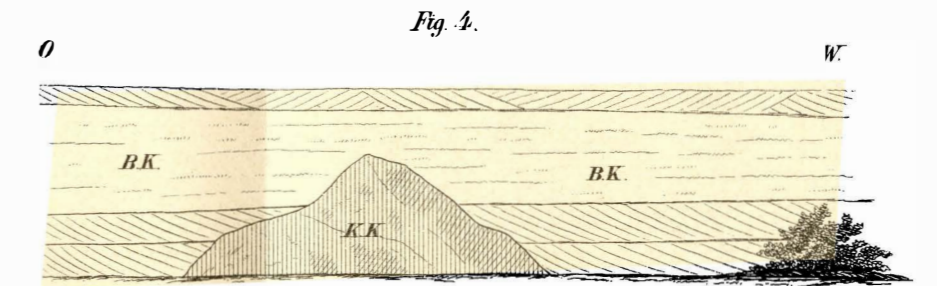
Aus der Klause von Scoppo. K.K. Korallen Kalk (Zandéen) klippenartig in den Bryozoen Kalk, B.K. Astien, aufragend.
