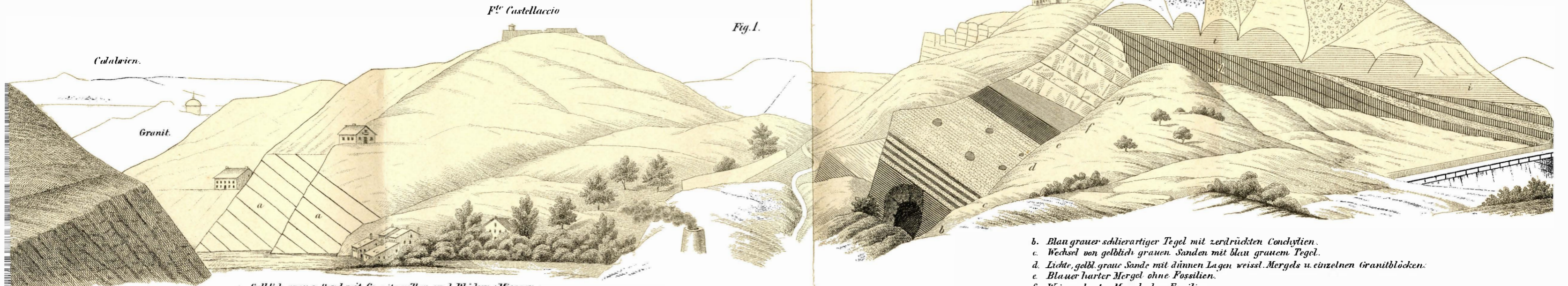
a. Gelblich grauer Sand mit Granitgeröllen und Blöcken (Miocæn)
