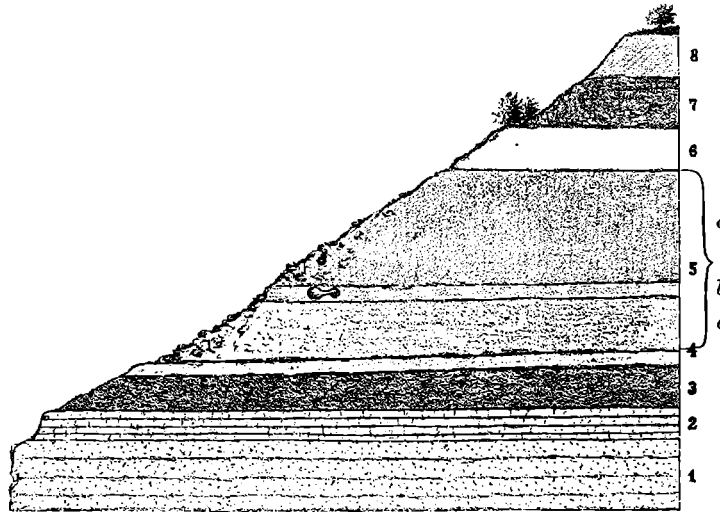
Fig. 10. Profil der Anhöhe „Lehmbrüche“ zwischen Laun und Mainz.
