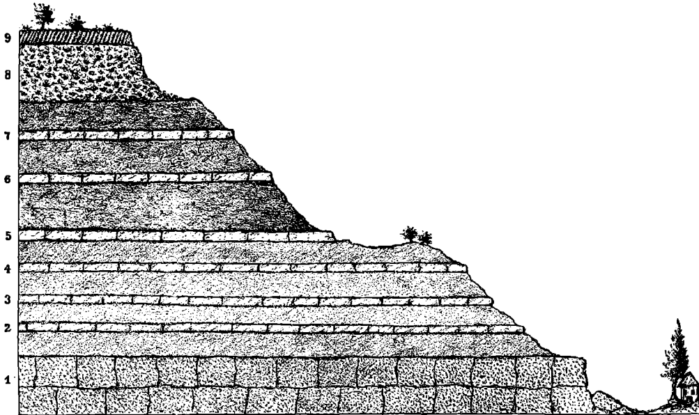
Fig. 11. Profil bei der Podhrazmühle nördlich von Slavětín (unweit Laun).
