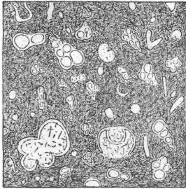
Fig. 6. Schliff der Eisenschichte Nro. 16. des Settenser Profils. Vergr. 50mal. Die graue Masse bei stärkerer Vergrösserung aus lauter Globigerinen u. Textillarien bestehend.
