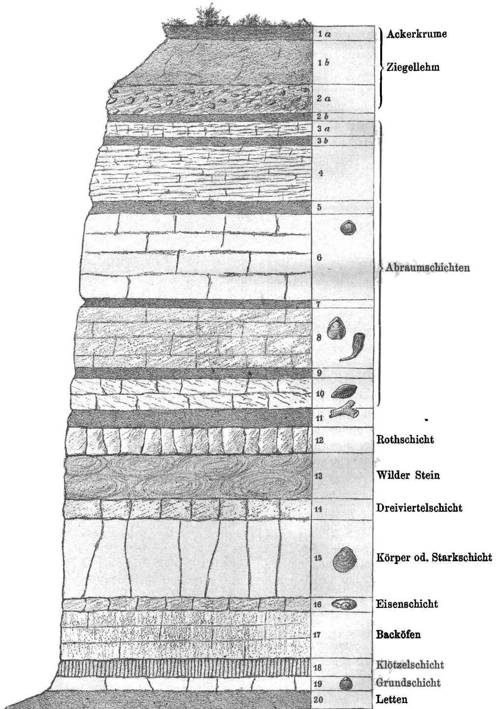
Fig. 3. Profil der Teplitzer Schichten im Pickhardt's Steinbruche bei Setz mit einer versuchsweisen Andeutung der in den einzelnen Schichten vorwaltenden Versteinerungen. Aufgenommen 13. August 1884.
