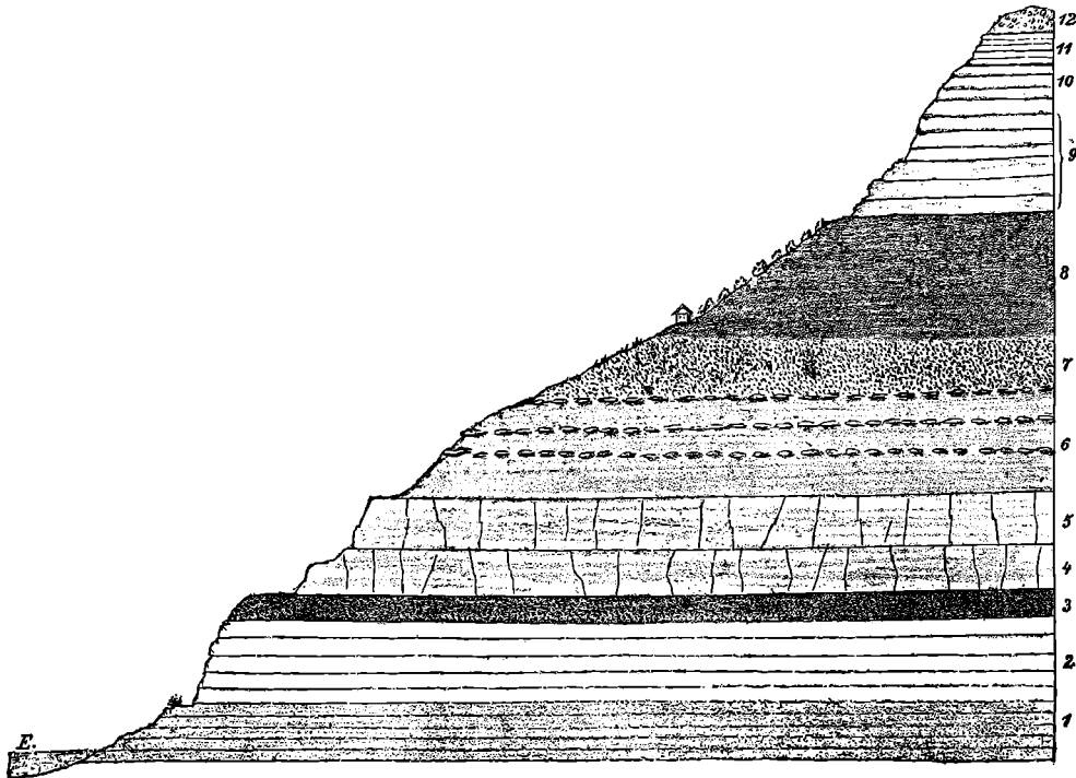
Fig. 15. Schematisches Profil des Sovice-Berges bei Brozáněk nordöstlich von Raudnitz.
