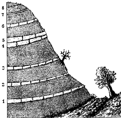
Fig. 14. Profil der oberen Hälfte der Teplitzer Schichten am Bache östlich im Dorfe Popelz bei Libochovic.
