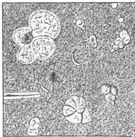
Fig. 7. Schliff der Grundschieht Nro. 19. des Settenser Profils. Vergr. 50mal.
