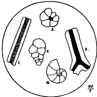
Fig. 1. Schliffprobe der scharfen Schichte von Leneschitz. 1. Spongien-Nadel (Geodia). 2. Hexactinellide. 3. Globigerina. 4. Textillaria. 5. Crustellaria.
