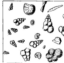
Fig. 4. Schlemmprobe der Schichte Nro. 5. des Settenzer Profils. Vergr. 50mal.
