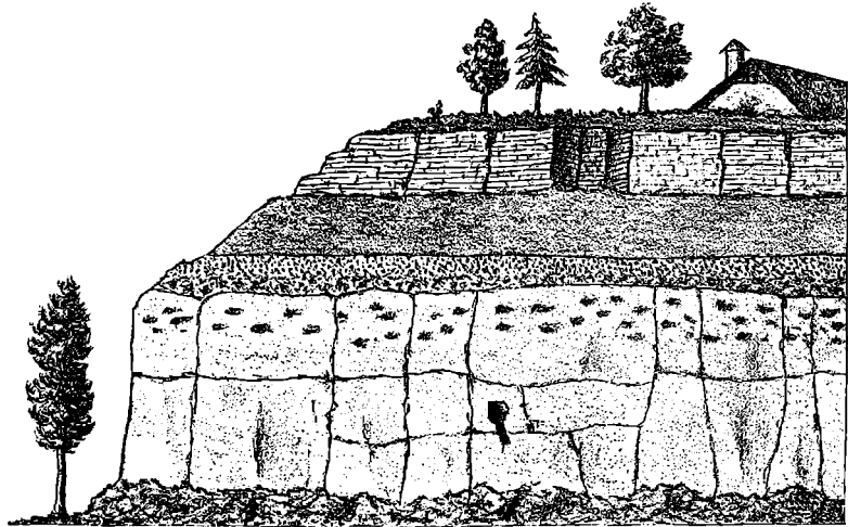
Fig. 19. Profil im Steinbruche hinter dem Hause Nro. 248 in Abtsdorf.
