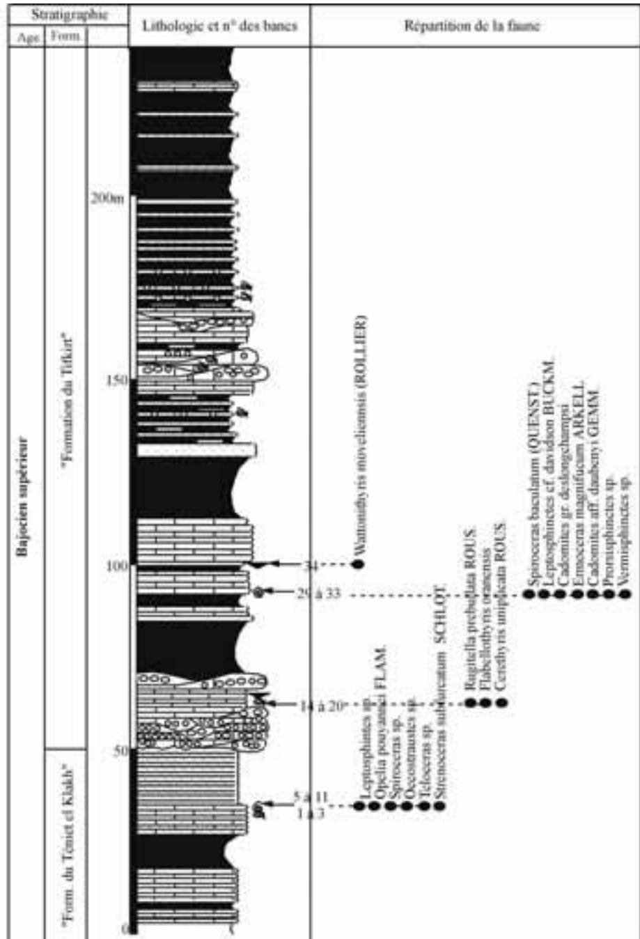
Répartition biostratigraphique des brachiopodes et des ammonites du Bajocien supérieur du Djebel Zerga de Sfisifa (Mekahli, 1989, inédit). 1 ammonites ; 2 bellerophontes ; 3 brachiopodes ; 4 biostratification ; 5 bivalves ; 6 brachiopodes ; 7 crinoïdes ; 8 débris de végétaux ; 9 entroques ; 10 fongues ; 11 madréporaires ; 12 oolithes ; 13 rhizocorallium ; 14 ripple marks ; 15 slumps ; 16 calcaires ; 17 dolomites ; 18 grès ; 19 marnes ; 20 silt et argiles.
