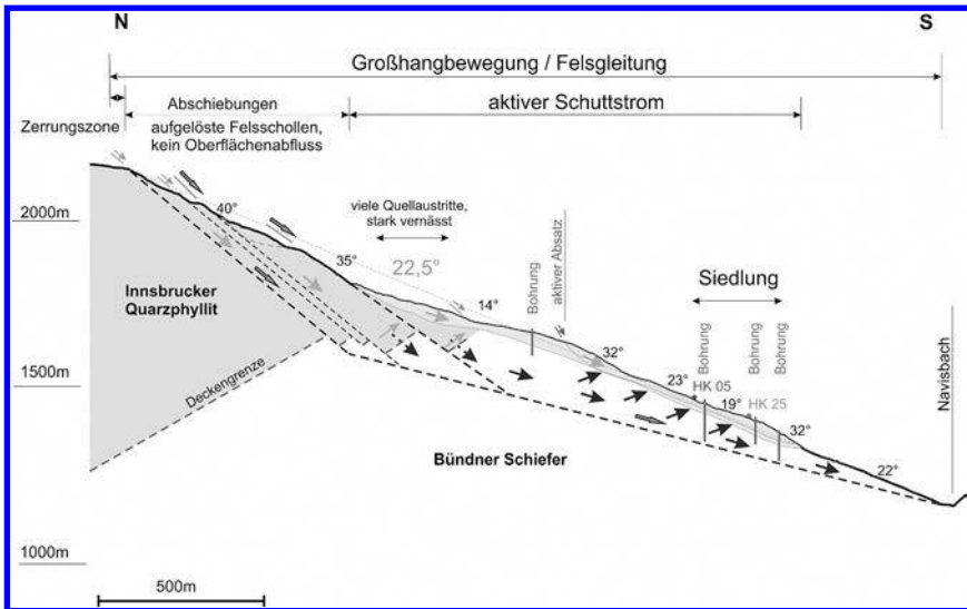
Abbildung 04: Ingenieurgeologischer Profilschnitt durch die Großhangbewegung Misjoch. Figure 04: Engineering geological section through the large-scale landslide Misjoch. Quelle: mod. nach Hofmann und Sausgruber, 2017
