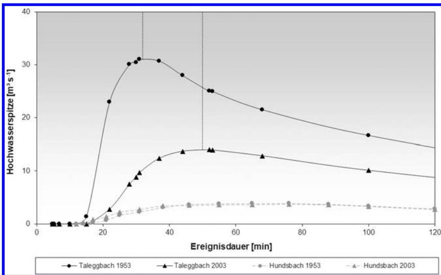
Abbildung 03: Geänderte Hochwasserspitzen bei Niederschlägen unterschiedlicher Dauer in den Einzugsgebieten Hundsbach und Taleggbach (Teileinzugsgebiete des Finsingbaches – nördlichstes rechtsufriges Seitental des Zillertales in Tirol) nach flächenwirtschaftlichen Maßnahmen (Integralmelioration).
