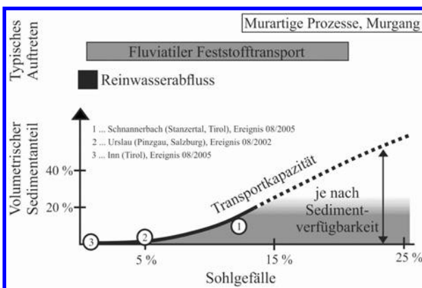
Abbildung 01: Schematische Darstellung zum typischen Auftreten von Verlagerungsprozessen in Gewässern in Abhängigkeit von Sohlneigung und Sedimentverfügbarkeit; Zuordnung der in Kapitel 12.4 beschriebenen Extremereignisse.
