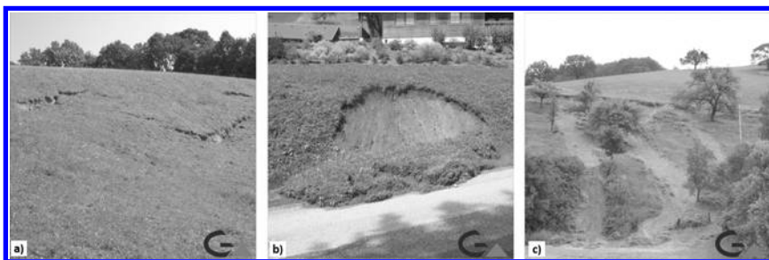
Abbildung 01: Spontan entstandene und entwickelte Prozesse unterschiedlicher Typen und/ oder Entwicklungsstadien in der Region »Klingfurth (NÖ)« in Juni 2009: Anriss/ initiale Rutschung (a), Translationsrutschung (b) und Lockergesteinsrutschungen (Initialprozess) die in Hangmuren übergehen können (Sekundärprozess).
