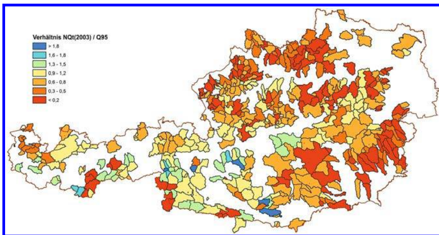
Abbildung 11: Niederwasserdurchfluss des Jahres 2003 ( NQ_1 ) in Bezug zu Q_{95} (325 Zwischen-EG, 1977–1996).
