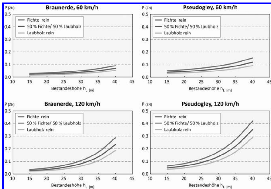
Abbildung 07: Wahrscheinlichkeit einer Zufallsnutzung ( P_{ZN} ) in Abhängigkeit von der Bestandesmittelhöhe, Windgeschwindigkeit, Boden- und Bestandestyp.
