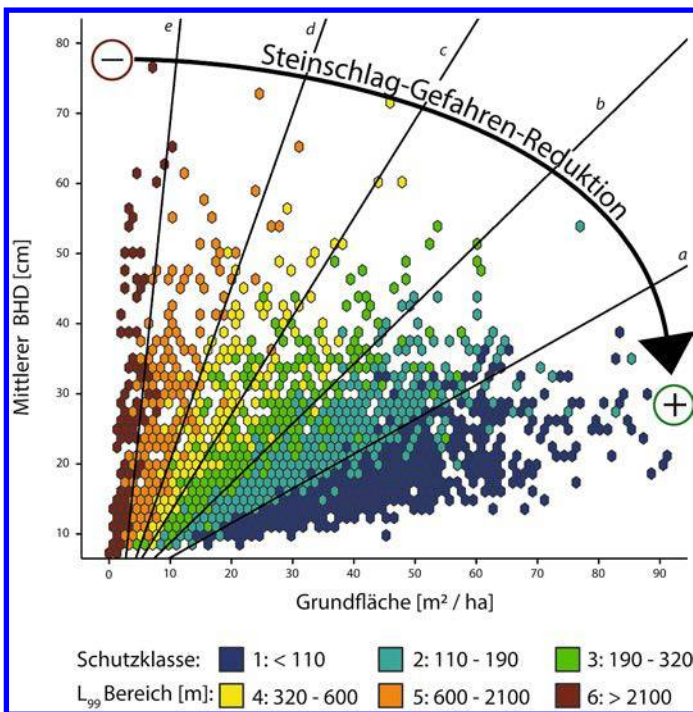
Abbildung 05: Einfluss der Verteilung von Grundfläche und BHD auf die Reduktion der Steinschlaggefahr.
