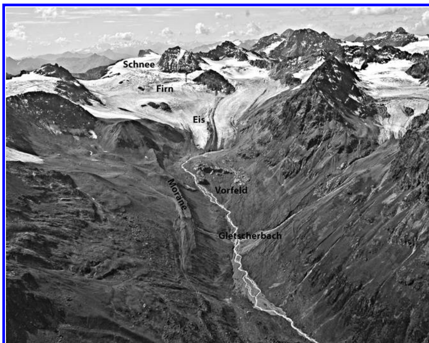
Abbildung 01: Beispiel eines Alpengletschers (Jamtalferner/Silvretta) und seiner Teilzonen sowie den typischen morphologischen Formen.
