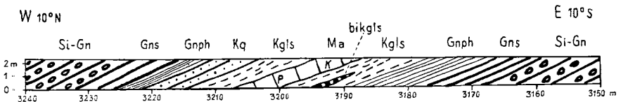
Abb. 2. Profil der metamorphen Kalklage im Siglitz-Gneis.
