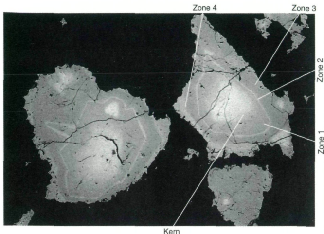
Abb. 3: Deutlich zonierte Fahlerzkristalle im Quarzit; Neufunkenstein, Grabanz, Mallesberger Mittagskogel, Karawanken, Kärnten. REM-Foto: BSE-Bild, Institut für Mineralogie-Kristallographie und Petrologie, Karl-Franzens-Universität Graz. Bildbreite: 0,9 mm.
