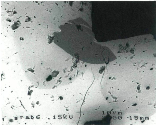
Abb. 8: Siegenit im deutlich zonierten Fahlerz; Neufinkenstein, Grabanz, Mallestiger Mittagskogel, Karawanken, Kärnten. REM-Foto: BSE-Bild, Institut für Mineralogie-Kristallographie und Petrologie, Karl-Franzens-Universität Graz. Bildbreite: 0,14 mm.
