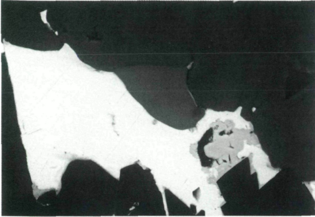
Abb. 7: Fahlerz (grau) mit Galenit, der teilweise in Anglesit (hellgrau) umgewandelt ist und Carbonaten im Quarzit/Sandstein; Neufinkenstein, Grabanz, Mallestiger Mittagskogel, Karawanken, Kärnten. REM-Foto: BSE-Bild, Institut für Mineralogie-Kristallographie und Petrologie, Karl-Franzens-Universität Graz. Bildbreite: 0,08 mm.
