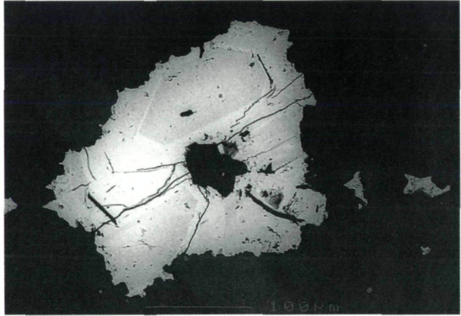
Abb. 4: Tennantit-reicher, idiomorpher Fahlerzkristall von As-ärmerem Fahlerz umwachsen; Neufunkenstein, Grabanz, Mallestiger Mittagkogel, Karawanken, Kärnten. REM-Foto: BSE-Bild, Institut für Mineralogie-Kristallographie und Petrologie, Karl-Franzens-Universität Graz. Bildbreite: 0,5 mm.
