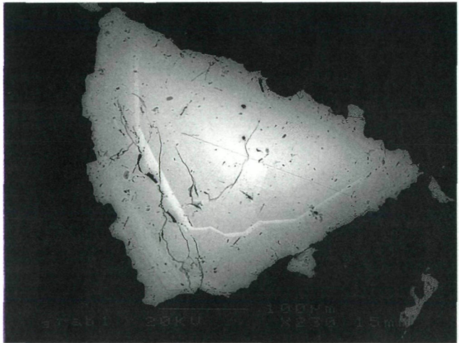
Abb. 6: Zonierter Fahlerzkristall mit undeutlich entwickelten Flächen; Neufunkenstein, Grabanz, Mallestiger Mittagkogel, Karawanken, Kärnten. REM-Foto: BSE-Bild, Institut für Mineralogie-Kristallographie und Petrologie, Karl-Franzens-Universität Graz. Bildbreite: 0,6 mm.
