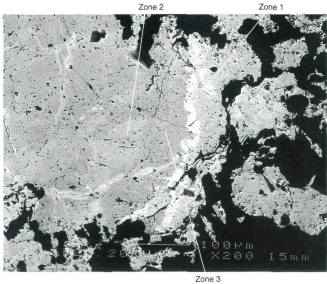
Abb. 5: Mäanderartig gewundenes, Sb-reiches Fahlerz im Sb-ärmeren, deutlich chemisch inhomogenen Fahlerz; Neufunkenstein, Grabanz, Mallestiger Mittagkogel, Karawanken, Kärnten. REM-Foto: BSE-Bild, Institut für Mineralogie-Kristallographie und Petrologie, Karl-Franzens-Universität Graz. Bildbreite: 0,6 mm.
