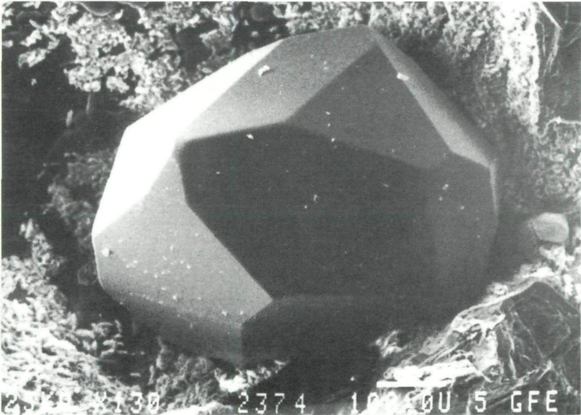
Abb. 2: Nitrobarit, vielflächiger Einzelkristall, REM-Aufnahme, 130fach vergrößert
