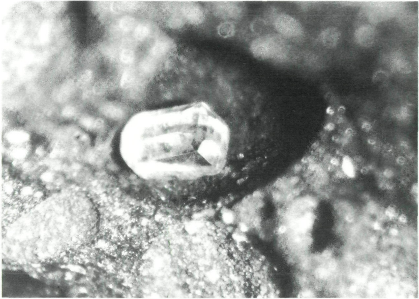
Abb. 1: Nitrobarit, Einzelkristall, Größe 1 mm
