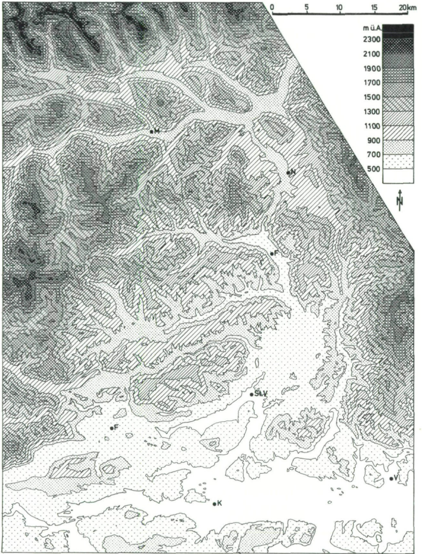
Abb. 1: Höhengschichtenkarte des Mittelkärntner und des Norischen Raumes. Die 200-m-Höhengschichtenkarte zeigt deutlich, wie sich das Klagenfurter Becken als Großraum in einem Halbrund nach Norden bis in das Metnitzgebiet ausbuchtet. Sie zeigt eine großmorphologische Konfiguration in Anlehnung an ein Rumpftreppenmodell. Nach einer W-E gerichteten Schwellenzone, die die alte Wasserscheide zwischen Drau- und Murgebiet darstellt, beginnt der Norische Großraum in einer Art Doppeltalanlage. Seine letzte flächenerhaltende tiefste Erosionsbasis ist die Neumarkter Hochfläche.
