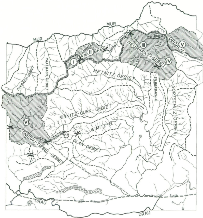
Abb. 2: Die präglazialen Gewässer-Einzugsgebietsregionen Mittelkärntens zwischen Drau und Mur: Strichlierte Linien: Relief-Hauptscheitellinien (Wasserscheiden), wobei mit der strichpunktierter Linie die ältestpleistozäne Drau-Mur-Wasserscheide hervorgehoben ist. – Mit Ringen dargestellte Linie: Der heutige Verlauf der Drau-Mur-Wasserscheide. – Doppelt strichlierte Linie: Vermutlicher Verlauf der präglazialen Drau- und Gurk-Tiebel-Tiefenlinie. I: Gebietsverlust der Mur an das Draugebiet durch die Anzapfung des Röttingbaches. II: Gebietsverlust des Lambrechtbach-Systems (Auenbach-Talbach-Thaya) an die Laßnitz. III: Gebietsverlust der Mur an die Drau durch die Dürnstein-Olsa-Anzapfung des Neumarkter Gebietes. IIIa: Kleiner Gebietsverlust des Doppelbaches (Mur) an den Perchauer Bach (Drau). IV: Gebietsverlust der Mur an die Drau durch die Görttschitz-Anzapfung des Neumarkter Gebietes. V: Gebietsverlust der Drau (Lavant) an die Mur, Anzapfung durch den Granitzenbach. VI: Gebietsverlust des präglazialen Gnesau-Tiebel-Gebietes an das Sirnitz-Gurk-Gebiet. VIa: Kleiner Gebietsverlust des Glan-Gebietes („Enge Gurk“) an das Sirnitz-Gurk-Gebiet. (= Talwasserscheiden.)
