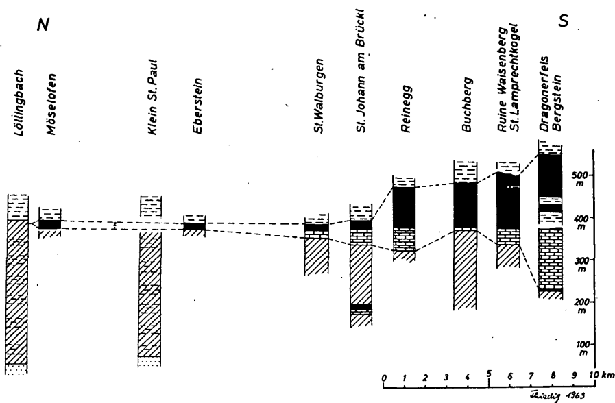
Abb. 3. Die Fazies der epizonalen Karbonatserie am Westrand der Saualpe vom Löllinggraben bis zum Dragonerfels (ca. 28 km).
