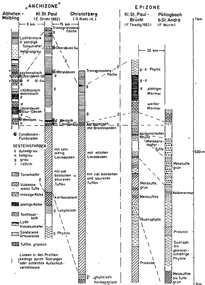
Abb. 2. Säulenprofile der charakteristischen Schichtfolgen aus der Epizone und dem anchimetamorphen Altpaläozoikum.
