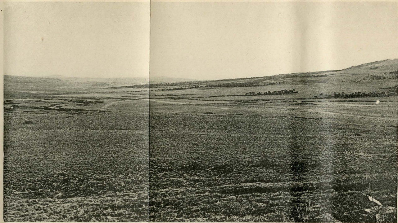
2. Vallée supérieure del Arco vers le sud
