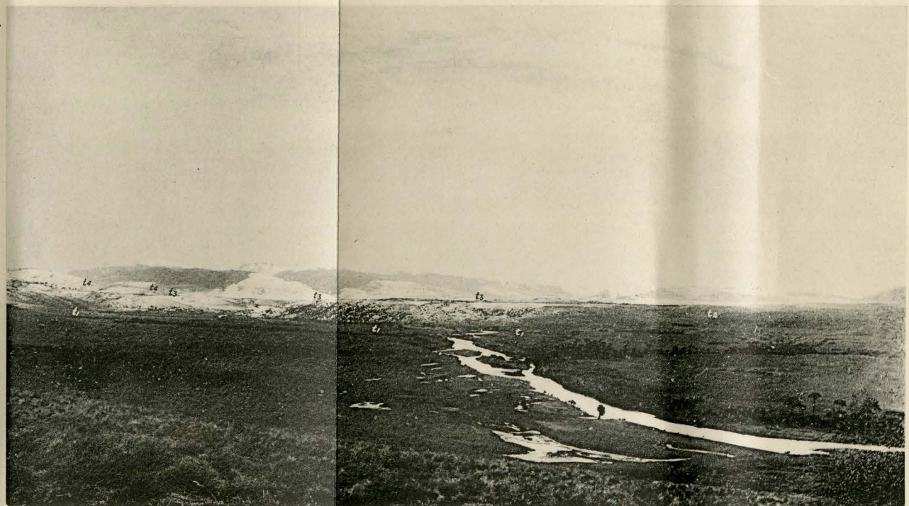
4. Les terrasses d'alluvion du Biobio supérieur t 1 — t 4 = Terrasses
