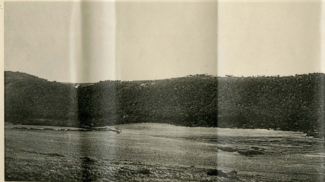
3. Le «Divortium aquarum» actuel au Paso del Arco m → Direction des eaux
