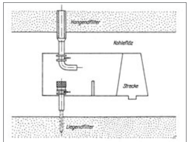
Abb. 5-1-12: Kombiniertes Filter
