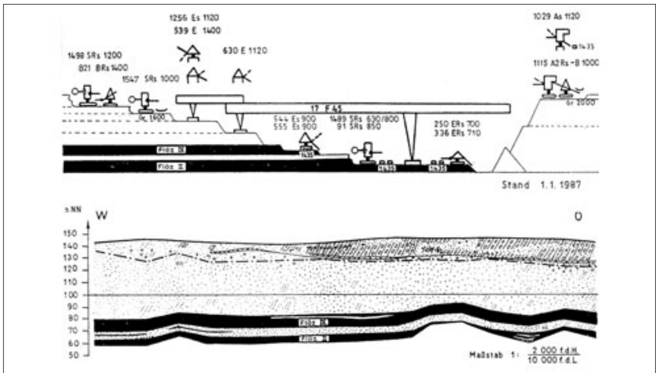
Abb. 5-2-40: Geräteinsatzschema und Lagerstättenbedingungen Brückentagebau Espenhain
