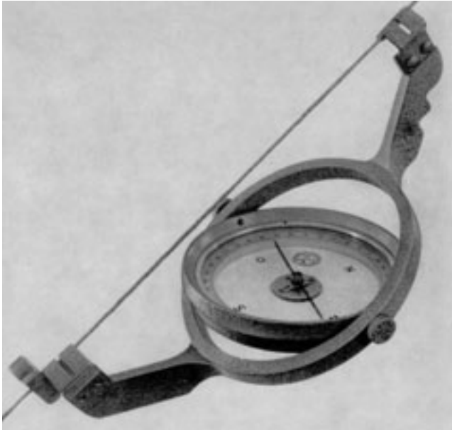
Abb. 7-3-2: Freiburger Hängekompass
