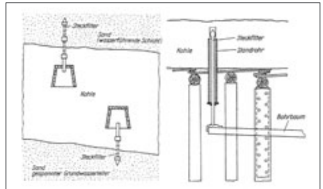
Abb. 5-1-11: Prinzipdarstellung Steckfilter
