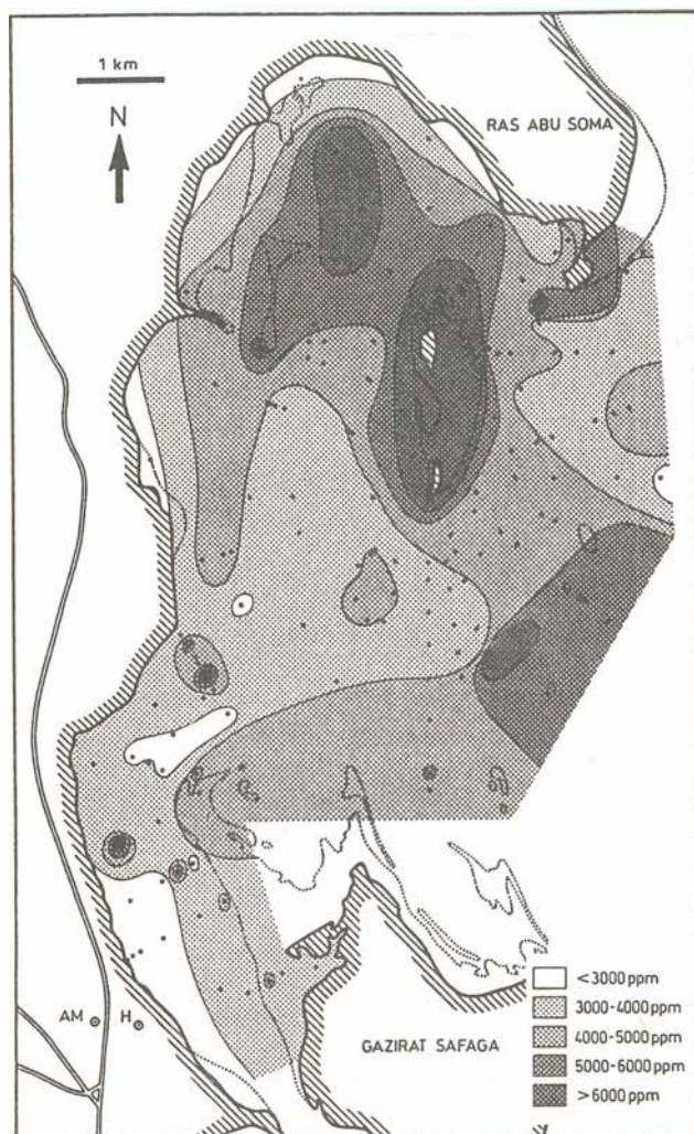
Fig. 48. Distribution of strontium ( \text{Sr}^{++} ).
