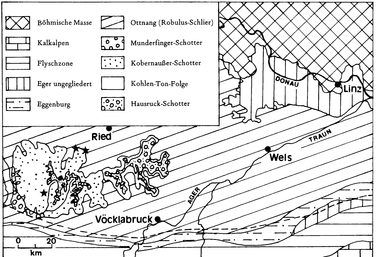
Abb. 4: Geologische Übersichtskarte der Molassezone Oberösterreichs, Verbreitung der limnisch-fluviatilen miozänen Ablagerungen im Hausruck und Kobernauser Wald nach FUCHS (1980) und MACKENBACH (1984).
