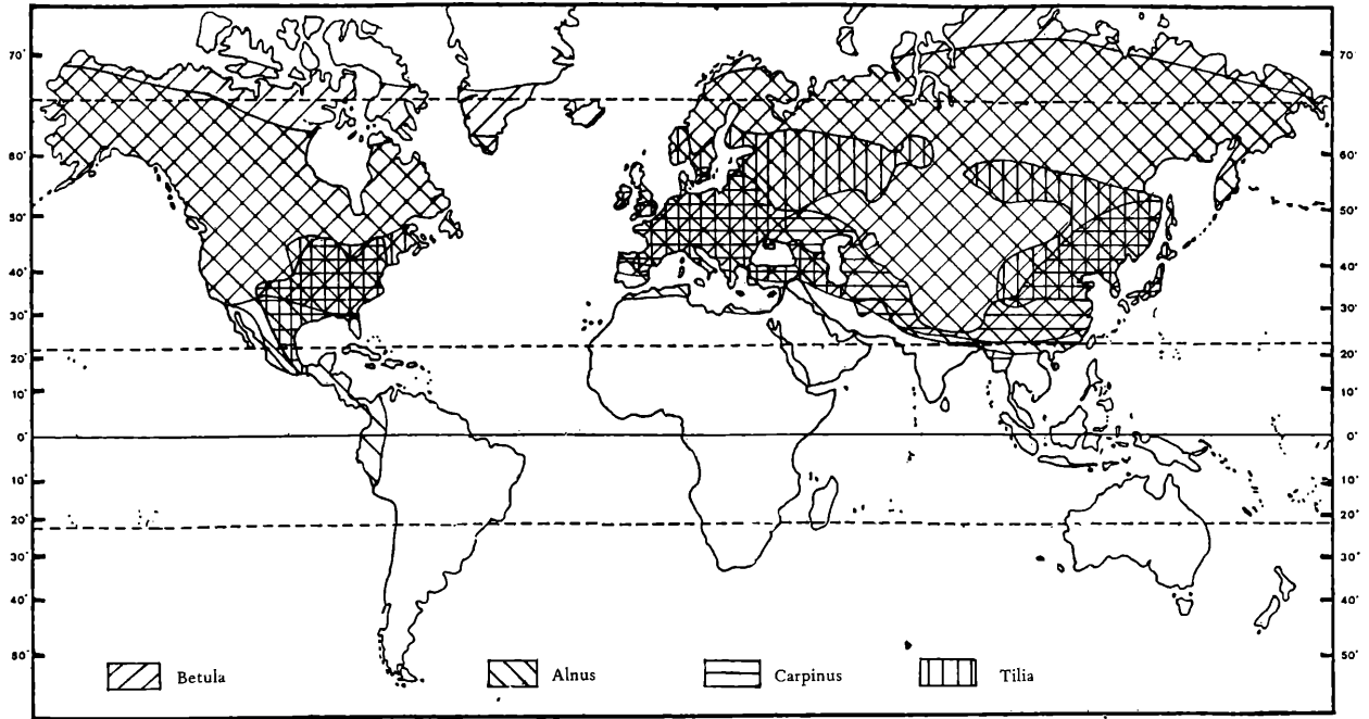
Abb. 8–15: Rezente Verbreitung einiger nachgewiesener Gattungen aus KRÜSSMANN 1976–1978. Abb. 8: Weitgehend gesamt nordhemisphärisch verbreitete Gattungen ( Betula , Alnus , Carpinus , Tilia ).
