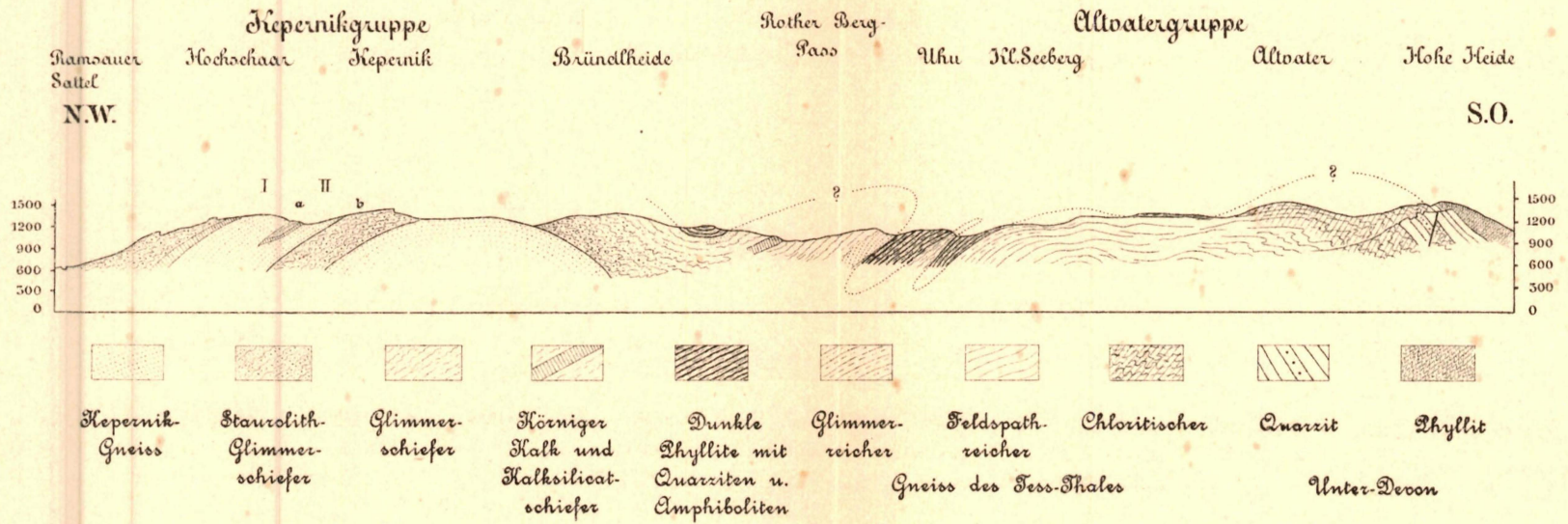
Profil des Hohen Gesenkes 1:100.000
