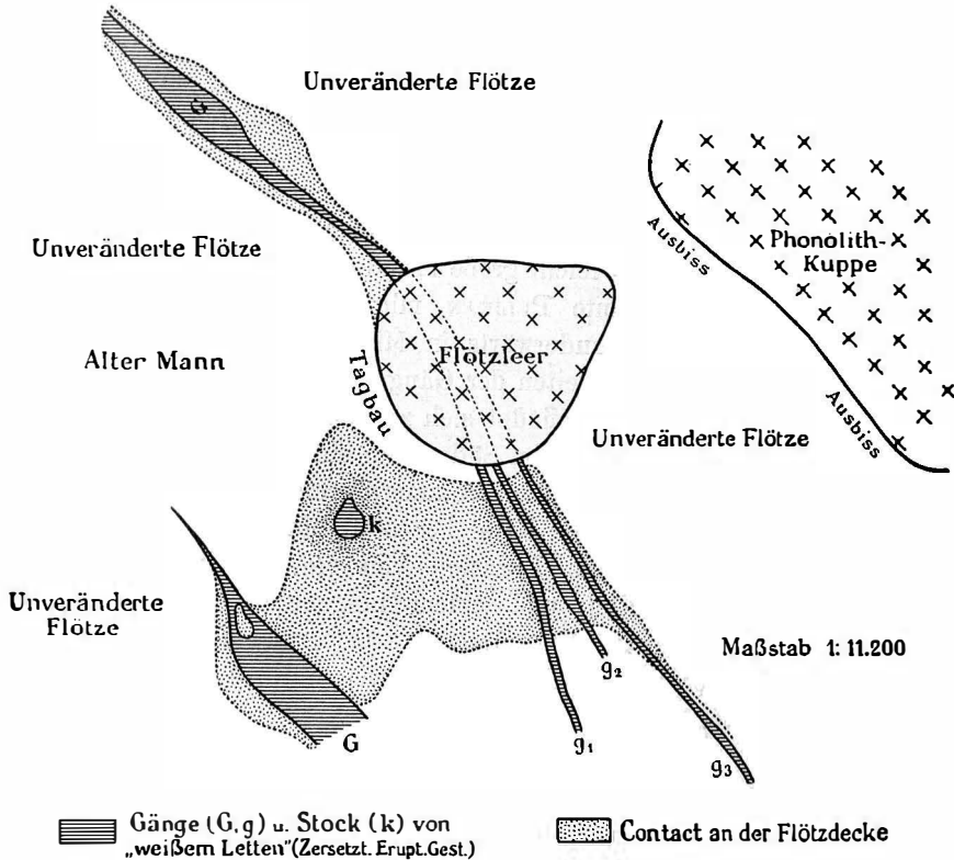
Fig. 46. Trachytgänge und Verkokung der Braunkohle in der Emeranzee bei Bilin, nach PELIKAN.
