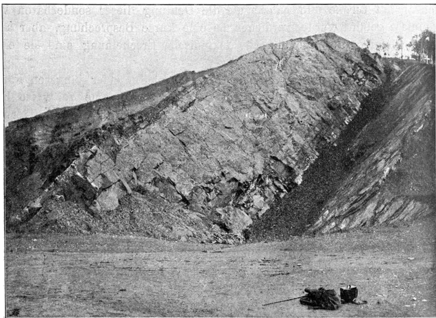
Fig. 29. Lagergang von Diabas im Graptolithenschiefer. Kolonie Hodkowiczka südlich von Prag.
