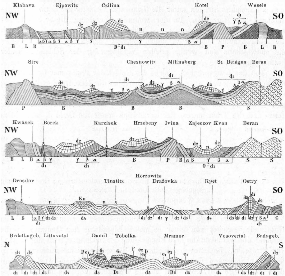
Fig. 20—24. Profile durch den südwestlichen Teil der mittelböhmisches Silurmulse nach KREJČI und K. FEISTMANTEL, von Südwest gegen Nordost aneinander gereiht.
