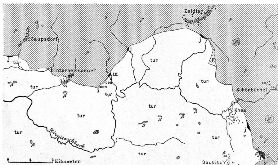
Fig. 51. Die Bucht von Zeidler. Überschiebung des Granits über Jura und Kreide. tur Turon, cen Cenoman, j Jura, P Rotliegendes, γ Granit, β Basalt, I, IX Untersuchungs-Stollen.
