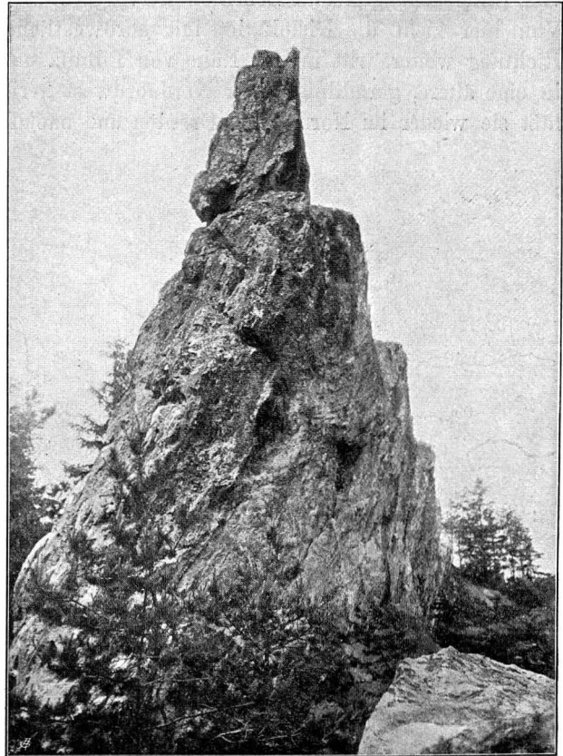
Fig. 50. Steilgestellter Schichtenkopf des Kreidesandsteines am Kamme des Trögelsberges bei Pankratz.
