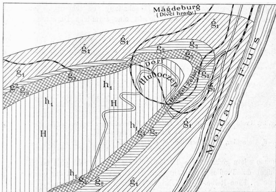
Fig. 27. Muldenförmige Lagerung der Devonschichten bei Hluboczeper nach BARRANDE.
