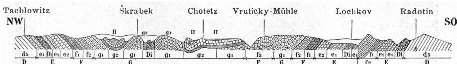
Fig 31. Profil durch das Kalkgebiet im Radotiner Tale nach KREJČÍ und FEISTMANTEL.
