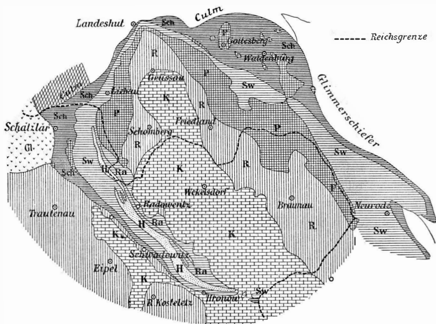
Fig. 53. Das niederschlesisch-böhmische Steinkohlenbecken nach A. WEITHOFER.
