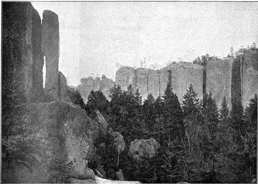
Fig. 39. Senkrechte Klüftung im Quadersandstein. Weckelsdorf.
