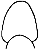
Figur 3. Querschnitt des kleinen Exemplars (Taf. III, Fig. 4) von Perisphinctes mombassanus nov. sp. Ober-Oxford, Mombassa.
