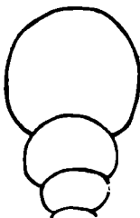
Figur 6. Querschnitt zu Perisphinctes africanus nov. sp. (Taf. III, Fig. 2). Ober-Oxford, Mombassa.
