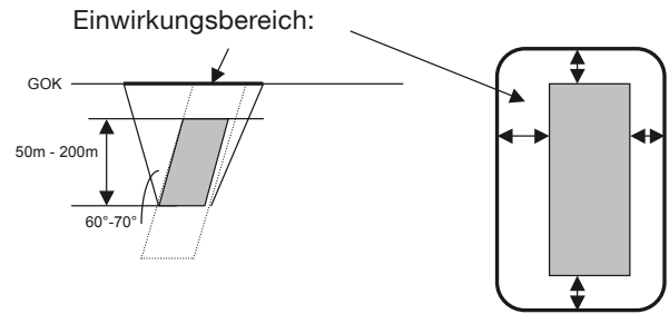
Abb. 178. Untertagebau bei oberflächennahen Lagerstätten: Beispiel des Einwirkungs- bereichs für gangförmige Lagerstätten.
