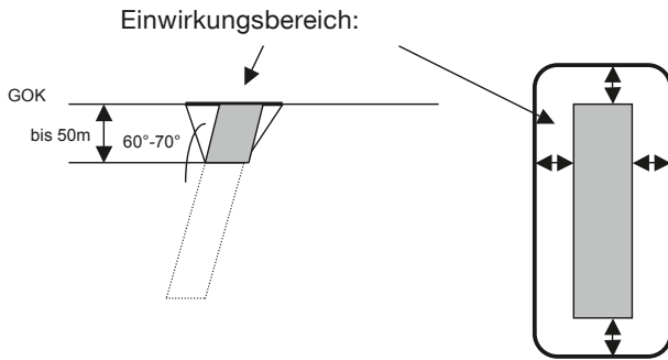
Abb. 176. Untertagebau bei tagesnahen Lagerstätten: Beispiel des Einwirkungs- bereichs für gangförmige Lagerstätten. Fig. 176. Underground Mining of Surface Near Deposits: Example of Sphere of Influence for Vein-like Deposits.
