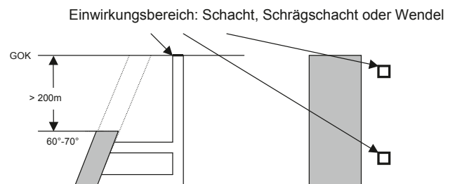
Abb. 179. Untertagebau bei Lagerstätten im tieferen Untergrund: Beispiel des Einwirkungs- bereichs.
