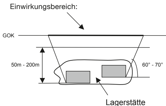
Abb. 177. Untertagebau bei oberflächennahen Lagerstätten: Beispiel des Einwirkungs- bereichs für unregelmäßige Lagerstätten. Fig. 177. Underground Mining of Low Depth Deposits: Example of Sphere of Influence for Irregular Deposits.
