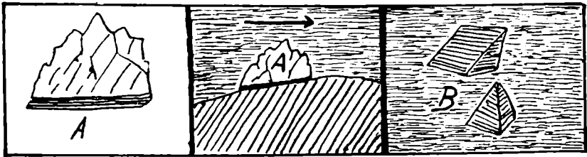
Fig. 15. Nicht vorkommende Geschiebeformen.
