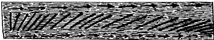
Fig. 2. Hineindrehen eines Querlings in die Achse des Treibstroms.
