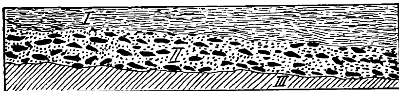
Fig. 6. Einschaltung von Grundmoräne zwischen Eis und Felssohle. I Eis, II Grundmoräne, III Felssohle.
