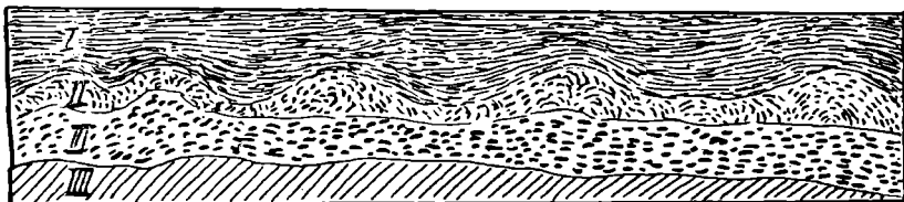
Fig. 7. Einschaltung einer Schlierenzone. I Eisströmung, II Schlierenbildung, III Grundmoräne, IV Felssohle.
