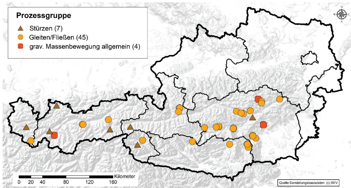
Abb. 3: Räumliche Verteilung der für Juli 2024 mittels Recherchen in Online-Medien erfassten gravitativen Massenbewegungen unterschiedlicher Prozessgruppen (in Klammern die jeweilige Gesamtanzahl) (Anmerkung: Die Anzahl der Ereignisse wird vom gewählten Maßstab nicht korrekt wiedergegeben).
