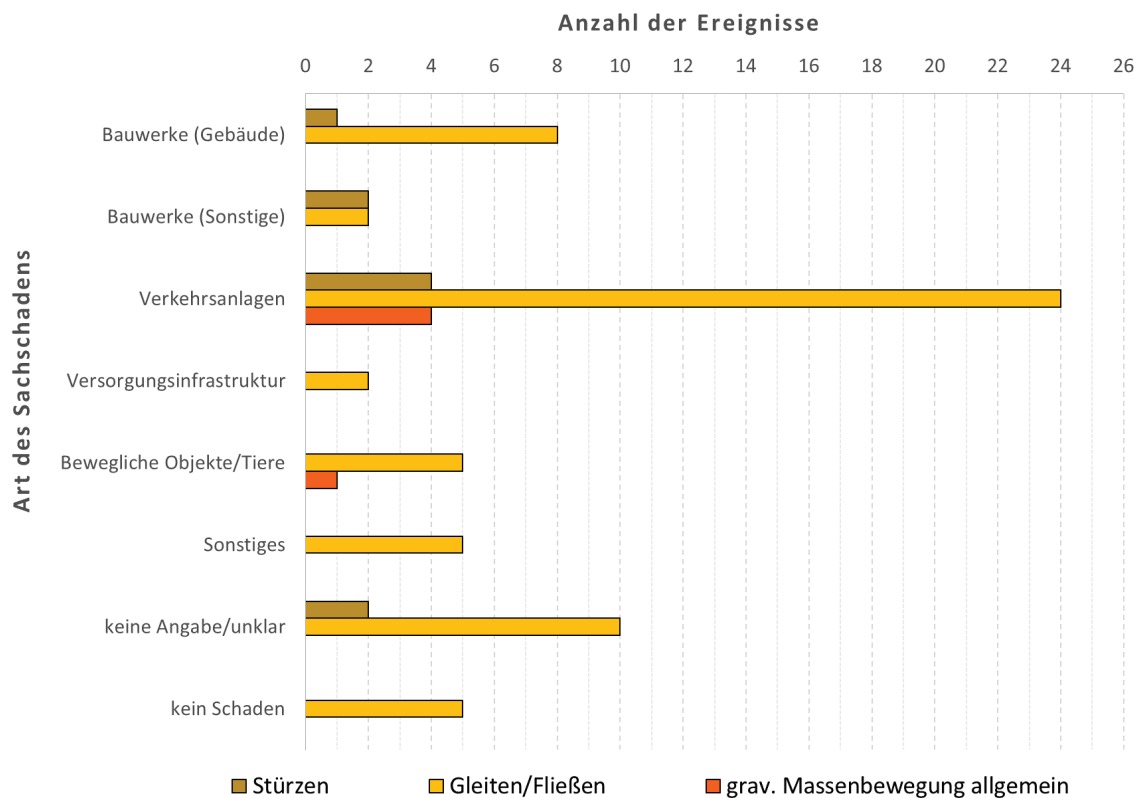
Abb. 5: Überblick zu den mit gravitativen Massenbewegungen im Juli 2024 einhergegangenen Arten von Sachschäden (Achtung: Mehrfachnennungen möglich, weil bei einem Ereignis mehrere Sachschadensarten auftreten können!). Datenbasis: Recherchen der GeoSphere Austria) in Online-Medien.
