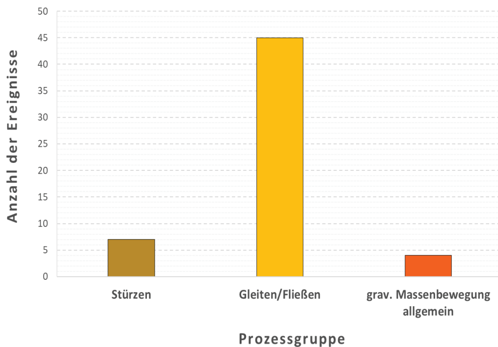
Abb. 1: Mittels Recherchen in Online-Medien erfasste gravitative Massenbewegungen im Juli 2024, differenziert nach Prozessgruppen.
