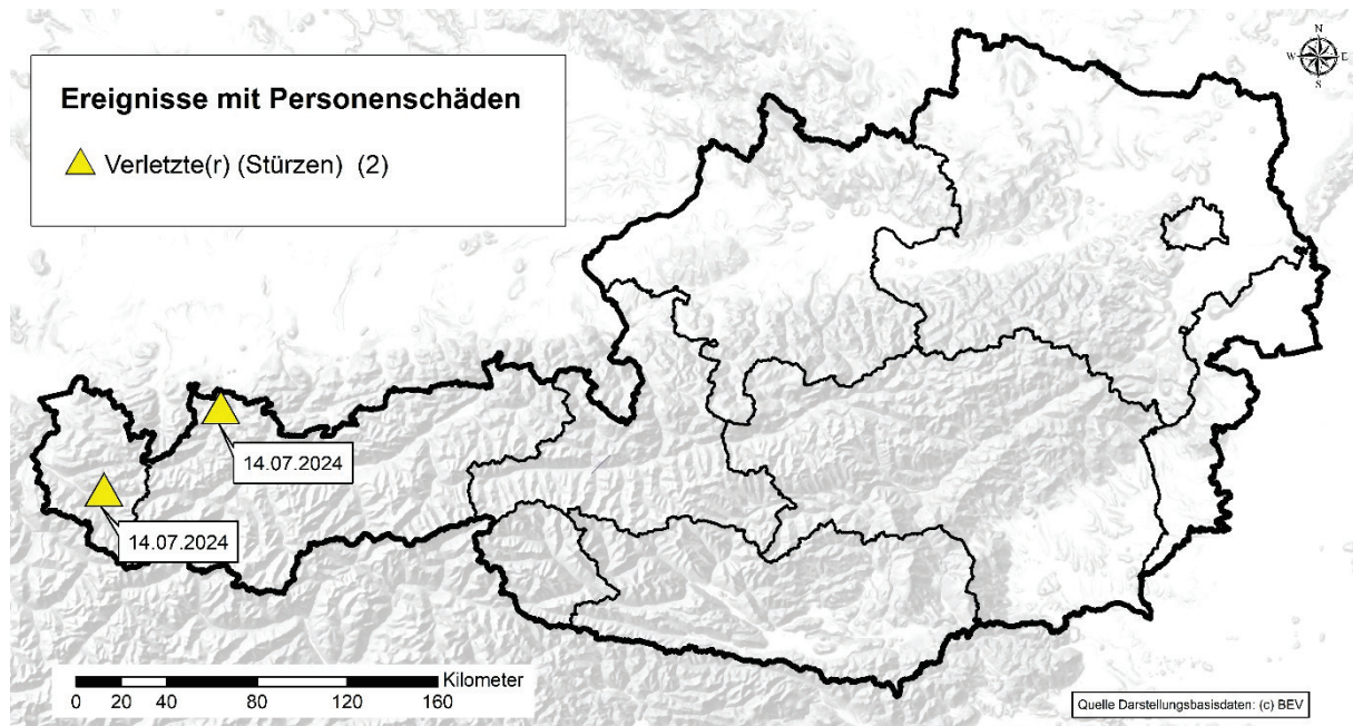
Abb. 4: Räumliche Verteilung der mittels Recherchen in Online-Medien im Juli 2024 erfassten gravitativen Massenbewegungen mit Toten oder Verletzten, differenziert nach Prozessgruppen (in Klammern die jeweilige Anzahl der Ereignisse).
