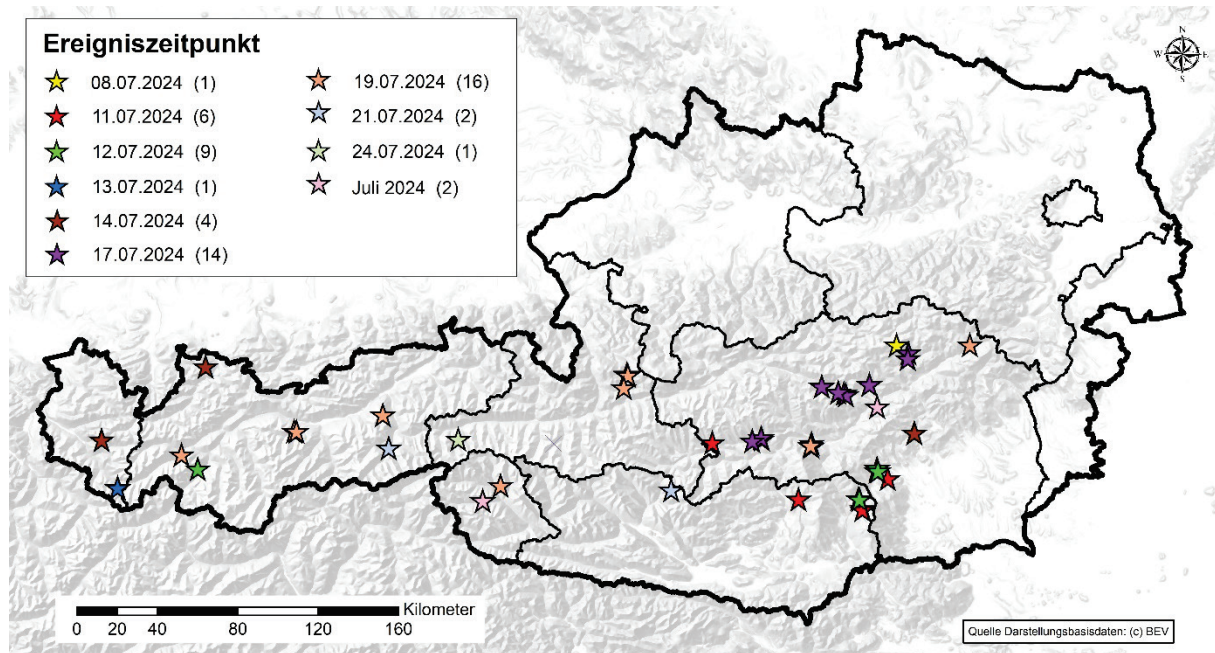
Abb. 6: Räumliche und zeitliche Verteilung der mittels Recherchen in Online-Medien erfassten gravitativen Massenbewegungen in Österreich im Juli 2024 (in Klammern die Anzahl der Ereignisse) (Anmerkung: Die Anzahl der Ereignisse wird vom gewählten Maßstab nicht korrekt wiedergegeben).
