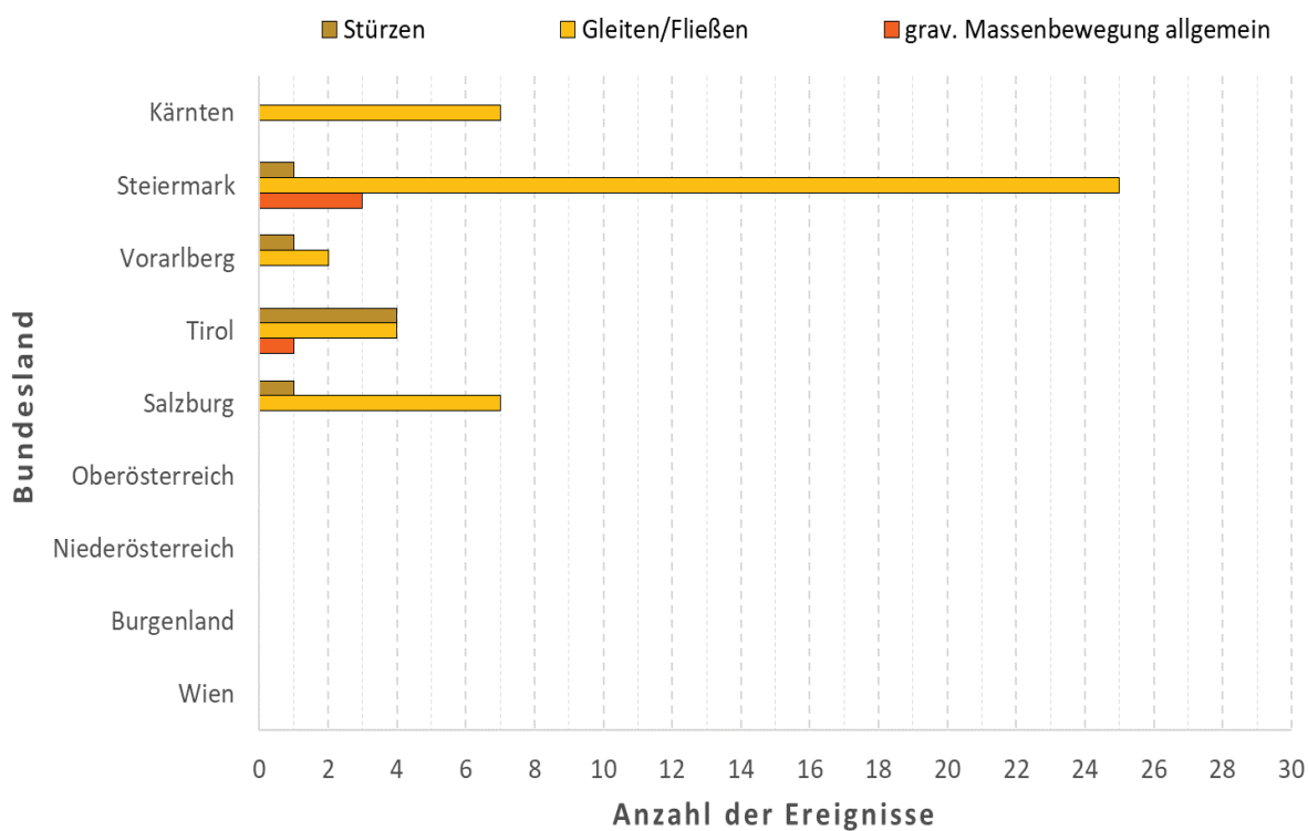
Abb. 2: Mittels Recherchen in Online-Medien für Juli 2024 erfasste gravitative Massenbewegungen, differenziert nach Bundesländern und Prozessgruppen.
