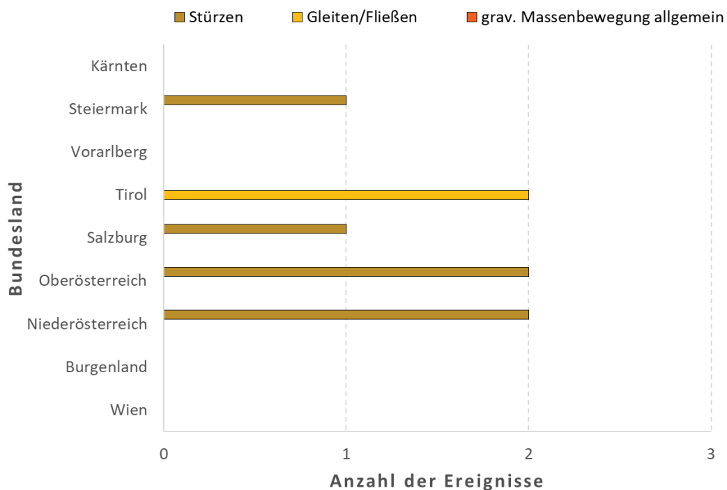
Abb. 2: Mittels Recherchen in Online-Medien für April 2024 erfasste gravitative Massenbewegungen, differenziert nach Bundesländern und Prozessgruppen.
