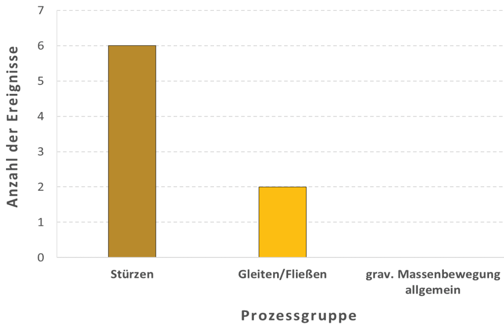
Abb. 1: Mittels Recherchen in Online-Medien erfasste gravitative Massenbewegungen im April 2024, differenziert nach Prozessgruppen.
