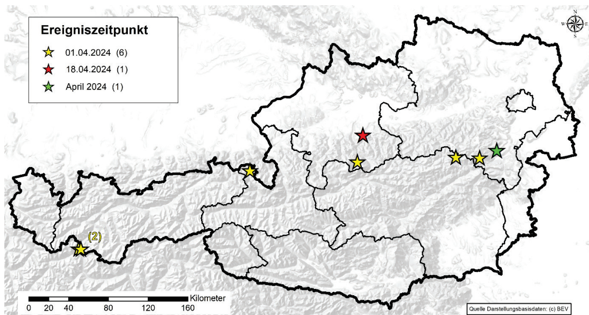
Abb. 5: Räumliche und zeitliche Verteilung der mittels Recherchen in Online-Medien erfassten gravitativen Massenbewegungen in Österreich im April 2024 (in Klammern die Anzahl der Ereignisse).
