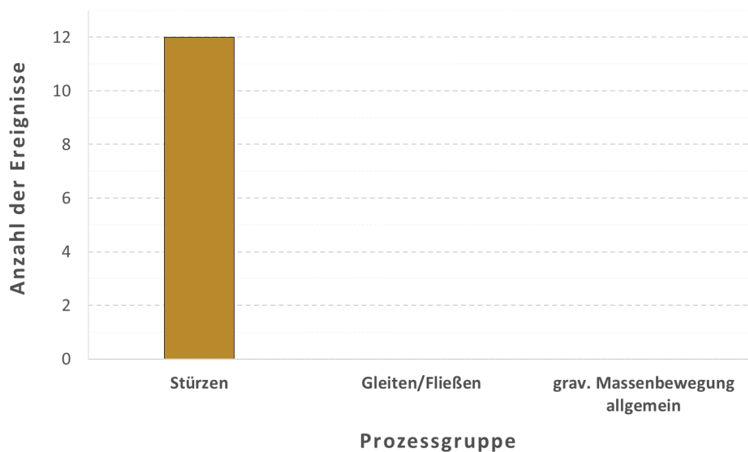
Abb. 1: Mittels Recherchen in Online-Medien erfasste gravitative Massenbewegungen im Februar 2024, differenziert nach Prozessgruppen.
