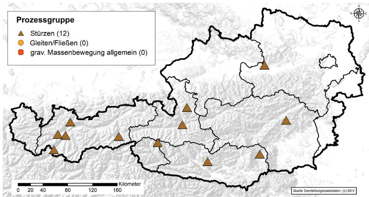
Abb. 3: Räumliche Verteilung der für Februar 2024 mittels Recherchen in Online-Medien erfassten gravitativen Massenbewegungen unterschiedlicher Prozessgruppen (in Klammern die jeweilige Gesamtanzahl).
