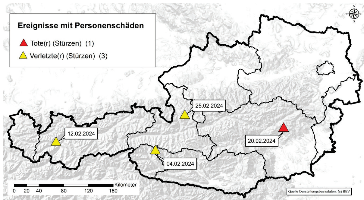
Abb. 4: Räumliche Verteilung der mittels Recherchen in Online-Medien im Februar 2024 erfassten gravitativen Massenbewegungen mit Toten oder Verletzten, differenziert nach Prozessgruppen (in Klammern die jeweilige Anzahl der Ereignisse).
