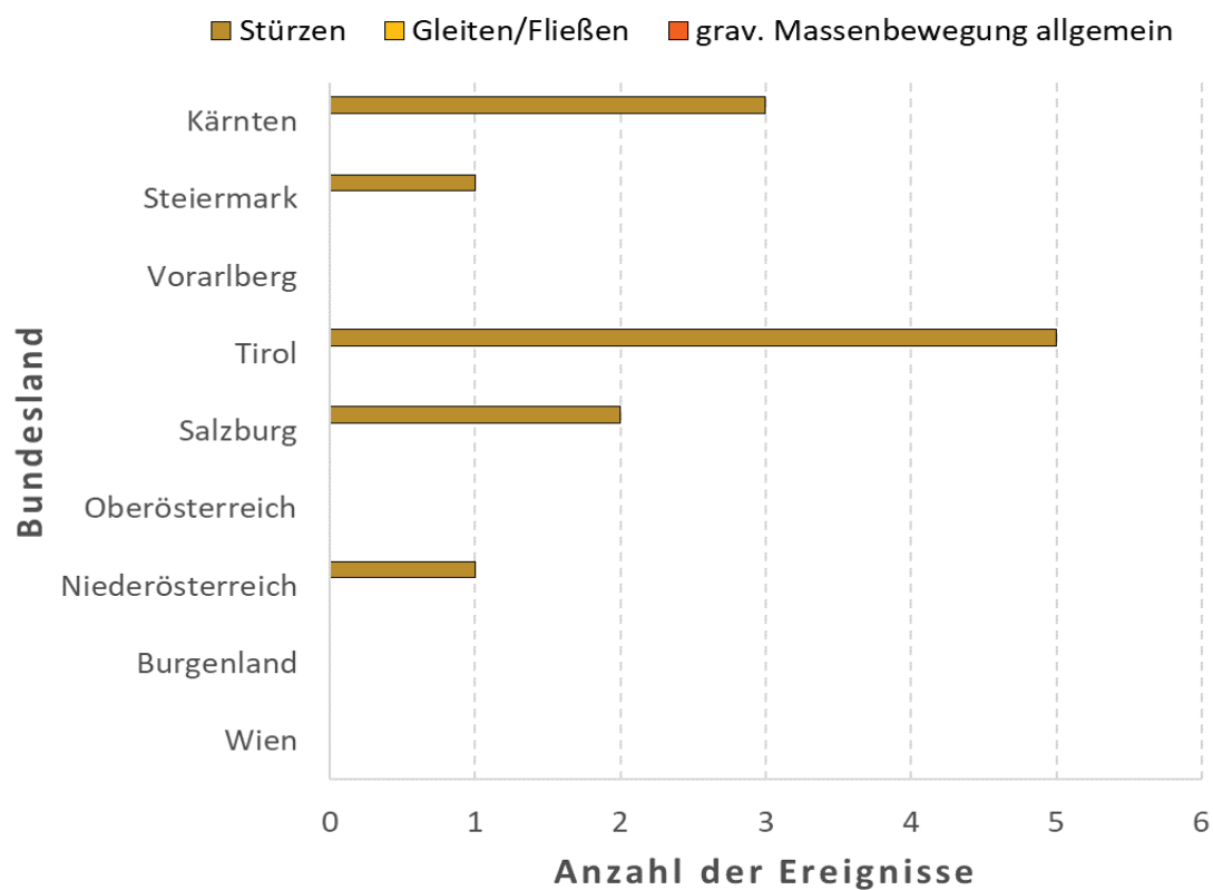
Abb. 2: Mittels Recherchen in Online-Medien für Februar 2024 erfasste gravitative Massenbewegungen, differenziert nach Bundesländern und Prozessgruppen.
