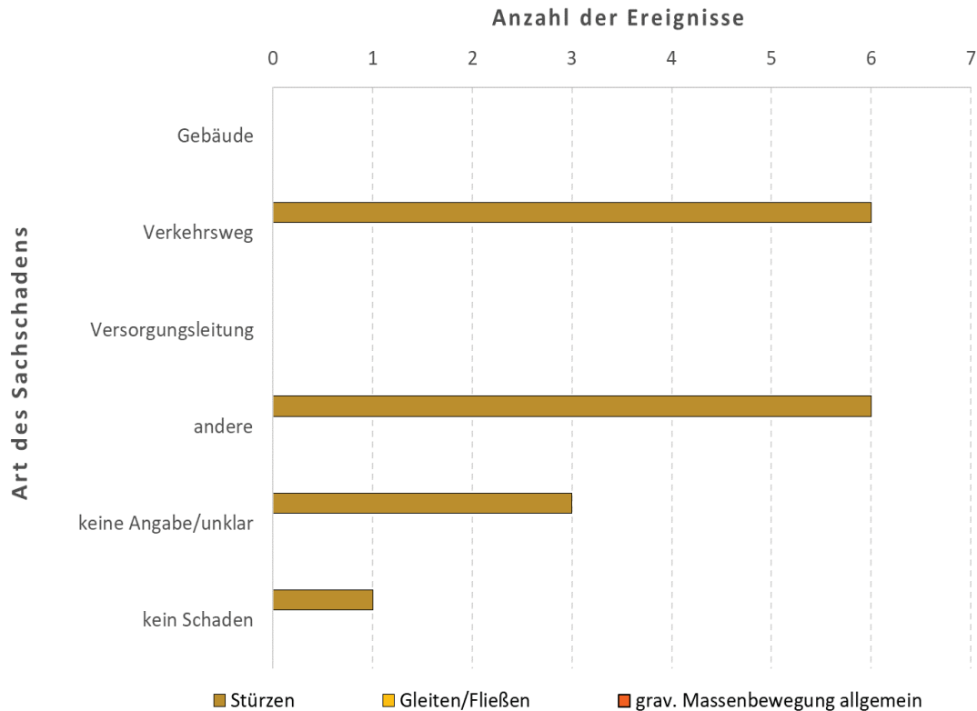
Abb. 5: Überblick zu den mit gravitativen Massenbewegungen im Februar 2024 einhergegangenen Arten von Sachschäden (Achtung: Mehrfachnennungen möglich, weil bei einem Ereignis mehrere Sachschadensarten auftreten können!). Datenbasis: Recherchen der GeoSphere Austria) in Online-Medien.
