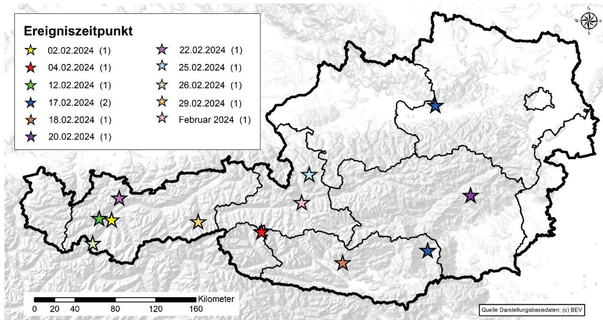
Abb. 6: Räumliche und zeitliche Verteilung der mittels Recherchen in Online-Medien erfassten gravitativen Massenbewegungen in Österreich im Februar 2024 (in Klammern die Anzahl der Ereignisse) (Anmerkung: Die Anzahl der Ereignisse wird vom gewählten Maßstab nicht korrekt wiedergegeben).
