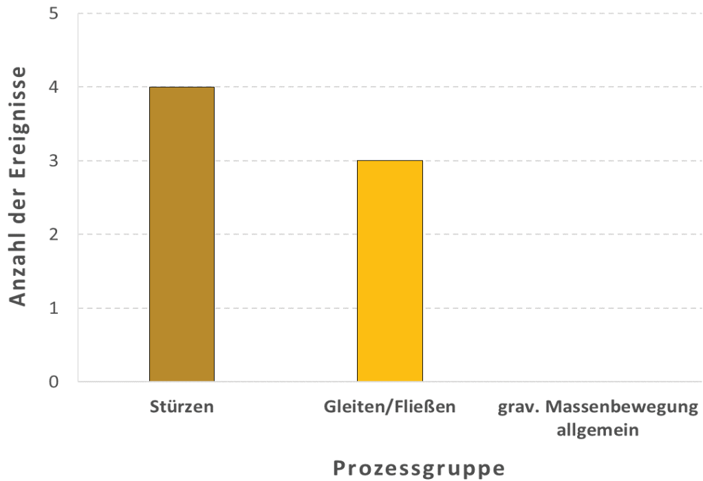
Abb. 1: Mittels Recherchen in Online-Medien erfasste gravitative Massenbewegungen im Jänner 2024, differenziert nach Prozessgruppen.
