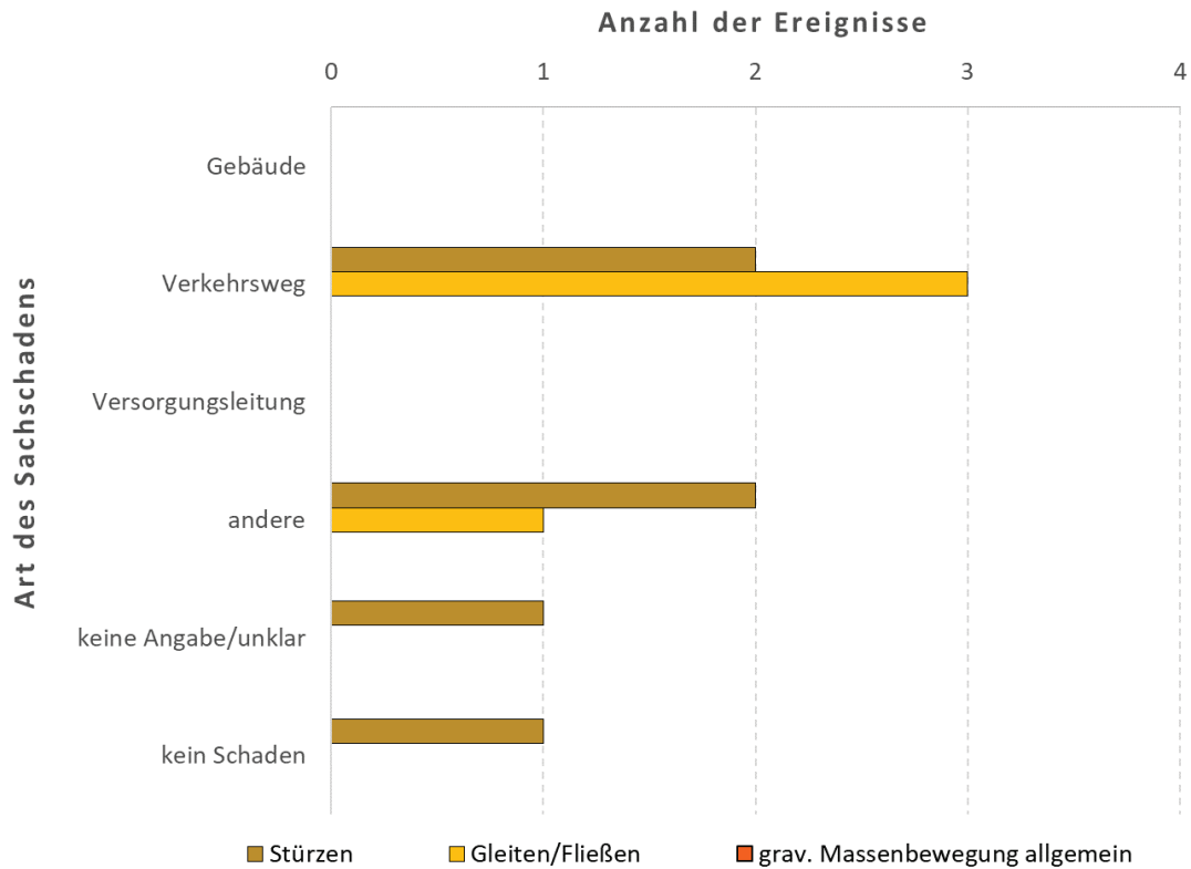
Abb. 4: Überblick zu den mit gravitativen Massenbewegungen im Jänner 2024 einhergegangenen Arten von Sachschäden (Achtung: Mehrfachnennungen möglich, weil bei einem Ereignis mehrere Sachschadensarten auftreten können!). Datenbasis: Recherchen der GeoSphere Austria) in Online-Medien.
