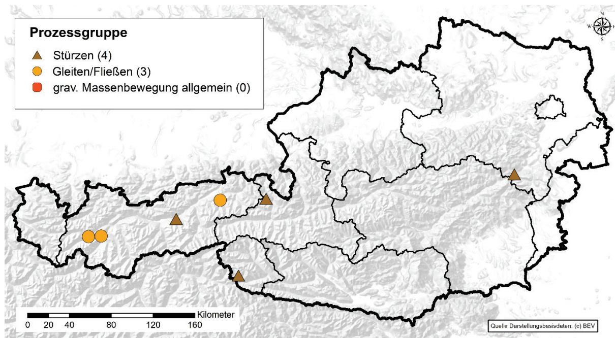
Abb. 3: Räumliche Verteilung der für Jänner 2024 mittels Recherchen in Online-Medien erfassten gravitativen Massenbewegungen unterschiedlicher Prozessgruppen (in Klammern die jeweilige Gesamtanzahl).
