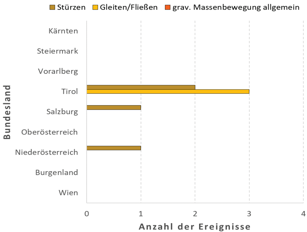
Abb. 2: Mittels Recherchen in Online-Medien für Jänner 2024 erfasste gravitative Massenbewegungen, differenziert nach Bundesländern und Prozessgruppen.
