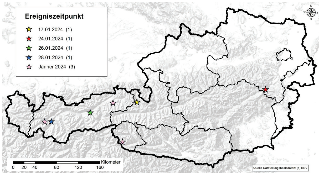
Abb. 5: Räumliche und zeitliche Verteilung der mittels Recherchen in Online-Medien erfassten gravitativen Massenbewegungen in Österreich im Jänner 2024 (in Klammern die Anzahl der Ereignisse).
