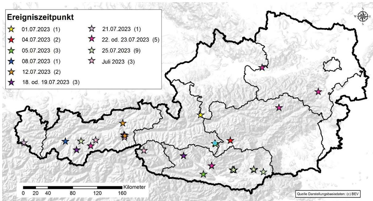
Abb. 6: Räumliche und zeitliche Verteilung der mittels Recherchen in Online-Medien erfassten gravitativen Massenbewegungen in Österreich im Juli 2023 (in Klammern die Anzahl der Ereignisse) (Anmerkung: Die Anzahl der Ereignisse wird vom gewählten Maßstab nicht korrekt wiedergegeben).
