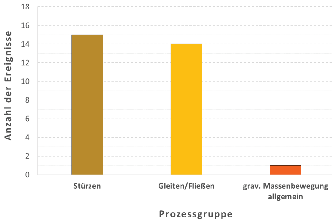
Abb. 1: Mittels Recherchen in Online-Medien erfasste gravitative Massenbewegungen im Juli 2023, differenziert nach Prozessgruppen.
