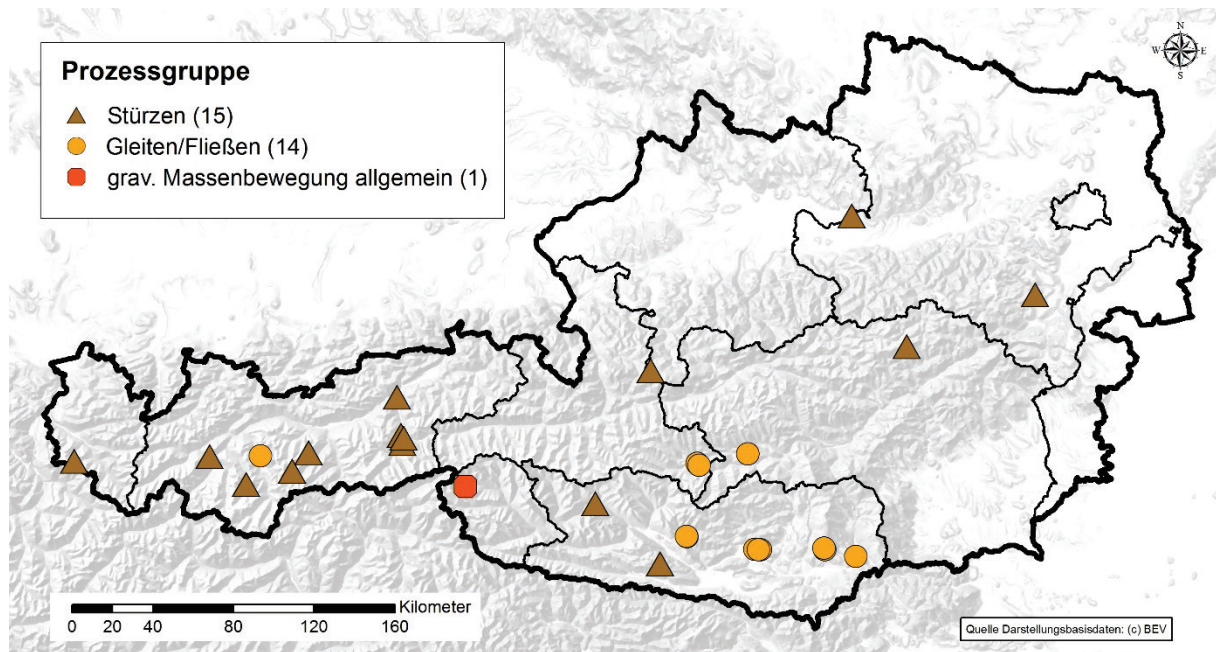
Abb. 3: Räumliche Verteilung der für Juli 2023 mittels Recherchen in Online-Medien erfassten gravitativen Massenbewegungen unterschiedlicher Prozessgruppen (in Klammern die jeweilige Gesamtanzahl) (Anmerkung: Die Anzahl der Ereignisse wird vom gewählten Maßstab nicht korrekt wiedergegeben).
