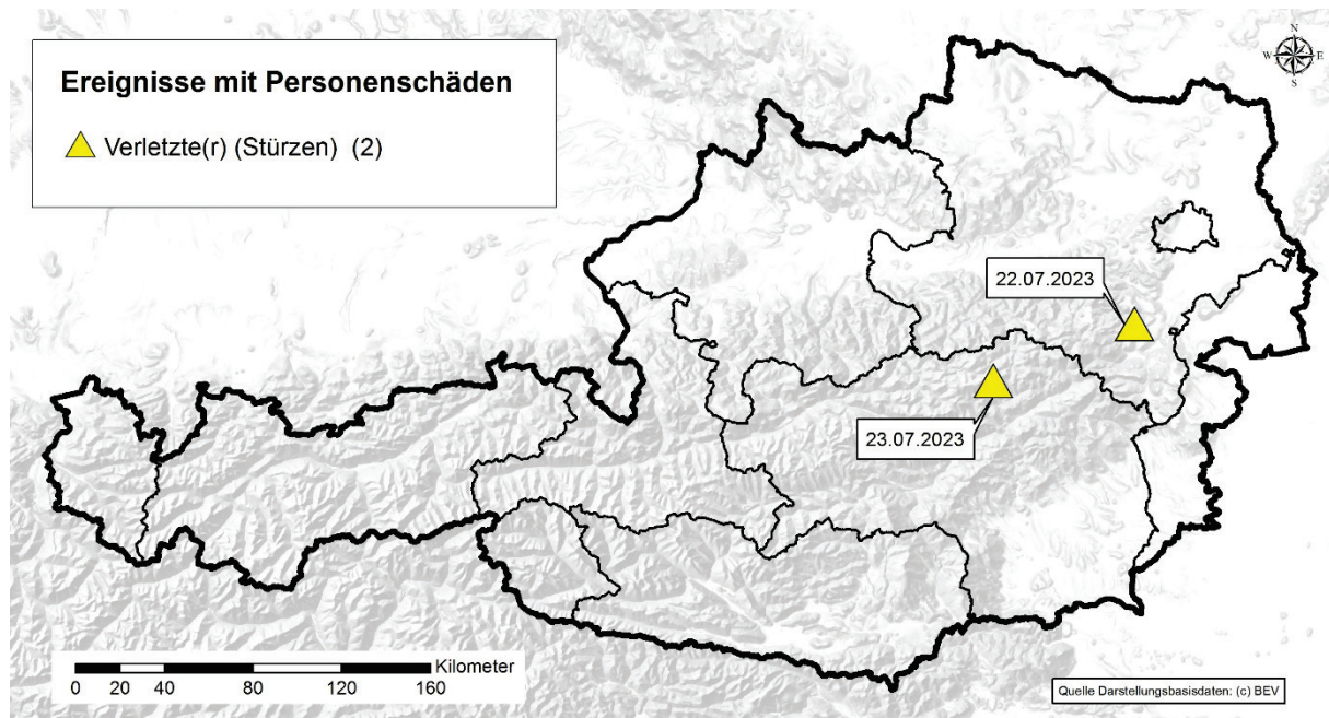
Abb. 4: Räumliche Verteilung der mittels Recherchen in Online-Medien im Juli 2023 erfassten gravitativen Massenbewegungen mit Toten oder Verletzten, differenziert nach Prozessgruppen (in Klammern die jeweilige Anzahl der Ereignisse).
