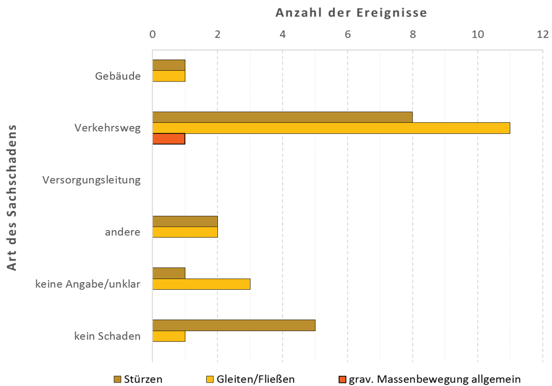
Abb. 5: Überblick zu den mit gravitativen Massenbewegungen im Juli 2023 einhergegangenen Arten von Sachschäden (Achtung: Mehrfachnennungen möglich, weil bei einem Ereignis mehrere Sachschadensarten auftreten können!). Datenbasis: Recherchen der GeoSphere Austria) in Online-Medien.
