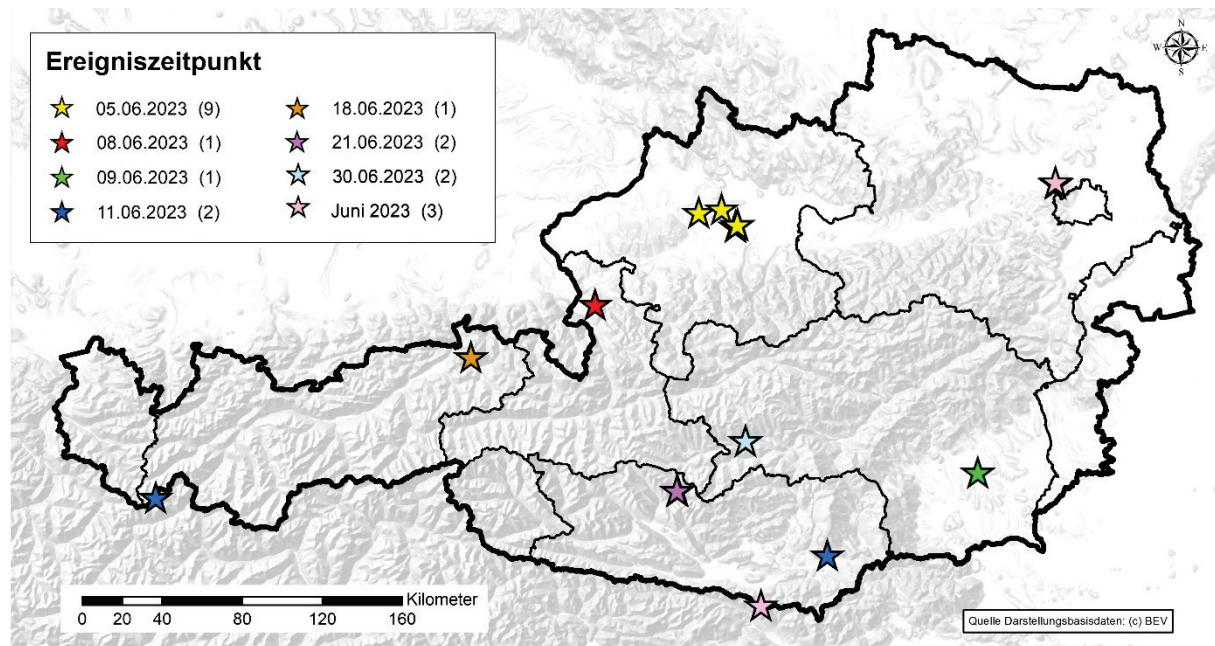
Abb. 6: Räumliche und zeitliche Verteilung der mittels Recherchen in Online-Medien erfassten gravitativen Massenbewegungen in Österreich im Juni 2023 (in Klammern die Anzahl der Ereignisse). Zehn Ereignisse konnten keinem genauen Datum zugeordnet werden (Anmerkung: Die Anzahl der Ereignisse wird vom gewählten Maßstab nicht korrekt wiedergegeben).
