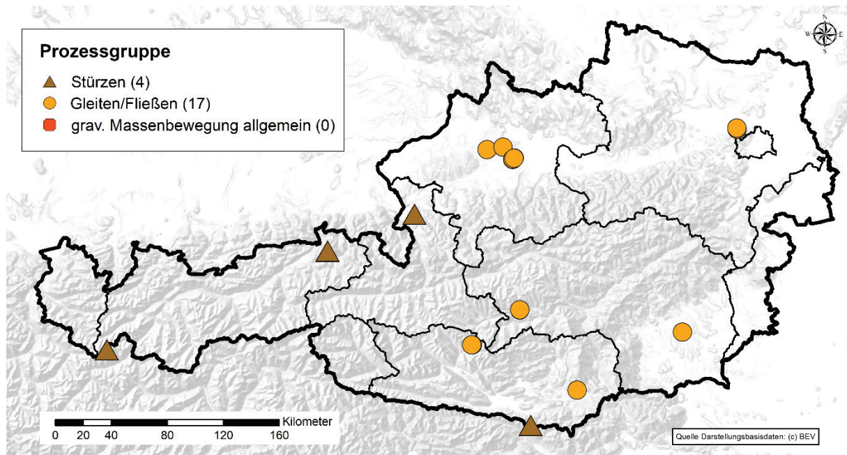
Abb. 3: Räumliche Verteilung der für Juni 2023 mittels Recherchen in Online-Medien erfassten gravitativen Massenbewegungen unterschiedlicher Prozessgruppen (in Klammern die jeweilige Gesamtanzahl) (Anmerkung: Die Anzahl der Ereignisse wird vom gewählten Maßstab nicht korrekt wiedergegeben).
