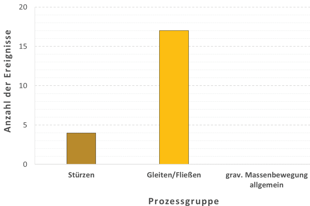
Abb. 1: Mittels Recherchen in Online-Medien erfasste gravitative Massenbewegungen im Juni 2023, differenziert nach Prozessgruppen.
