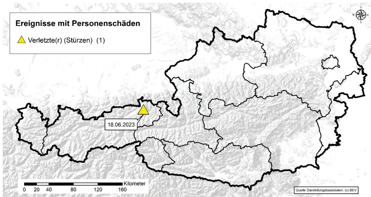
Abb. 4: Räumliche Verteilung der mittels Recherchen in Online-Medien im Juni 2023 erfassten gravitativen Massenbewegungen mit Toten oder Verletzten, differenziert nach Prozessgruppen (in Klammern die jeweilige Anzahl der Ereignisse).
