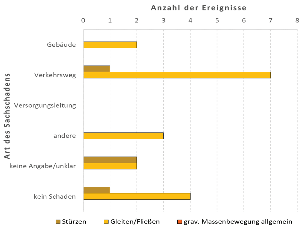
Abb. 5: Überblick zu den mit gravitativen Massenbewegungen im Juni 2023 einhergegangenen Arten von Sachschäden (Achtung: Mehrfachnennungen möglich, weil bei einem Ereignis mehrere Sachschadensarten auftreten können!). Datenbasis: Recherchen der GeoSphere Austria) in Online-Medien.
