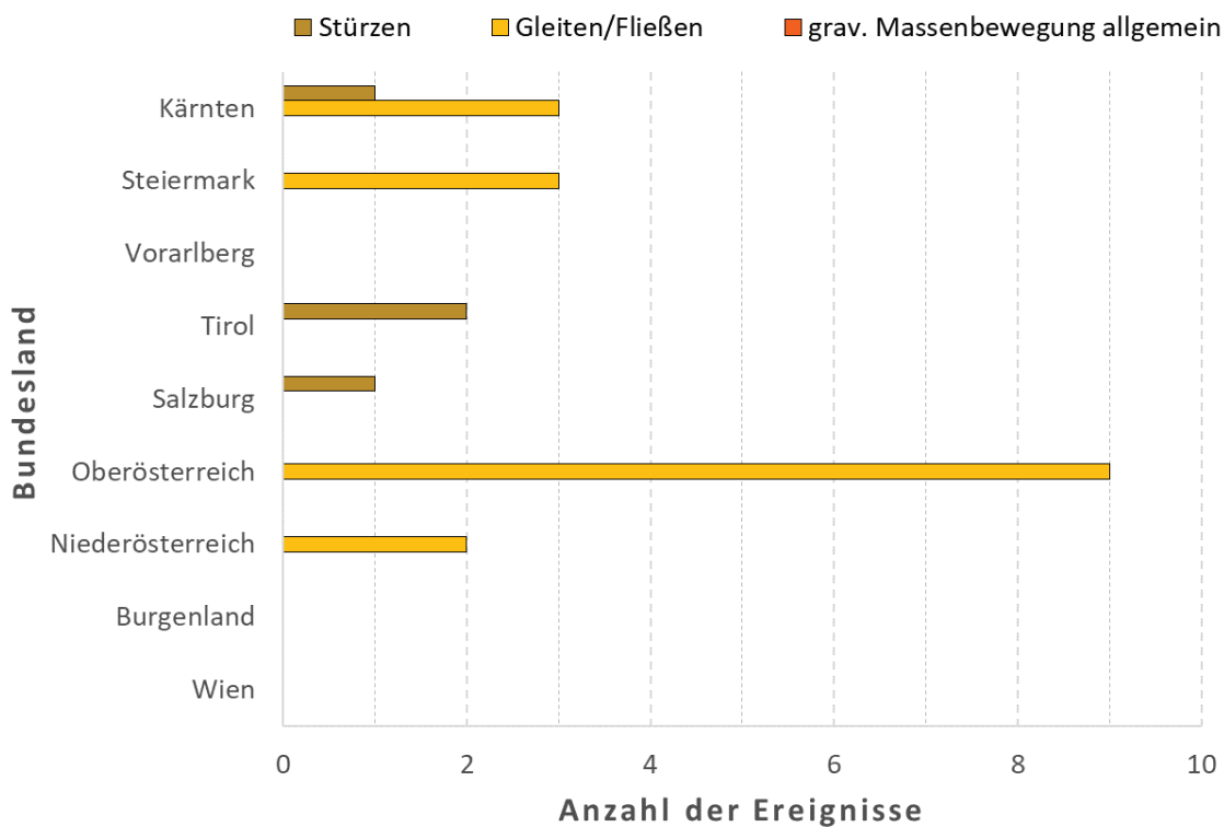
Abb. 2: Mittels Recherchen in Online-Medien für Juni 2023 erfasste gravitative Massenbewegungen, differenziert nach Bundesländern und Prozessgruppen.
