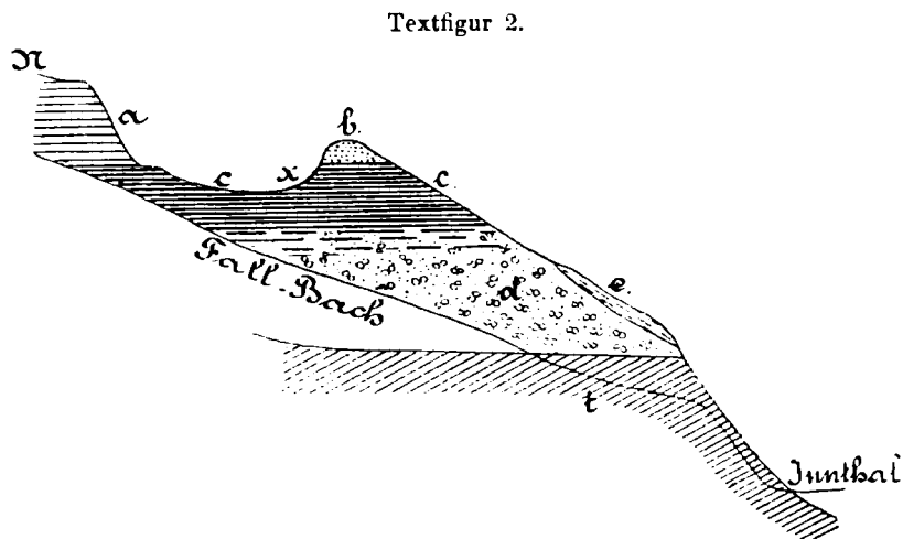
a Glaciale Schotter; b rothe Breccie; c geschichteter vielfach verworfener Tegel und x der Punkt, an welchem in der Tegelgrube Pflanzenreste gefunden wurden; d Grund-Moräne mit gekritzten Geschieben; e Schutzkegel-Conglomerat, die Breccien spärlich führend; t Trias-Dolomit.
