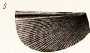
H. lobata
