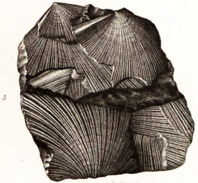
H. lobata
