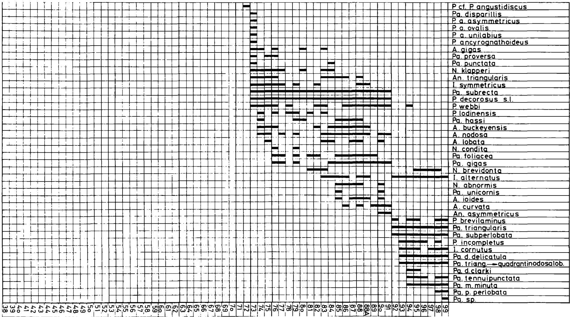
Abb. 24: Profil „Wolayer Glieder“ - Verteilung von Conodonten im Mittel- und Oberdevon (Valentin-Kalk und Pal-Kalk; nach B. GODDERTZ, 1982).
