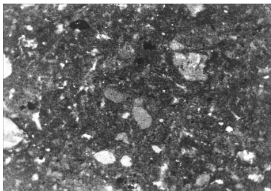
Abb. 5. Roter Bauxit im Durchlicht. Dunkle Bereiche stärker, helle Bereiche weniger mit Fe-Mineralen pigmentiert. Sedimentierte knöllchenförmige Komponenten verschiedener mineralischer Zusammensetzung. Bildausschnitt 1,44 × 0,94 mm. 1 Nicol.
