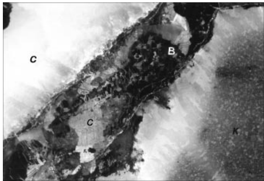
Abb. 12. Schwach Bauxit-pigmentierter feinkristalliner Gosau-Kalkstein (rechts, K) im Liegenden des Bauxitlagers rupturrell beschädigt und mit mechanisch eingeschwemmtem Bauxit (dunkelgrau, B) und späti-gem Calcitkristallinat (C) in zwei Deformations- und zwei Kristallisationsphasen zementiert. Schwache Zerschering der gesamten Fugenfüllung. Auflicht, polierter Anschliff, + Nicols. Bildausschnitt 0,93 × 0,66 mm.
