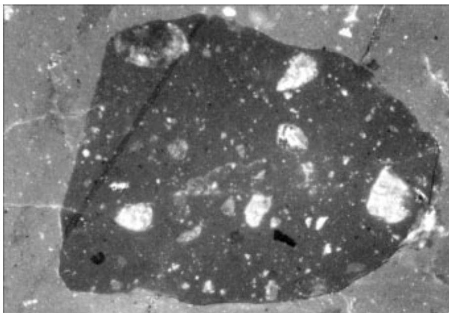
Abb. 9. Bauxit in Bauxit: Resedimentierte, bereits polymikt zusammengesetzte Bauxitkomponente mit Hämatit, Lepidokrokit, Goethit und Rutil im helleren, weniger pigmentierten Bauxit. Polierter Anschliff. x Nicols. Bildausschnitt 3,73 × 2,65 mm.
