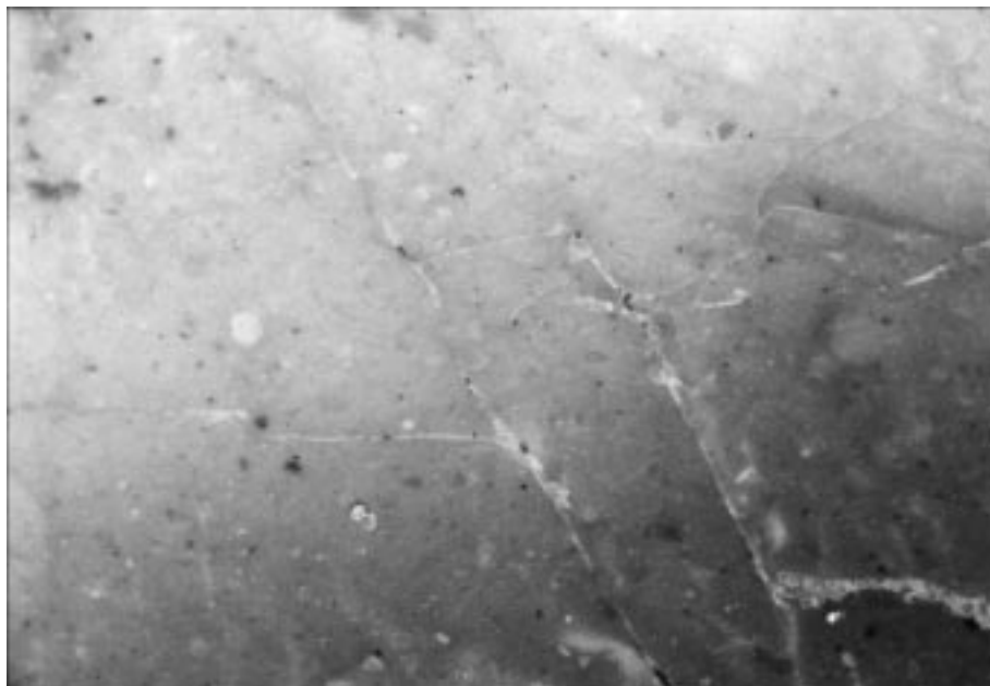
Abb. 8. Übergang vom rot pigmentierten (im Bild grau) zum nicht pigmentierten Bauxit (grauweiß) im polierten Anschliff bei + Nicols. Bildausschnitt 3,73 × 2,65 mm.
