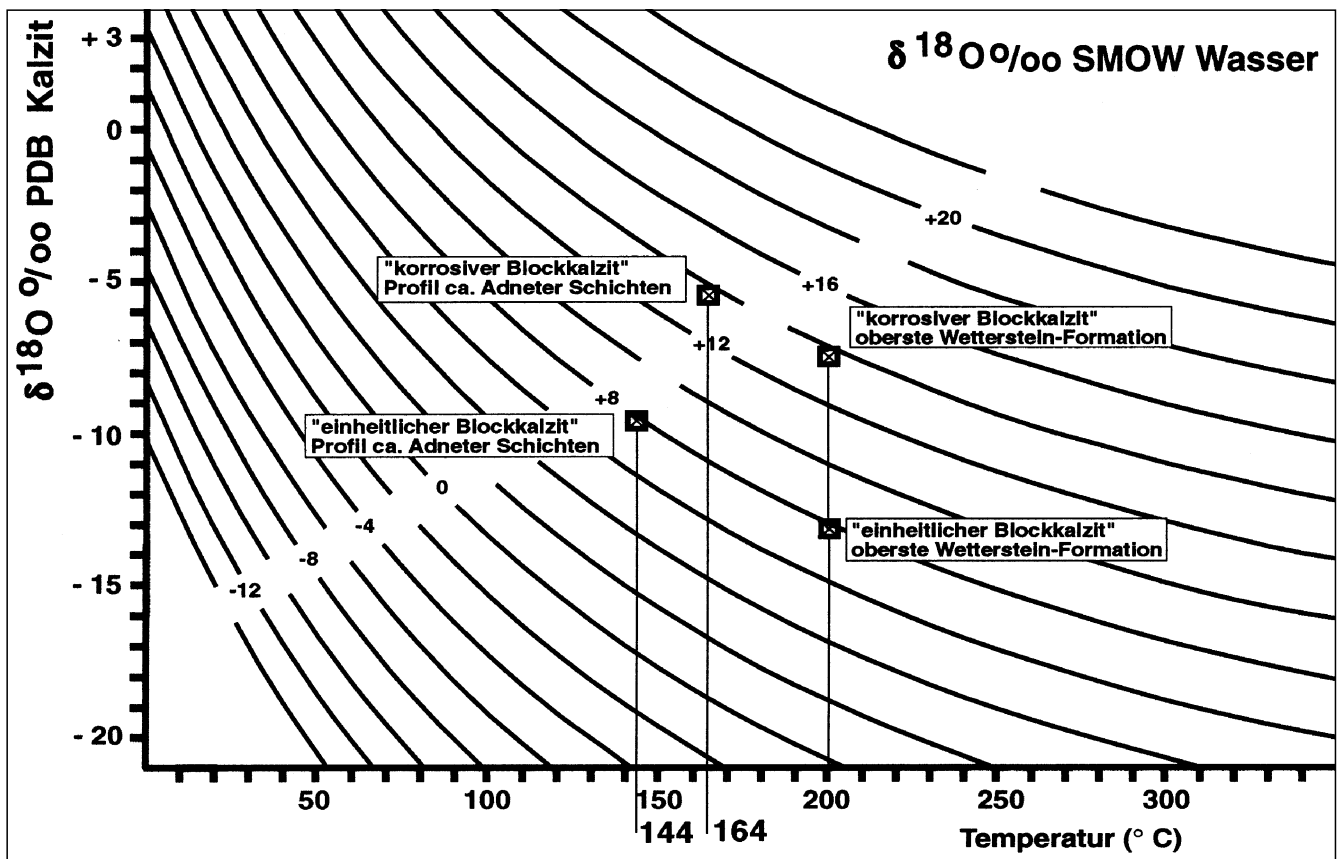
Abb. 13. Verschiebung der durchschnittlichen Sauerstoffisotopenverhältnisse von der obersten Wetterstein-Formation zum Profil Rhät bis Unter-Kreide (ca. 500 m Mächtigkeit, Mitte des Profils entspricht ca. den Adneter Schichten; vgl. Abb. 10). Die Isolinien der Formationswasserzusammensetzung ergeben sich aus den Gleichungen (1) und (2). Die durchschnittliche Bildungstemperatur der Zemente im Profilabschnitt Rhät bis Unter-Kreide wurde unter Annahme konstanter Isotopenzusammensetzung des Formationswassers aus dem verschobenen Isotopenwert abgeleitet.
