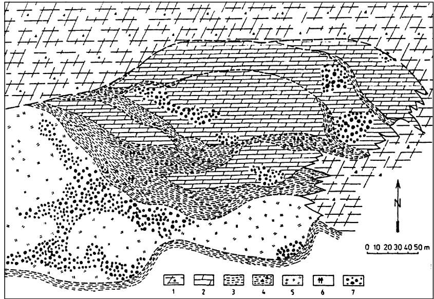
Abb. 20. Vererzung von Riffdolomit und Dolomit benachbarter lagunärer Fazies im Revier Graben/Mezica (aus STRUCL, 1984). 1 = bituminöser Dolomit; 2 = lagunärer vererzter Dolomit; 3 = Tonstein; 4 = tonig-dolomitische Brekzie; 5. dolomitierter Riffkalk; 6 = Gips und Anhydrit; 7 = Pb-Zn-Mineralisation.
