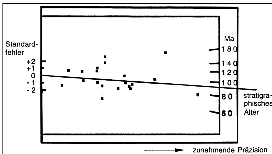
Abb. 14. Apatit-Spaltspurenalter einer mittelkretazischen Flyschprobe von der Gornja.
