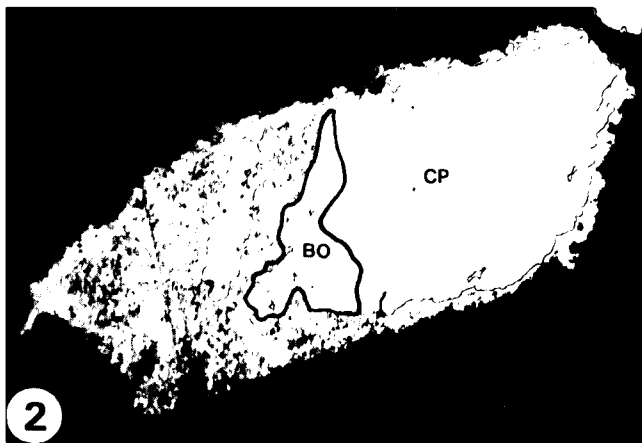
Abb. 2. In Quarz eingebettetes Chalkopyrit-Korn (CP) zeigt Verdrängung durch Bornit (BO) und nachfolgend solche von Anilit (an). Bildbreite = 100 \mu\text{m} .
