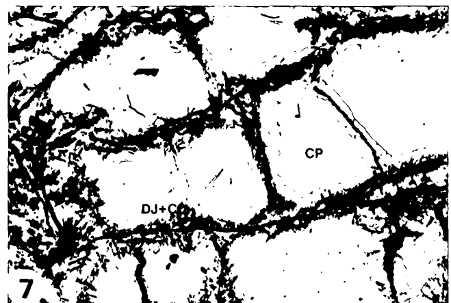
Abb. 7. Chalkopyrit mit zementativer Verdrängung durch Djurleit und (rhomb.) Chalkosin (CC). Saumbreite = 40–60 \mu m .
