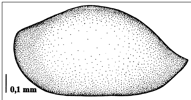
Abb. 128. Bairdia (Rectobairdia) cf. hisingeri (MÜNSTER 1830). Seiten-Ansicht einer linken Klappe (Latex-Abguß) nach dem Exemplar T15 S 0072 (vgl. Taf. 11, Fig. 12). Unter-Karbon (Oberes Viseum), Nötsch-Formation (sensu SCHÖNLAUB, 1985). Fundpunkt SCHÖNLAUB 1, Region Oberhöher bei Nötsch, Kärnten.
