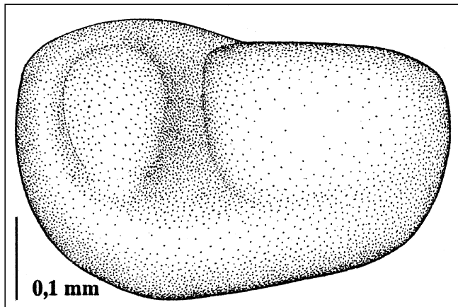
Abb. 93. Knoxiella ? cf. infera BAUSCHMINA 1965. Seiten-Ansicht einer linken Klappe (Steinkern) nach dem Exemplar T31 S03189 (vgl. Taf. 7, Fig. 16). Unter-Karbon (Oberes Viseum), Nötsch-Formation (sensu SCHÖNLAUB, 1985). Fundpunkt SCHÖNLAUB 1, Region Oberhöher bei Nötsch, Kärnten.
