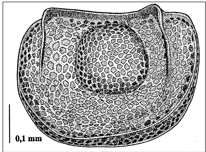
Abb. 70. Amphissites (Amphissites) centronotus (ULRICH & BASSLER 1906). Seiten-Ansicht einer linken Klappe (Latex-Abguß) nach dem Exemplar T19 S02993 (vgl. Taf. 7, Fig. 4). Bereich der hinteren Ecke ergänzt. Unter-Karbon (Oberes Viseum), Nötsch-Formation (sensu SCHÖNLAUB, 1985). Fundpunkt SCHÖNLAUB 1, Region Oberhöher bei Nötsch, Kärnten.
