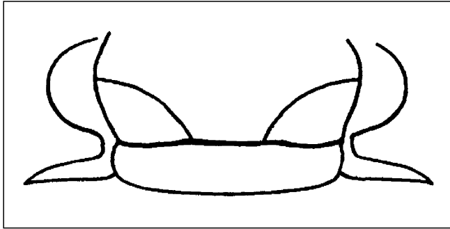
Abb. 31. Paladin (Paladin) laticapitatus n. sp. Medianes Hinterende der Glabella breit, eine gerade Linie bildend.
