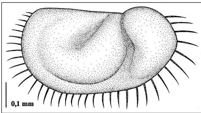
Abb. 97. Pseudobeyrichiopsis longispinosa n. sp. Seiten-Ansicht einer linken Klappe, weibliches Tier (Steinkern) nach dem Paratypus T29 S03176 (vgl. Taf. 8, Fig. 6). Stacheln am Vorder- und Hinterrand ergänzt. Unter-Karbon (Oberes Viseum), Nötsch-Formation (sensu SCHÖNLAUB, 1985). Fundpunkt SCHÖNLAUB 1, Region Oberhöher bei Nötsch, Kärnten.
