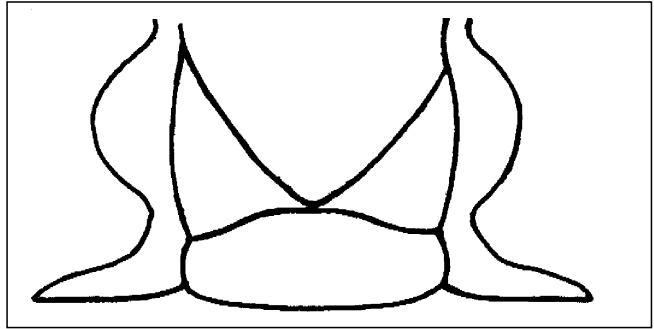
Abb. 32) Paladin (Paladin) eichwaldi . Medianes Hinterende der Glabella schmal, Abgerundet „zugespitzt“.
