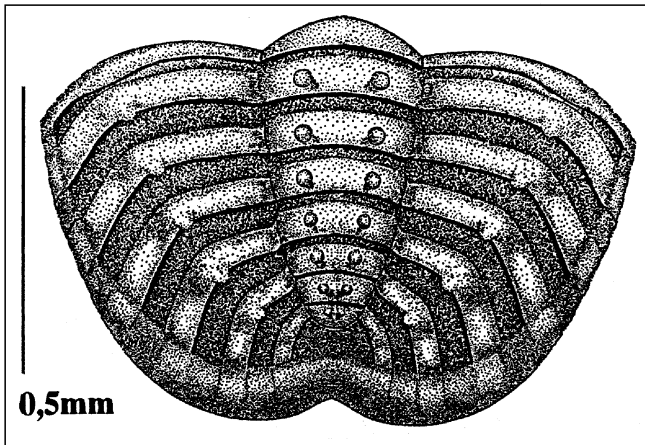
Abb. 12. Sehr junges Meraspis-Stadium (nach S 1 1992/03, Latex-Abguß), Dorsal-Ansicht (ca. 0,7 mm, vgl. Taf. 2, Fig. 8). Unter-Karbon (Oberes Viseum), Nötsch-Formation (sensu SCHÖNLAUB, 1985). Fundpunkt SCHÖNLAUB 1, Oberhöher bei Nötsch, Kärnten.
