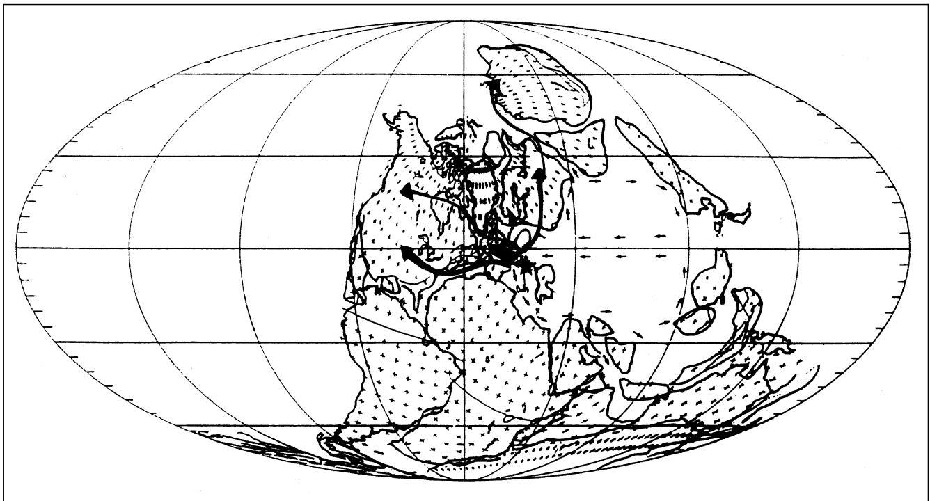
Abb. 138. Zusammenfassende Darstellung der paläobiogeographischen Beziehungen der Ostracoden von Nötsch in Kärnten während des Unter-Karbons (Visium). Der Stern zeigt die damalige ungefähre Lage des Arbeitsgebietes, die Dicke der Pfeile ungefähr die prozentualen Anteile der Verbreitungsrichtung an; kurze, kleine Pfeile = Äquatoriales Strömungssystem (verändert nach SCHÖNLAUB, 1992: Abb. 15).
