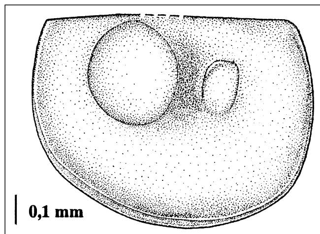
Abb. 58. Hollinella (Hollinella) cf. ulrichi (KNIGHT 1928). Seiten-Ansicht einer rechten Klappe (Steinkern, ? juvenile Form) nach dem Exemplar T13 01459 (vgl. Taf. 5, Fig. 13). Die Verdrückung am Dorsalrand wurde entzerrt. Unter-Karbon (Oberes Viseum), Nötsch-Formation (sensu SCHÖNLAUB 1985). Fundpunkt KODSI 1, Region Oberhöher bei Nötsch, Kärnten.
