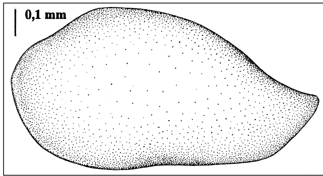
Abb. 130. Bairdia (Rectobairdia) sp. aff. B. fragosa MOREY 1935. Seiten-Ansicht einer linken Klappe (Steinkern) nach dem Exemplar T28 S03169 (vgl. Taf. 11, Fig. 14). Unter-Karbon (Oberes Viseum), Nötsch-Formation (sensu SCHÖNLAUB, 1985). Fundpunkt SCHÖNLAUB 1, Region Oberhöher bei Nötsch, Kärnten.
