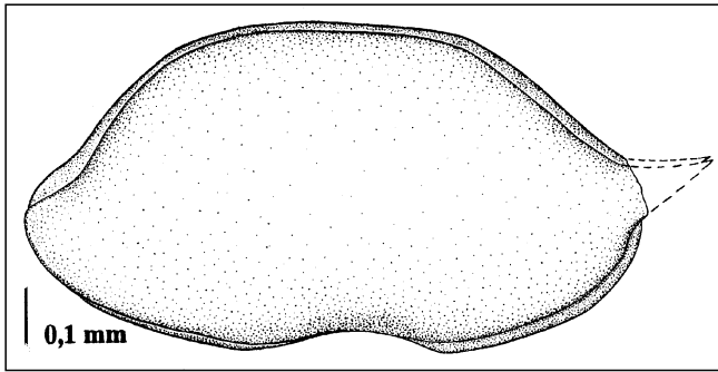
Abb. 123. Bairdia (Rectobairdia) kirinae ZANINA 1956. Seiten-Ansicht einer rechten Klappe (Latex-Abguß) nach dem Exemplar T2 S1367 (vgl. Taf. 11, Fig. 7). Stachel am Vorderende rekonstruiert. Unter-Karbon (Oberes Viseum), Nötsch-Formation (sensu SCHÖNLAUB, 1985). Fundpunkt SCHÖNLAUB 1, Region Oberhöher bei Nötsch, Kärnten.
