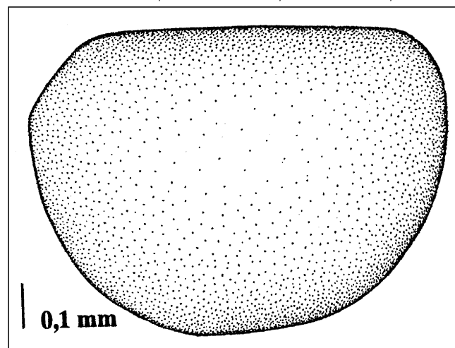
Abb. 84. Shemonaella cf. opima (KOTSCHETKOVA 1983). Seiten-Ansicht einer linken Klappe (Steinkern) nach dem Exemplar T26 S0315 (vgl. Taf. 9, Fig. 1). Hintere Ecke ergänzt. Unter-Karbon (Oberes Viseum), Nötsch-Formation (sensu SCHÖNLAUB, 1985). Fundpunkt SCHÖNLAUB 1, Region Oberhöher bei Nötsch, Kärnten.
