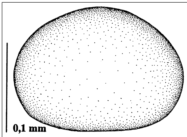
Abb. 104. Praepilatina? sp. Seiten-Ansicht einer linken Klappe (Latex-Abguß) nach dem Exemplar T06 K1457 (vgl. Taf. 10, Fig. 4). Unter-Karbon (Oberes Viseum), Nötsch-Formation (sensu SCHÖNLAUB, 1985). Fundpunkt KODSI 1, Region Oberhöher bei Nötsch, Kärnten.
