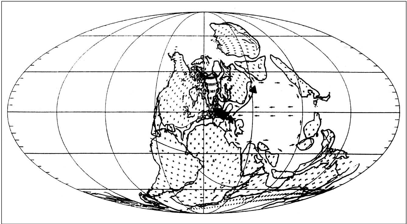
Abb. 137. Zusammenfassende Darstellung der paläobiogeographischen Beziehungen der Trilobiten von Nötsch in Kärnten während des Unter-Karbons (Visium). Der Stern zeigt die damalige ungefähre Lage des Arbeitsgebietes, die Dicke der Pfeile ungefähr die prozentualen Anteile der Verbreitungsrichtung an; kurze, kleine Pfeile = Äquatoriales Strömungssystem (verändert nach SCHÖNLAUB, 1992: Abb. 15).
