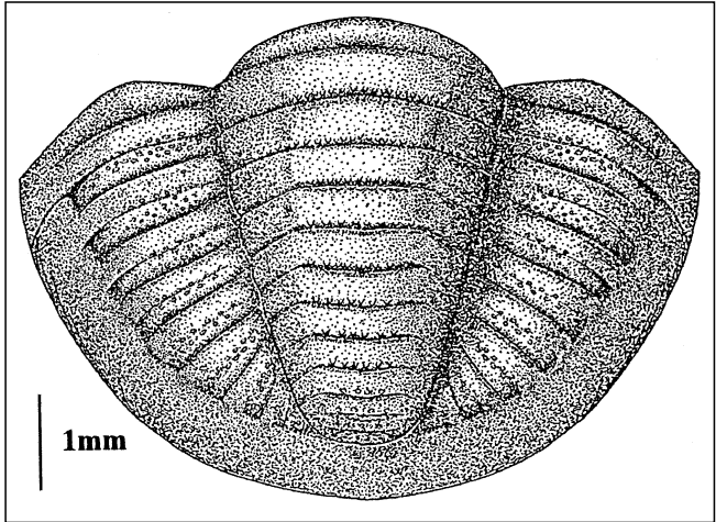
Abb. 51. Dorsal-Ansicht eines normal gebauten, gesunden Pygidiums (nach dem Exemplar S 1 1990/06; vgl. Taf. 2, Fig. 16a). Unter-Karbon (Oberes Viseum), Nötsch-Formation (sensu SCHÖNLAUB, 1985). Fundpunkt SCHÖNLAUB 1, Raum Oberhöher bei Nötsch, Kärnten.
