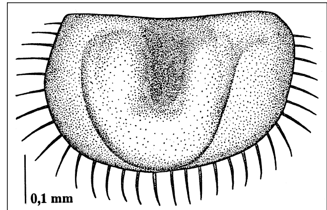
Abb. 95. Pseudobeyrichiopsis spinosa KOZUR 1985. Seiten-Ansicht einer linken Klappe (Steinkern, männliches Tier) nach dem Exemplar T28 S03170 (vgl. Taf. 8, Fig. 3). Die meisten Stacheln am gesamten freien Rand ergänzt. Unter-Karbon (Oberes Viseum), Nötsch-Formation (sensu SCHÖNLAUB, 1985). Fundpunkt SCHÖNLAUB 1, Region Oberhöher bei Nötsch, Kärnten.
