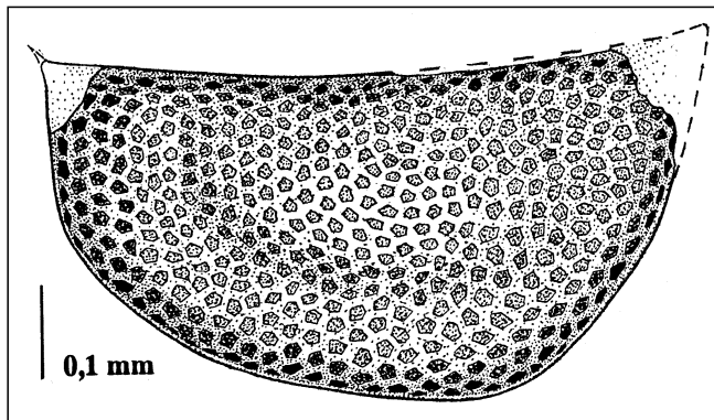
Abb. 69. Coronakirkbya ? n. sp. A. Seiten-Ansicht einer rechten Klappe (Latex-Abguß) nach dem Exemplar T4 S1112 (vgl. Taf. 7, Fig. 3). Vordere und hintere Ecke ergänzt. Unter-Karbon (Oberes Viseum), Nötsch-Formation (sensu SCHÖNLAUB, 1985). Fundpunkt SCHÖNLAUB 1, Region Oberhöher bei Nötsch, Kärnten.
