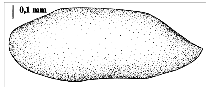
Abb. 131. Bairdia (Rectobairdia) sp. A. Seiten-Ansicht einer linken Klappe (Schalen-Exemplar) nach dem Exemplar T14 S0042 (vgl. Taf. 11, Fig. 15). Bereich des Hinterendes ergänzt. Unter-Karbon (Oberes Viseum), Nötsch-Formation (sensu SCHÖNLAUB, 1985). Fundpunkt SCHÖNLAUB 1, Region Oberhöher bei Nötsch, Kärnten.
