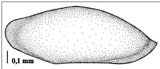
Abb. 120. Bairdia (Bairdia) n. sp. sensu BRADFIELD 1935. Seiten-Ansicht einer linken Klappe (Latex-Abguß) nach dem Exemplar T2 S1153 (vgl. Taf. 11, Fig. 3-4). Unter-Karbon (Oberes Viseum), Nötsch-Formation (sensu SCHÖNLAUB, 1985). Fundpunkt SCHÖNLAUB 1, Region Oberhöher bei Nötsch, Kärnten.
