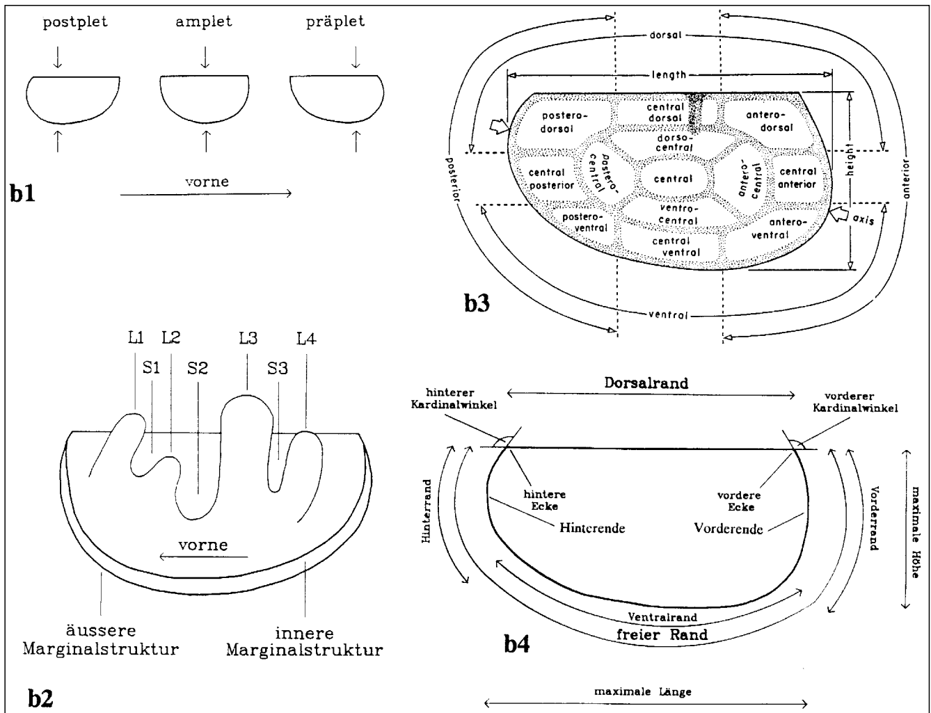
Abb. 52. Morphologie und Terminologie bei einem Ostracoden-Carapax (Seiten-Ansicht). Umriß-Grundtypen bei den Palaeocopida (b1).
