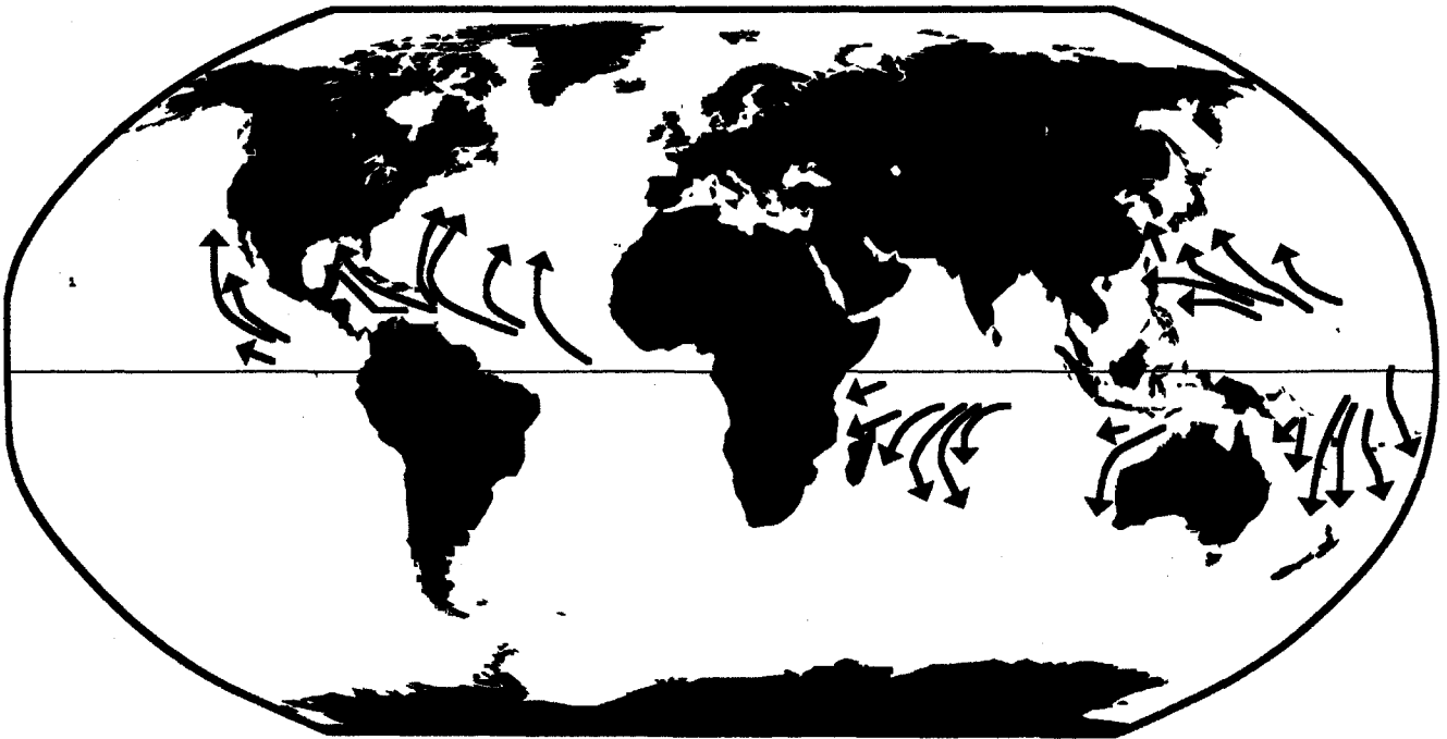
Abb. 7. Weltkarte mit den wichtigsten Hurrikan-Gebieten (nach KRÜGER, 1979). Bei Vergleich mit Abb. 3 fällt das weitgehende Zusammenfallen von Rifffgebieten und Hurrikangebieten auf.
