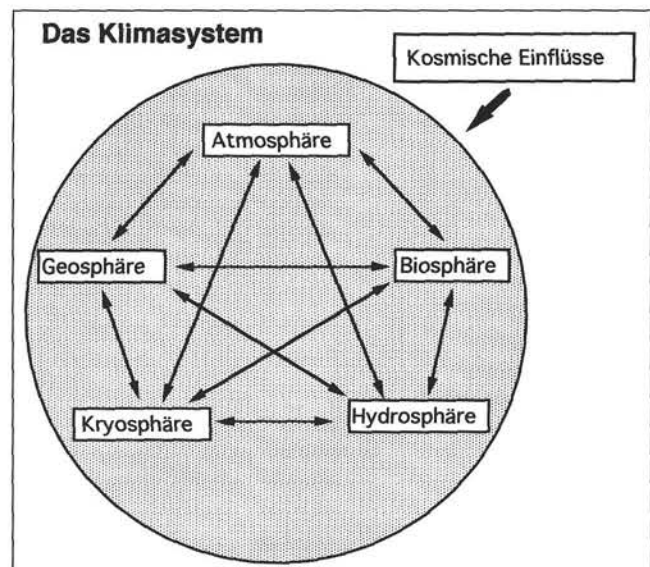
Abb. 2. Unter Klimasystem wird heute das komplexe Wechselwirkungsgefüge der hier dargestellten Komponenten verstanden.
