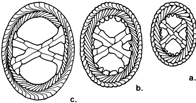
Fig. 13 a) Neochiastozygus modestus , early form. b) Neochiastozygus modestus , late form. c) Neochiastozygus perfectus .
