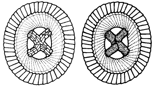
Fig. 7: Chiasmolithus inconspicuus n. sp.
