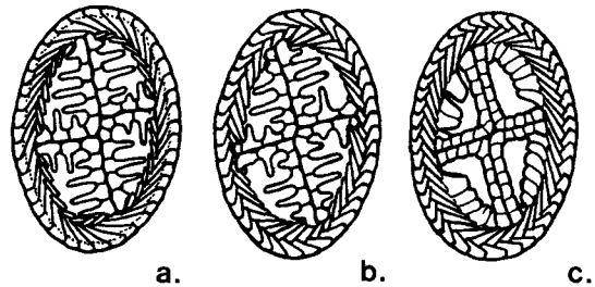
Fig. 15: “Asymmetrical species” a) Chiastozygus ultimus . b) Neochiastozygus primitivus . c) Neochiastozygus denticulatus .
