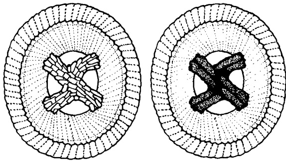
Fig. 5: Chiasmolithus edentulus n. sp.
