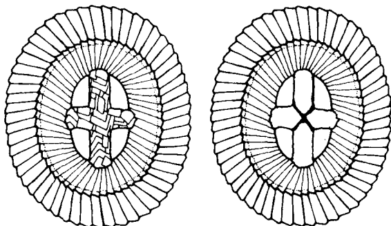
Fig. 9: Cruciplacolithus intermedius n. sp.
